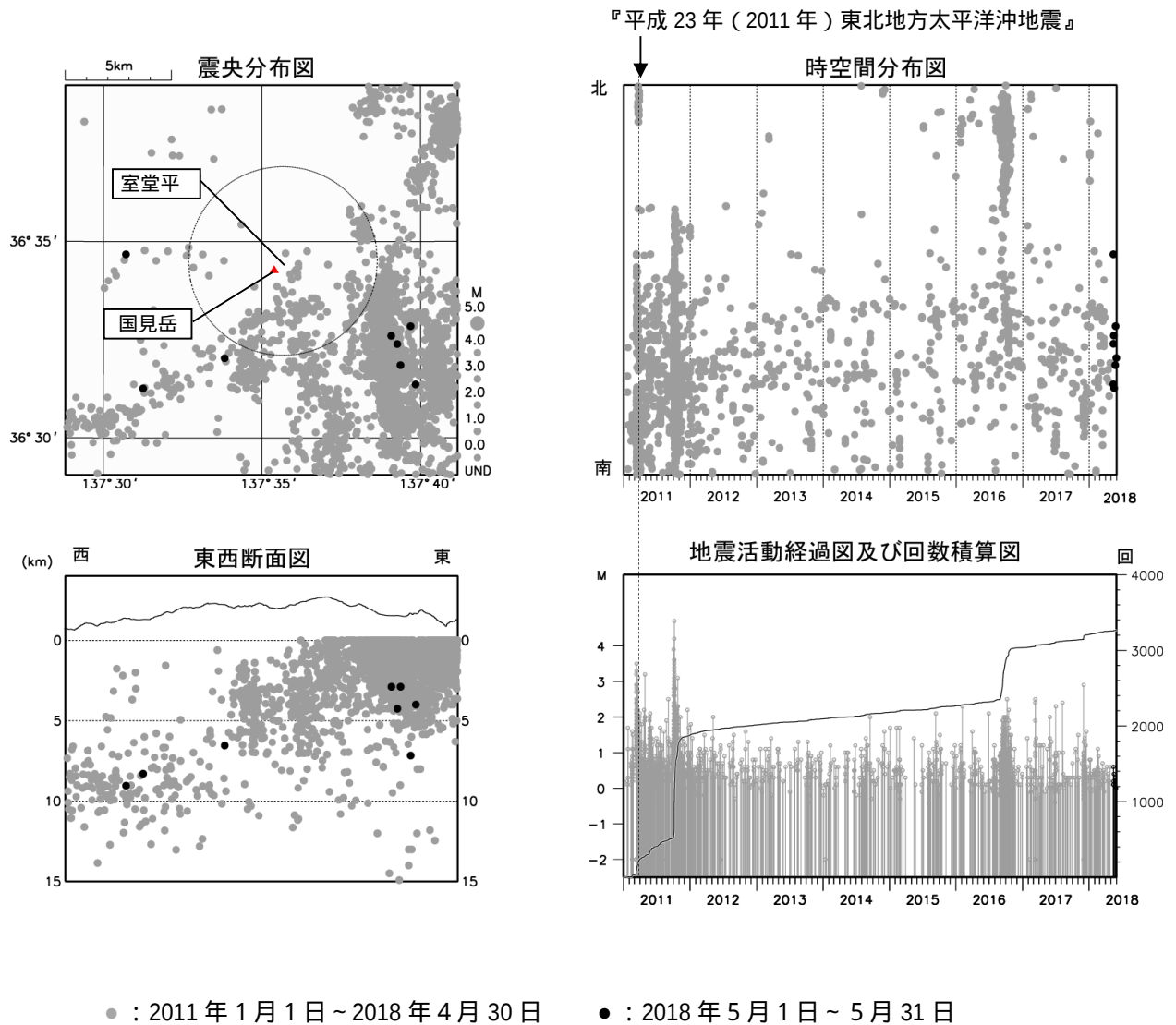
図 2 弥陀ヶ原 広域地震観測網による山体・周辺の地震活動（2011 年 1 月 1 日～2018 年 5 月 31 日）
