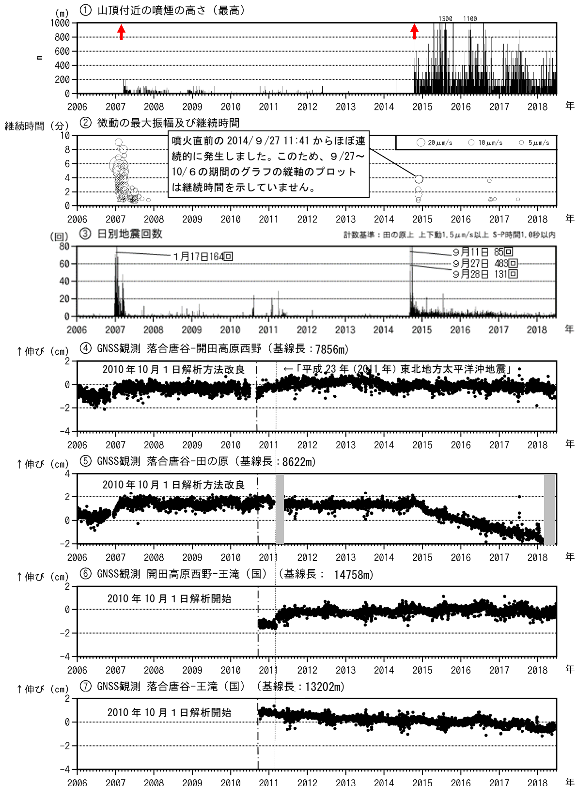
図4 御嶽山 長期間の火山活動経過図（2006年1月1日～2018年6月30日）
