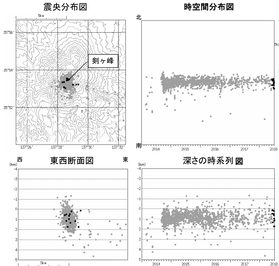
図 2 御嶽山 震源分布図（2014 年 1 月 1 日～2018 年 6 月 30 日）
