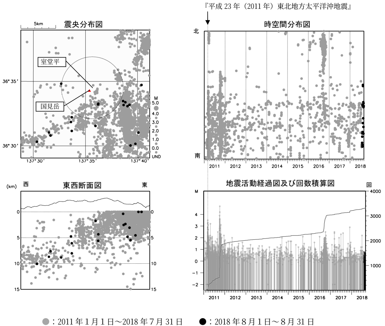
図 2 弥陀ヶ原 広域地震観測網による山体・周辺の地震活動（2011 年 1 月 1 日～2018 年 8 月 31 日）
