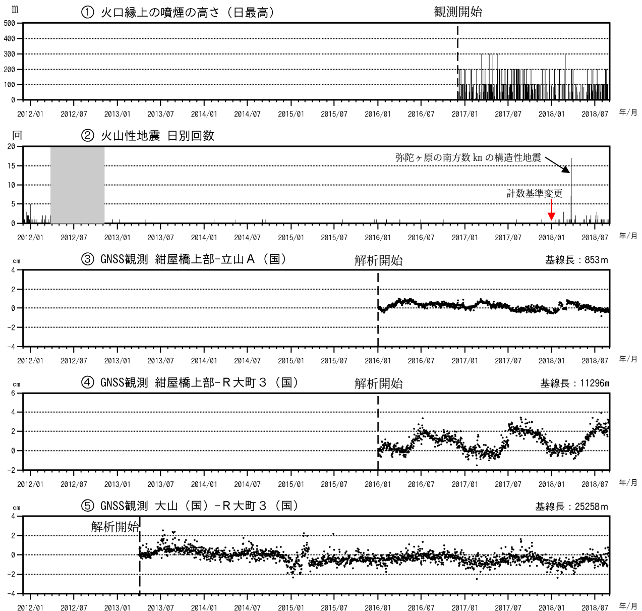
図3 弥陀ヶ原 火山活動経過図（2011 年 12 月 1 日～2018 年 8 月 31 日）
