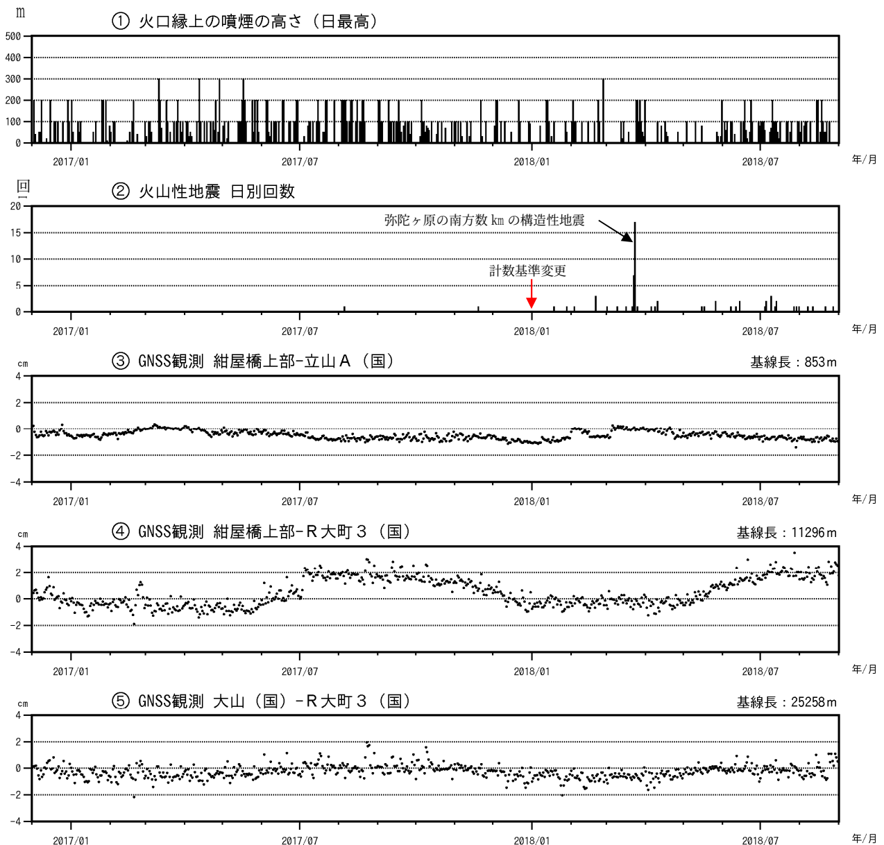
図4 弥陀ヶ原 最近の火山活動経過図（2016 年 12 月 1 日～2018 年 8 月 31 日）
