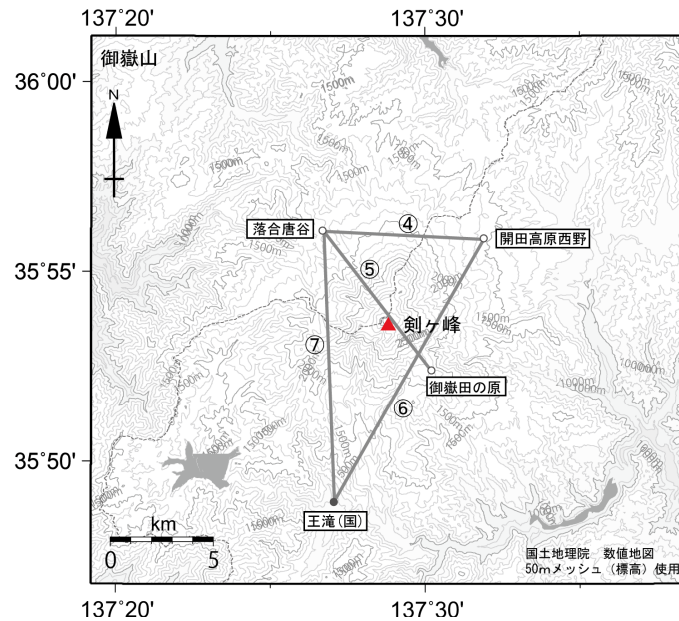
図 7 御嶽山 GNSS 連続観測点と基線番号
