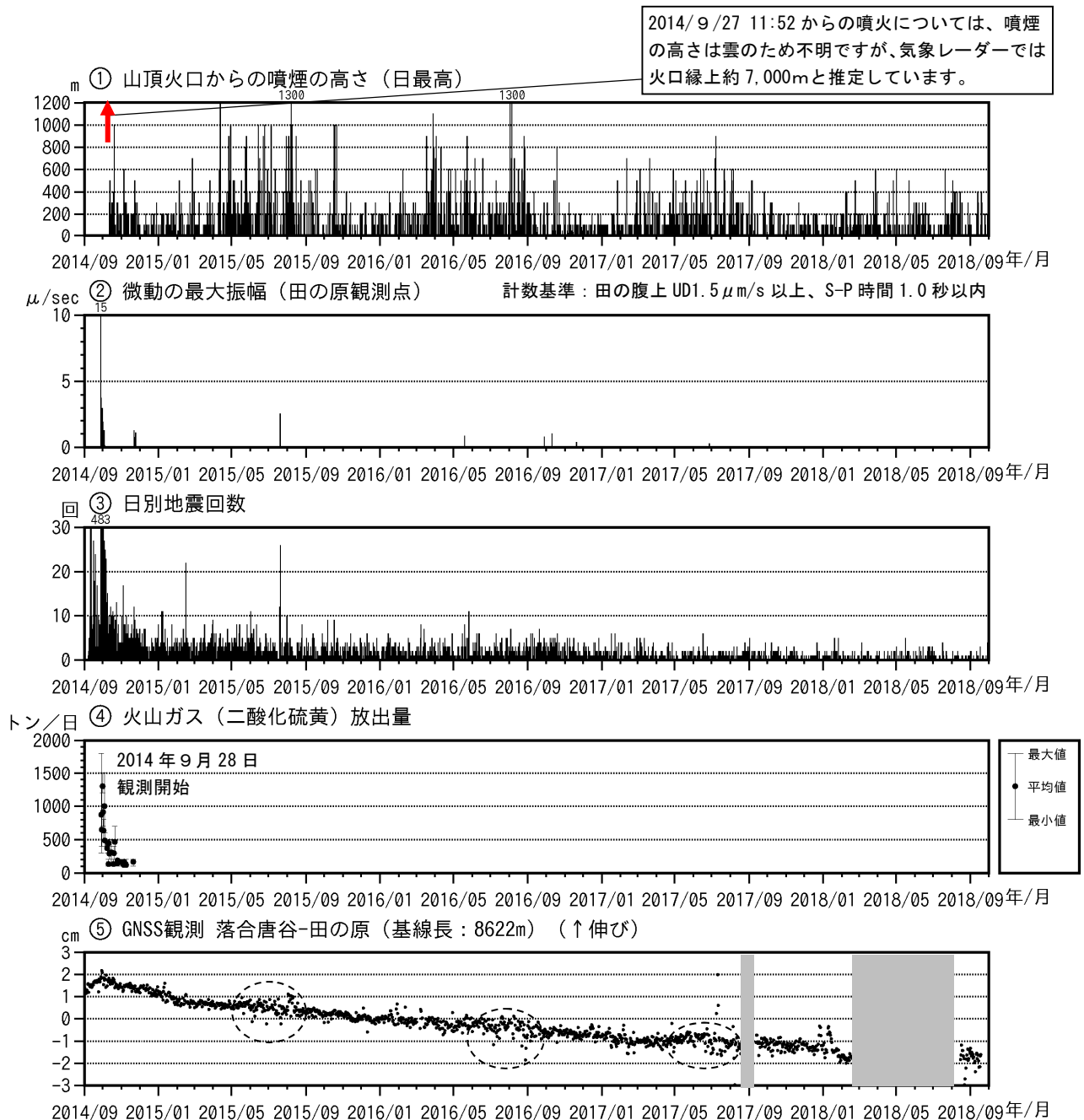
図3 御嶽山 最近の火山活動経過図（2014年9月1日～2018年9月30日）
