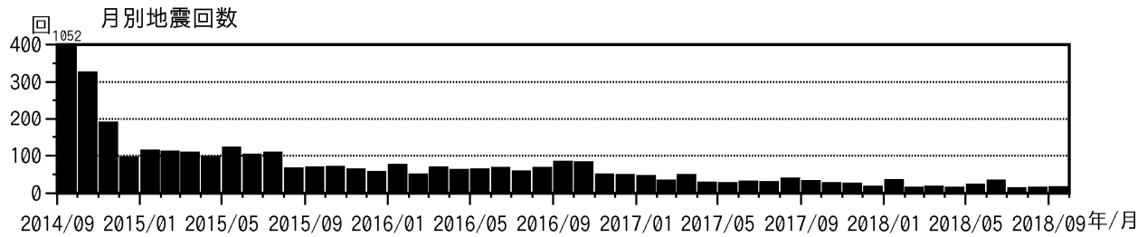
図 4 御嶽山 月別地震回数経過図（2014 年 9 月 1 日～2018 年 9 月 30 日）
