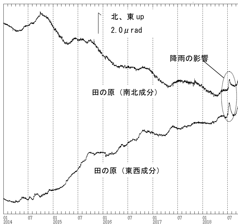
図 8 御嶽山 田の原観測点の傾斜変動（2014 年 1 月 1 日～2018 年 9 月 30 日）
