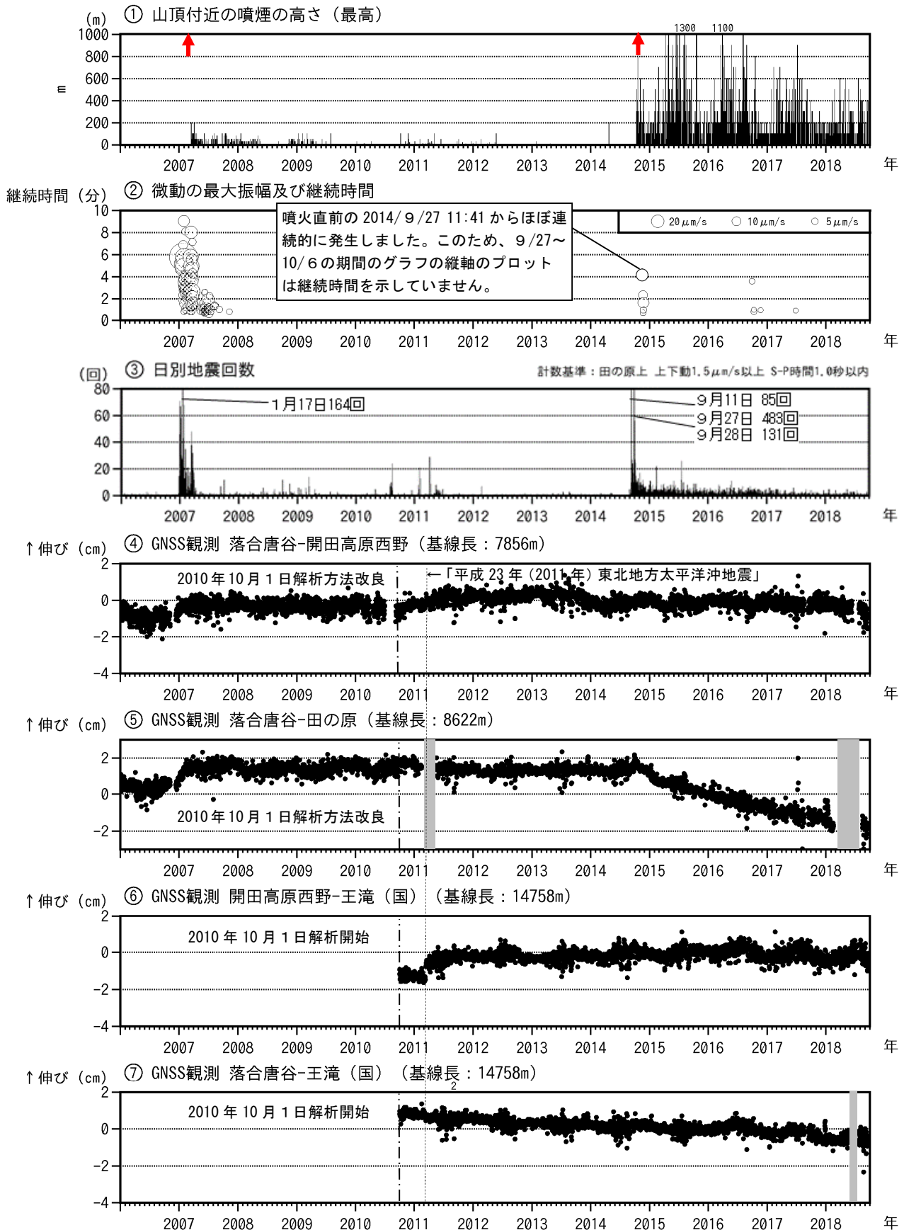
図6 御嶽山 長期間の火山活動経過図（2006年1月1日～2018年9月30日）
