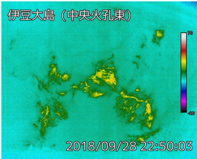
2018 年 9 月 28 日、中央火孔東監視カメラによる
