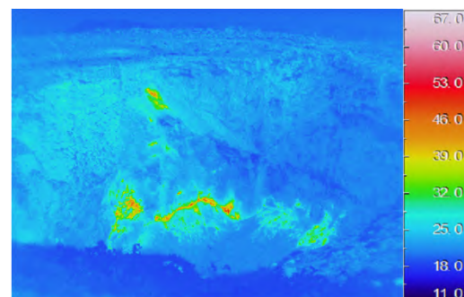
2017年9月15日08時40分 気温：17、薄曇り
