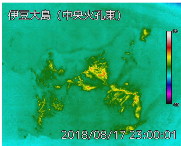
2018 年 8 月 17 日、中央火孔東監視カメラによる
