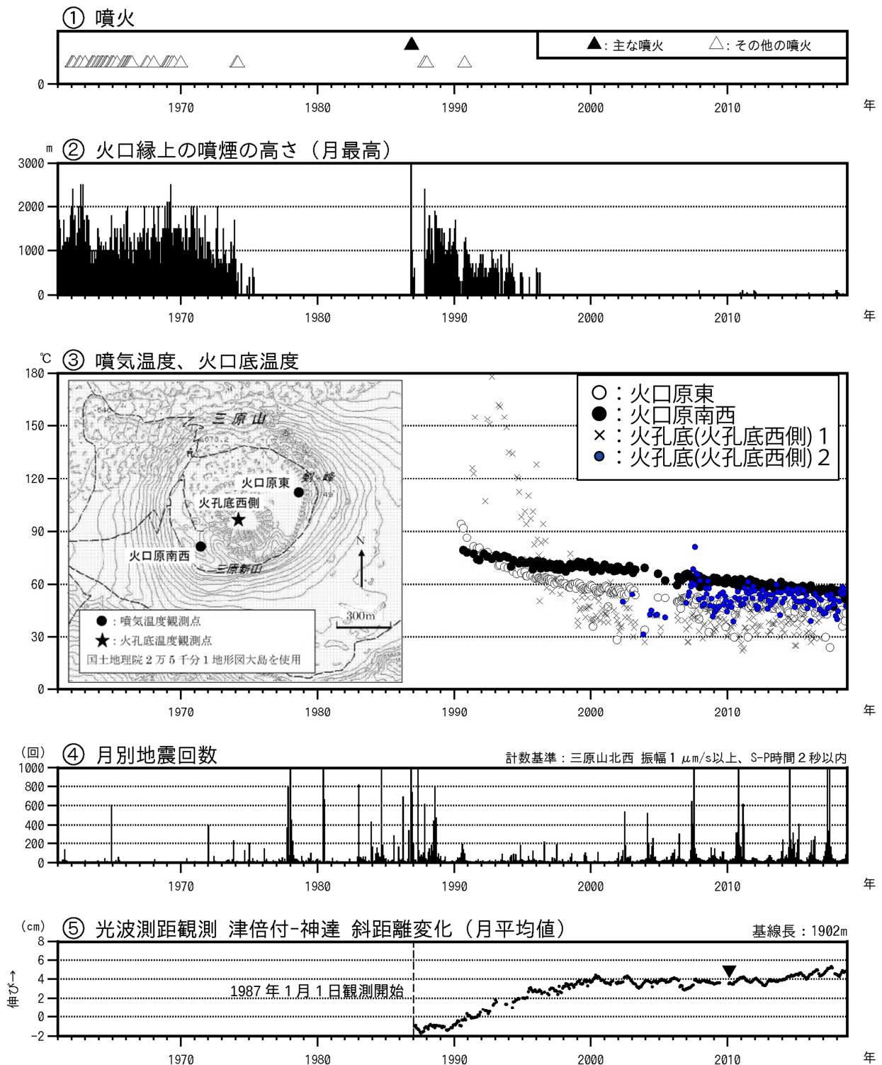
図 1 伊豆大島 長期間の火山活動経過図（1961 年 1 月～2018 年 9 月 30 日）
