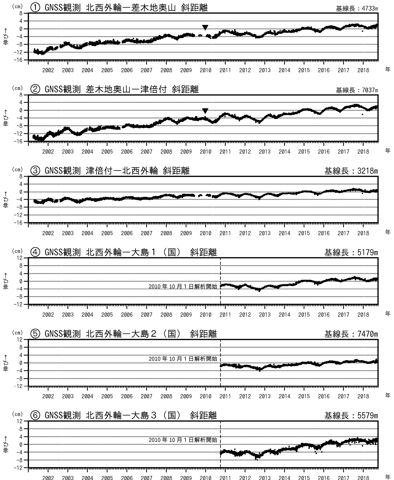
図3 伊豆大島 GNSS 連続観測による基線長変化(2001年1月～2018年9月30日)
