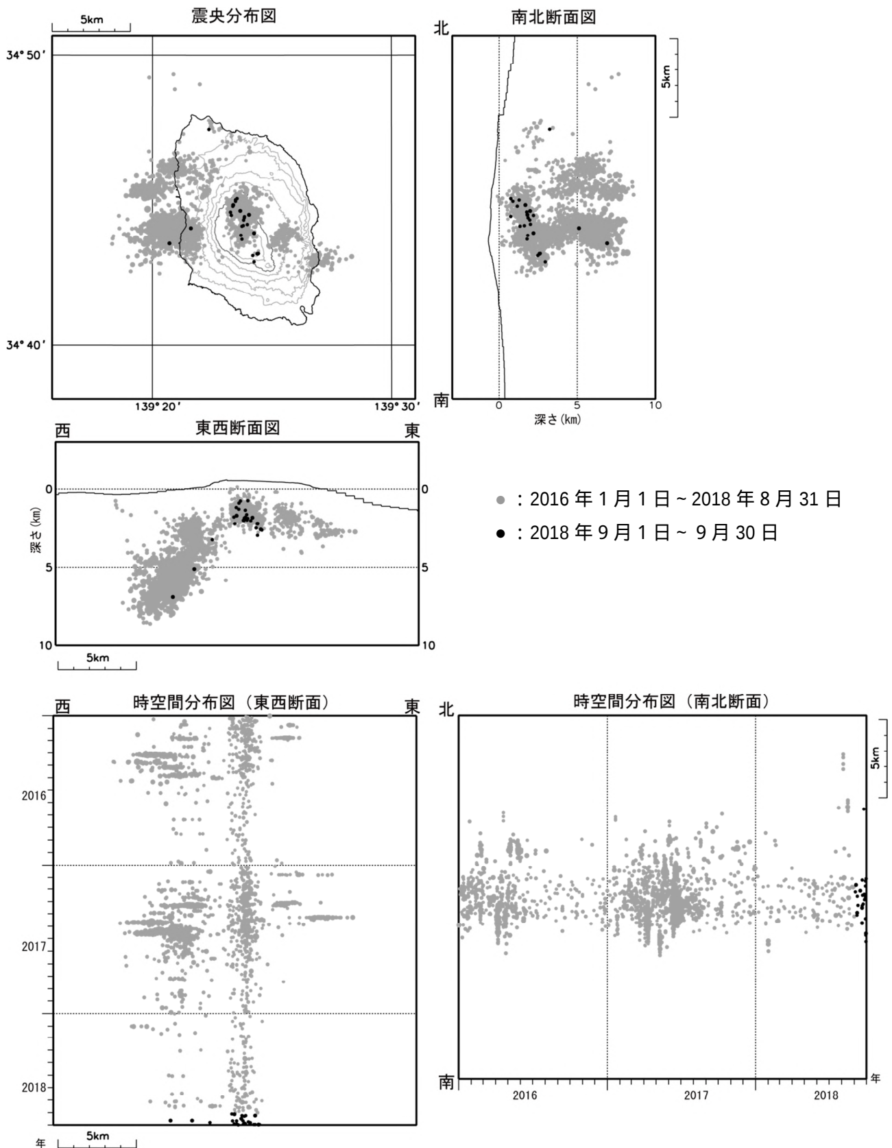
図 4 伊豆大島 震源分布図（2016 年 1 月 1 日 ~ 2018 年 9 月 30 日）
