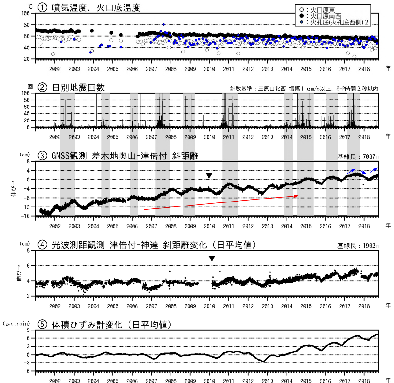
図 2 伊豆大島 最近の火山活動経過図（2001 年 1 月～2018 年 9 月 30 日）
