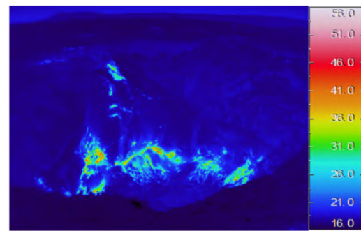
2018年9月12日04時43分 気温：16、曇り
