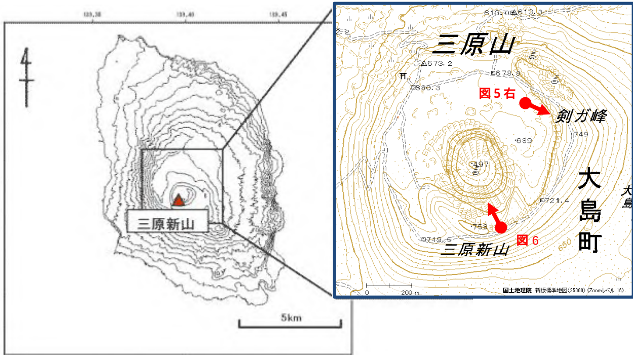
図 8 伊豆大島 現地調査での撮影場所と撮影方向（赤丸：撮影場所、→：撮影方向）
