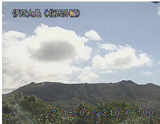
山頂部（9月23日、北西外輪監視カメラによる）
