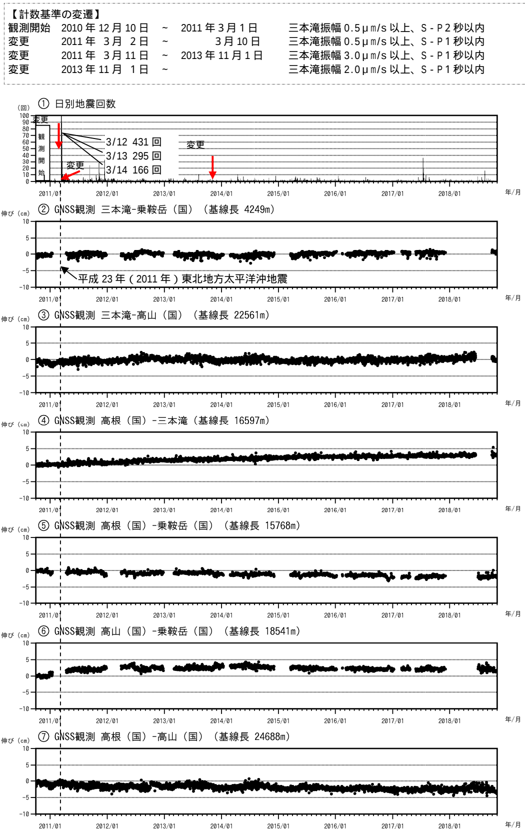
図 2 乗鞍岳 火山活動経過図
