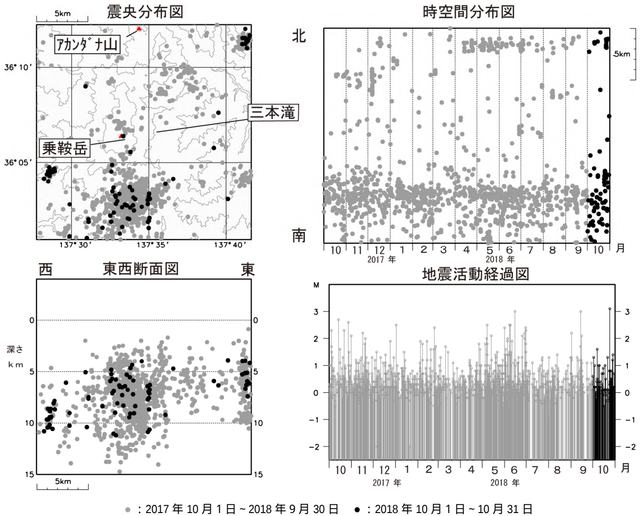
図 3 乗鞍岳 広域地震観測網による山体・周辺の地震活動(2017 年 10 月 1 日～2018 年 10 月 31 日) 広域地震観測網により震源決定したもので、深さは全て海面以下として決定しています。M (マグニチュード) は地震の規模を表します。図中の震源要素は一部暫定値が含まれており、後日変更することがあります。 ・乗鞍岳付近の地震活動は、低調に経過しています。 ・乗鞍岳から南方へ約 6 km 離れたところでまとまった地震活動がみられますが、構造的な地震で乗鞍岳の火山活動とは関係ないとみています。
