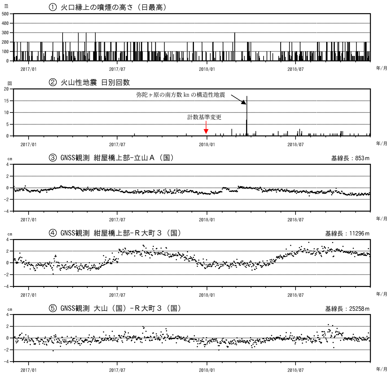
図4 弥陀ヶ原 最近の火山活動経過図（2016 年 12 月 1 日～2018 年 11 月 30 日）
