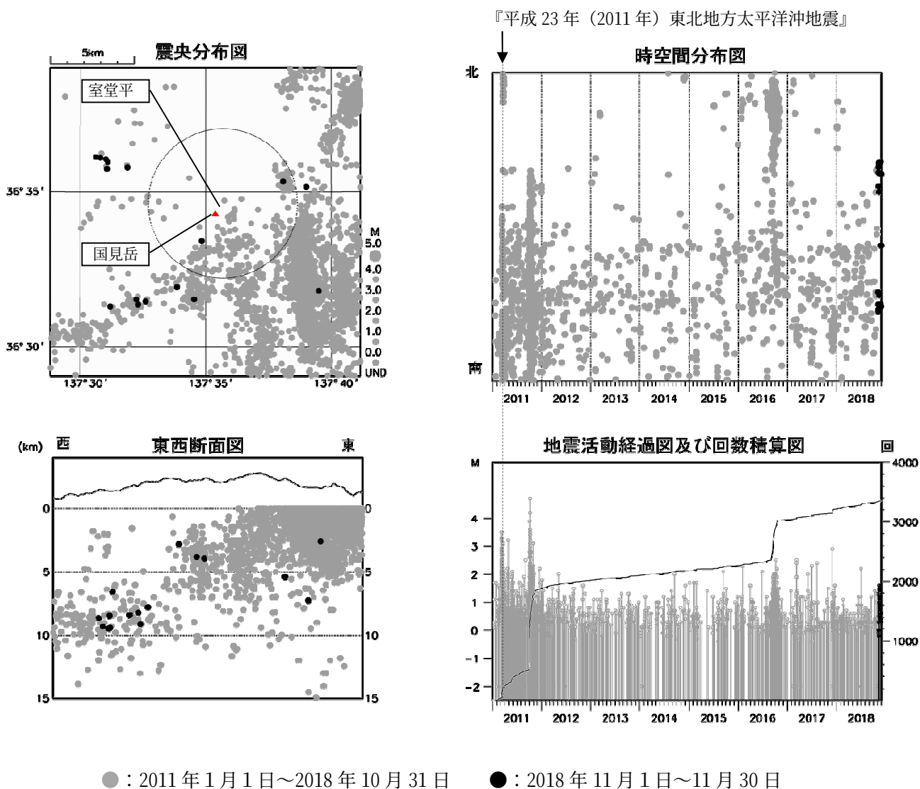
図2 弥陀ヶ原 広域地震観測網による山体・周辺の地震活動（2011 年 1 月 1 日～2018 年 11 月 30 日）
