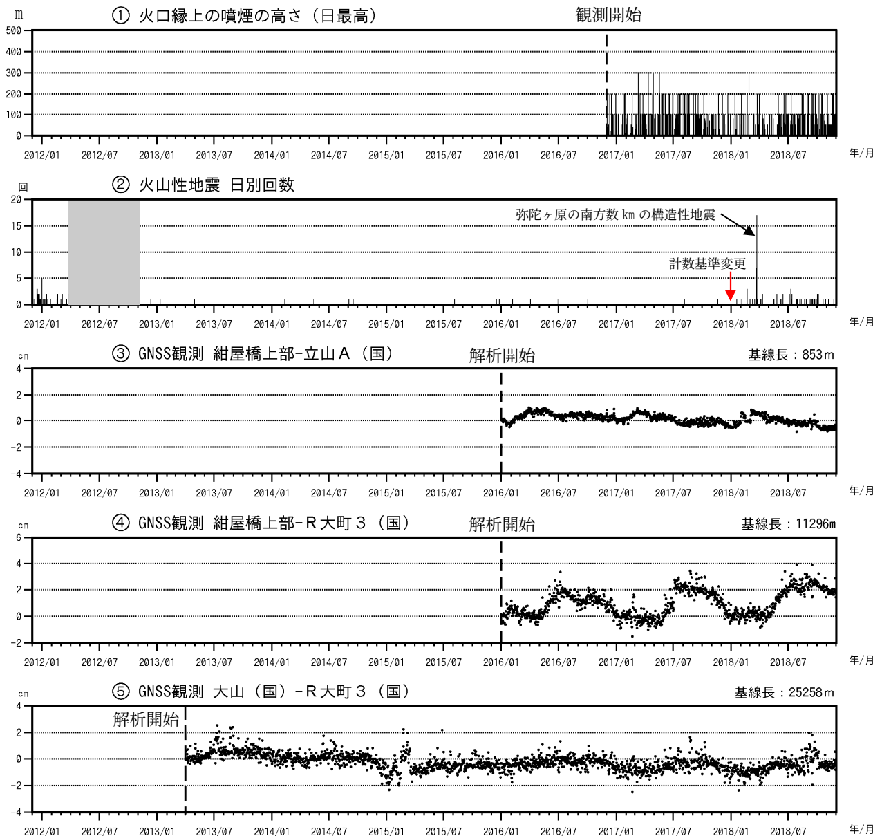
図3 弥陀ヶ原 火山活動経過図（2011 年 12 月 1 日～2018 年 11 月 30 日）
