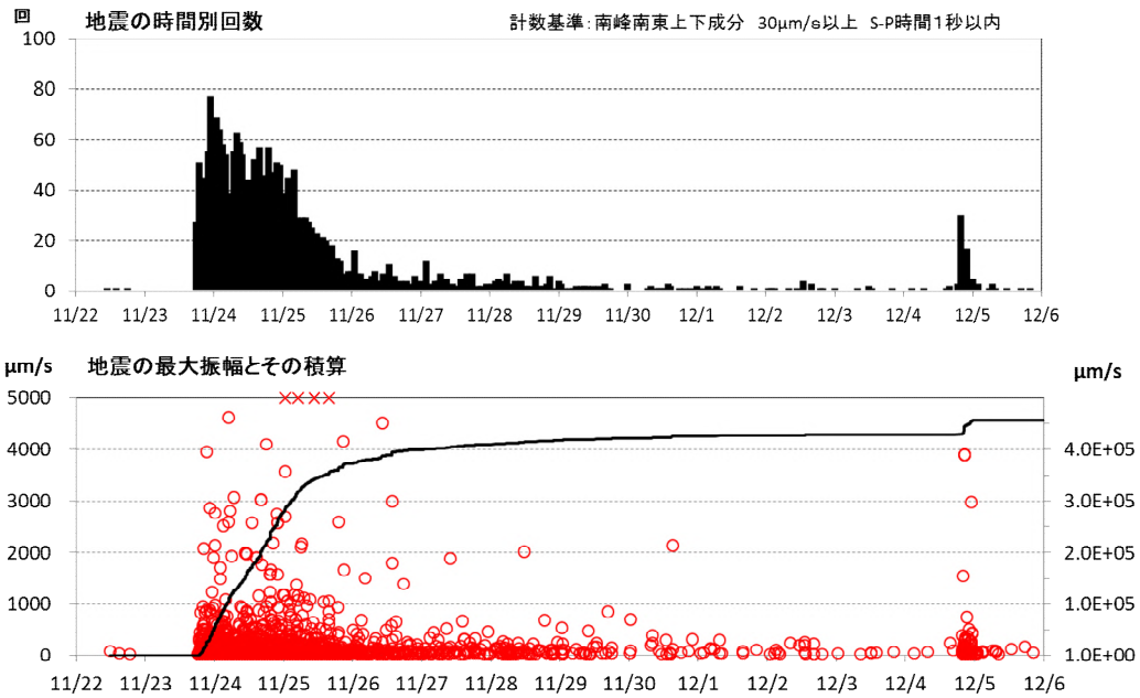
図 1 焼岳 やや振幅の大きな地震の時間別回数と振幅（2018 年 11 月 22 日～2018 年 12 月 5 日）
