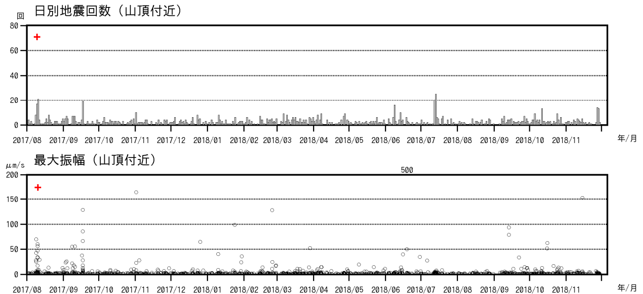
図 2 焼岳 山頂付近の地震回数、および南峰南東観測点上下動最大振幅 （2017 年 8 月 1 日～2018 年 12 月 5 日）
