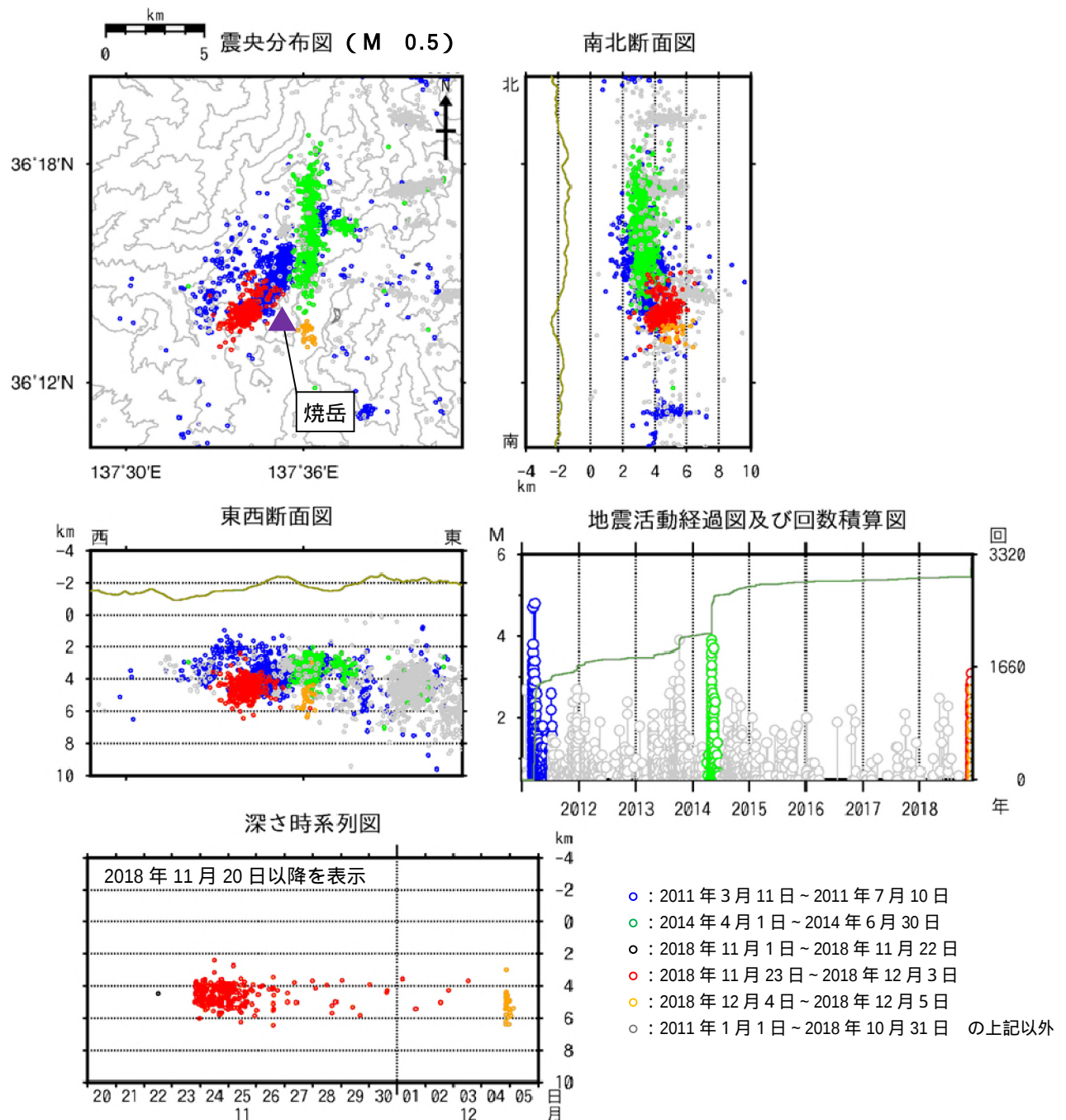
図3 焼岳 広域地震観測網による山体及び周辺の地震活動(2011年1月1日~2018年12月5日)
