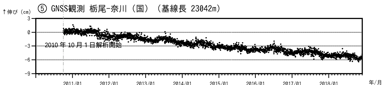
図 6 焼岳 火山活動経過図（2010年 8 月 2 日～2018年11月30日）
