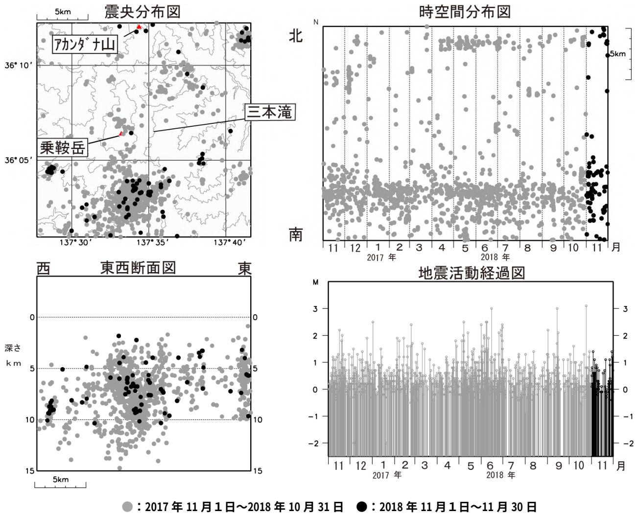
図 3 乗鞍岳 広域地震観測網による山体・周辺の地震活動(2017 年 11 月 1 日～2018 年 11 月 30 日) 広域地震観測網により震源決定したもので、深さは全て海面以下として決定しています。M（マグニチュード）は地震の規模を表します。図中の震源要素は一部暫定値が含まれており、後日変更することがあります。 ・乗鞍岳付近の地震活動は、低調に経過しています。 ・乗鞍岳から南方へ約 6 km 離れたところでもまとまった地震活動がみられますが、乗鞍岳の火山活動とは関係ないとみています。
