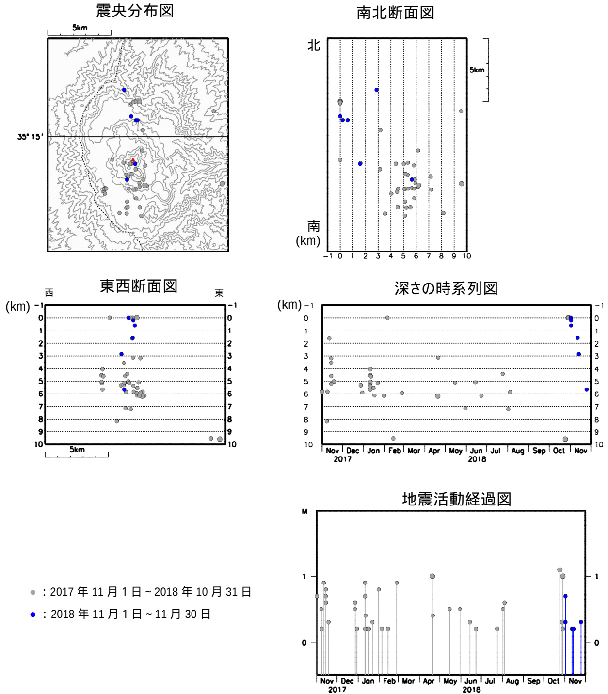
図 6 箱根山 広域地震観測網による山体周辺の震源分布図(2017 年 11 月 1 日 ~ 2018 年 11 月 30 日) M (マグニチュード) は地震の規模を表し、M0.2 以上の地震を表示しています。 広域地震観測網により震源決定したもので、深さは全て海面以下として決定しています。 図中の震源要素は一部暫定値が含まれており、後日変更することがあります。
