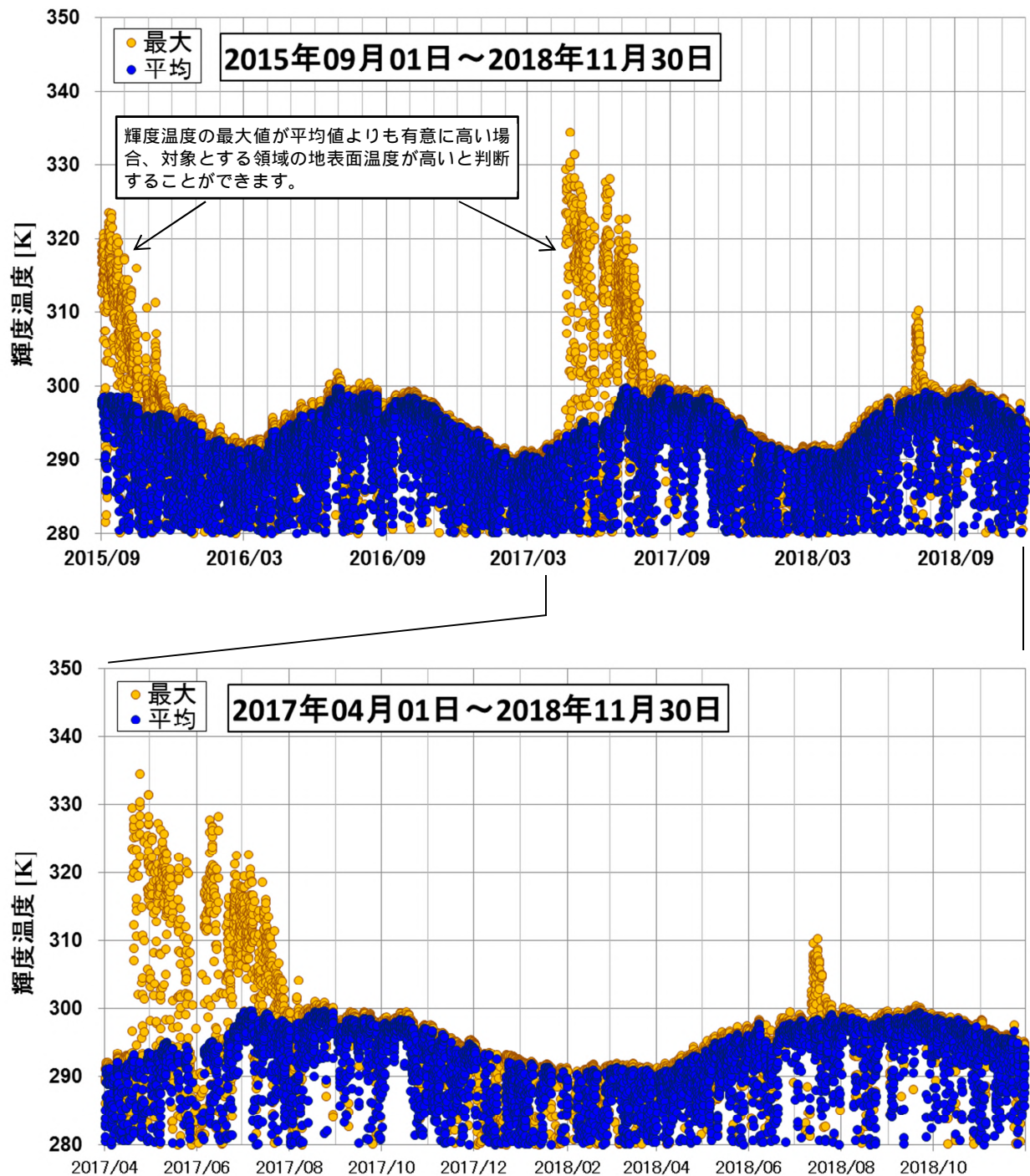
図 2 西之島 ひまわり 8 号の観測による西之島付近の輝度温度の変化
