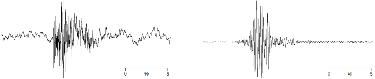
図12 草津白根山(本白根山) 主な火山性地震の特徴と波形例
