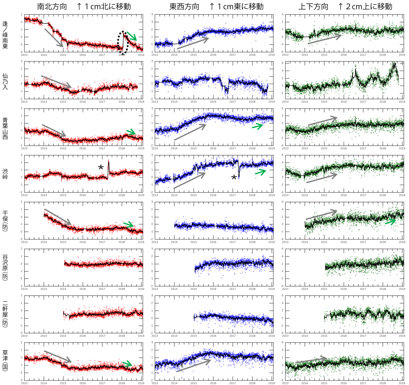
図6 草津白根山 GNSS観測による各観測点の変動(2013年1月1日~2019年1月31日) 地震等によるステップ、季節変動を除去しています。黒線は10日間の移動平均。長野(国)を固定。
