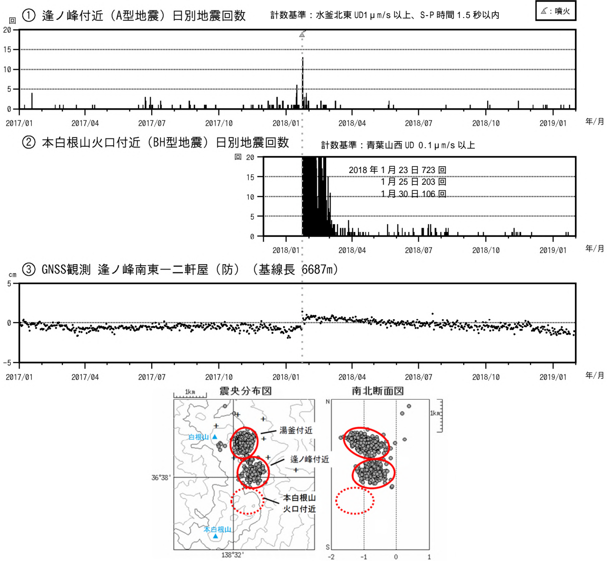
図 11 草津白根山(本白根山) 火山活動経過図(2017年1月1日~2019年1月31日)
