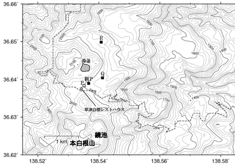
図8 草津白根山(白根山(湯釜付近)) 全磁力観測点配置図
