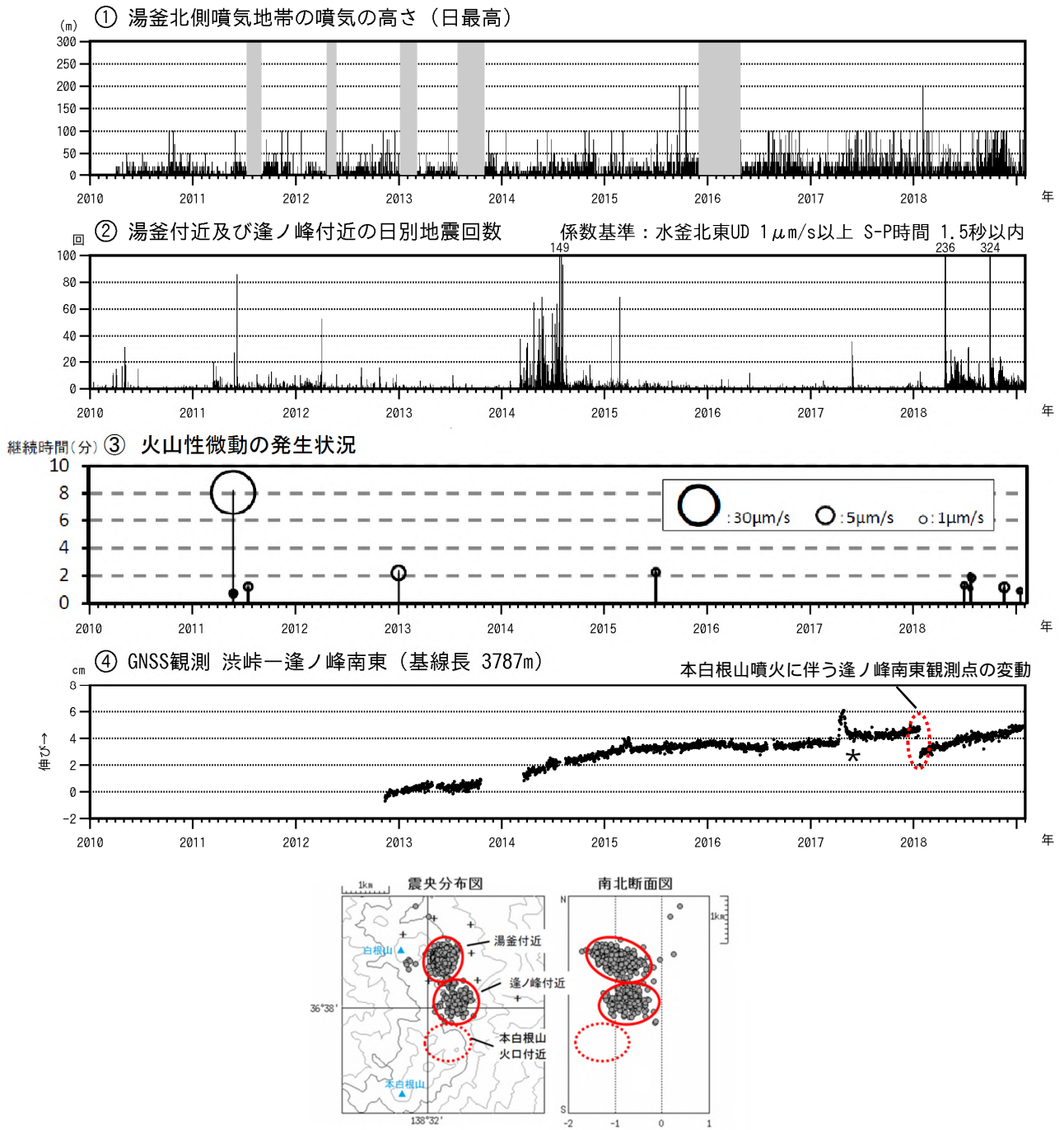
図4 草津白根山（白根山（湯釜付近））火山活動経過図（2010年1月1日～2019年1月31日） の灰色部分およびの空白部分は欠測を示します。 は図13のの基線に対応しています。 *の変動は、火山活動に起因するものではないと考えられます。 2013年1月に解析方法を変更しています。 最下段の震源分布図は、の地震の震源の概ねの位置を示しています。
