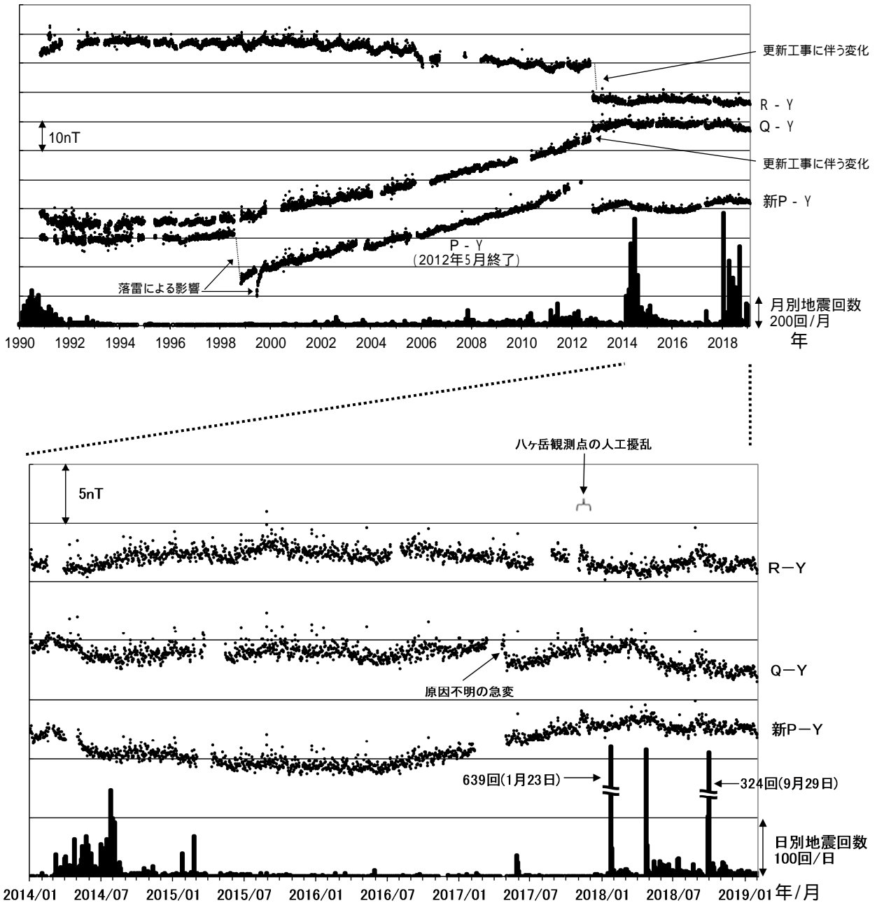
図7 草津白根山（白根山（湯釜付近））全磁力連続観測による全磁力値の変化及び地震回数
