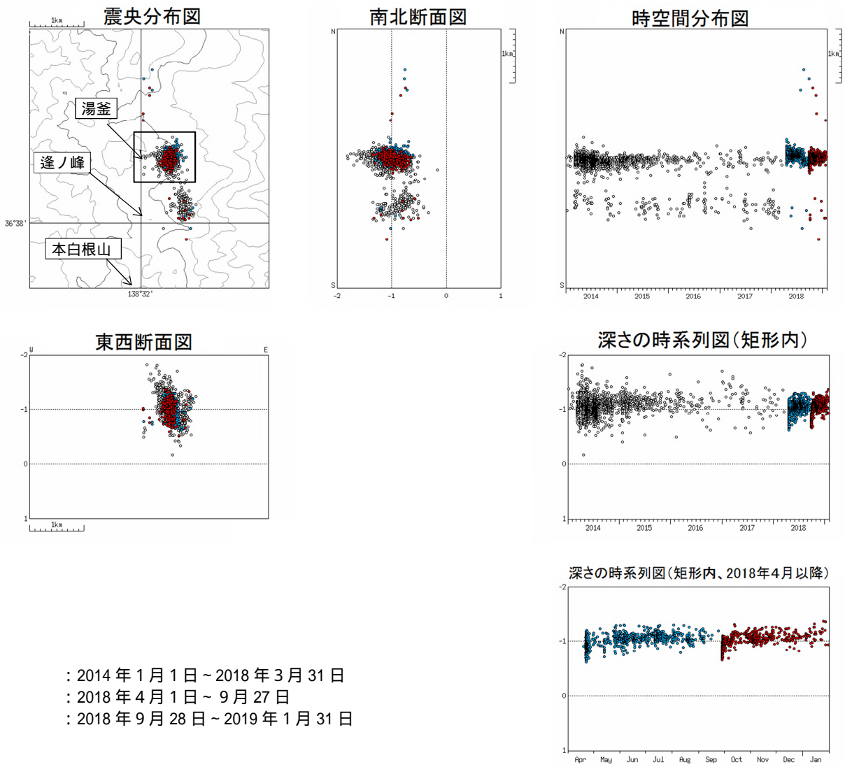
図5 草津白根山 震源分布図(2014年1月1日～2019年1月31日) 火山性地震の震源は、湯釜付近の海拔約1kmに分布しています。
