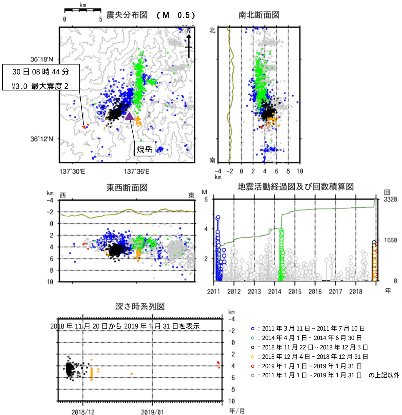
図 3 焼岳 広域地震観測網による山体及び周辺の地震活動(2011年 1 月 1 日 ~ 2019 年 1 月 31 日)
