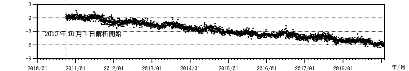
図 6 焼岳 火山活動経過図（2010年 8 月 2 日～2019 年 1 月 31 日）
