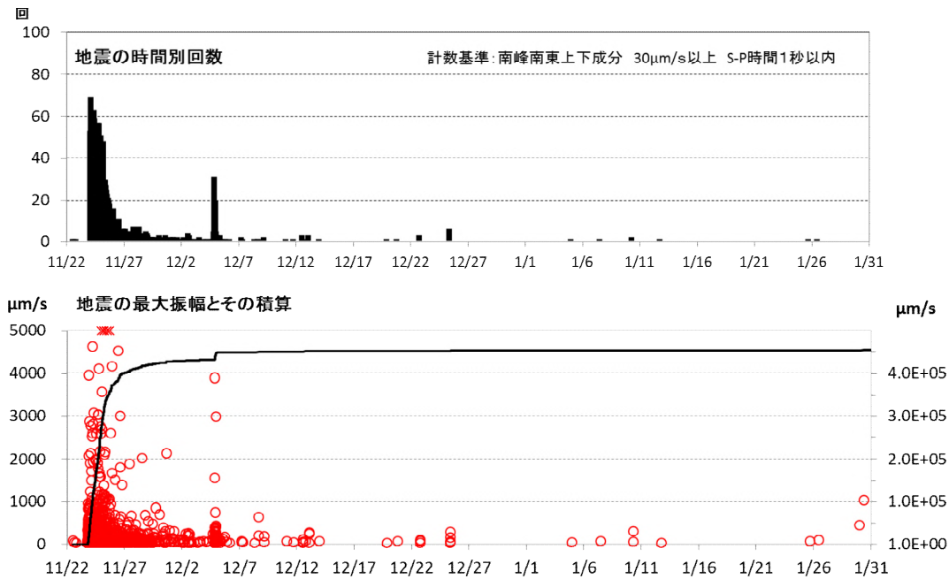
図 1 焼岳 やや振幅の大きな地震の時間別回数と振幅（2018 年 11 月 22 日～2019 年 1 月 31 日）
