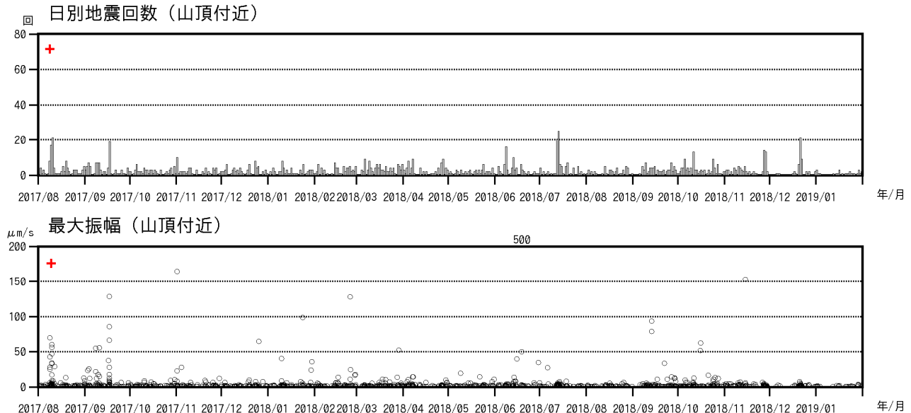
図 2 焼岳 山頂付近の地震回数、および南峰南東観測点上下動最大振幅 （2017 年 8 月 1 日～2019 年 1 月 31 日）
