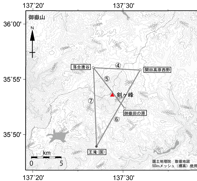
図 5 御嶽山 GNSS 連続観測点と基線番号
