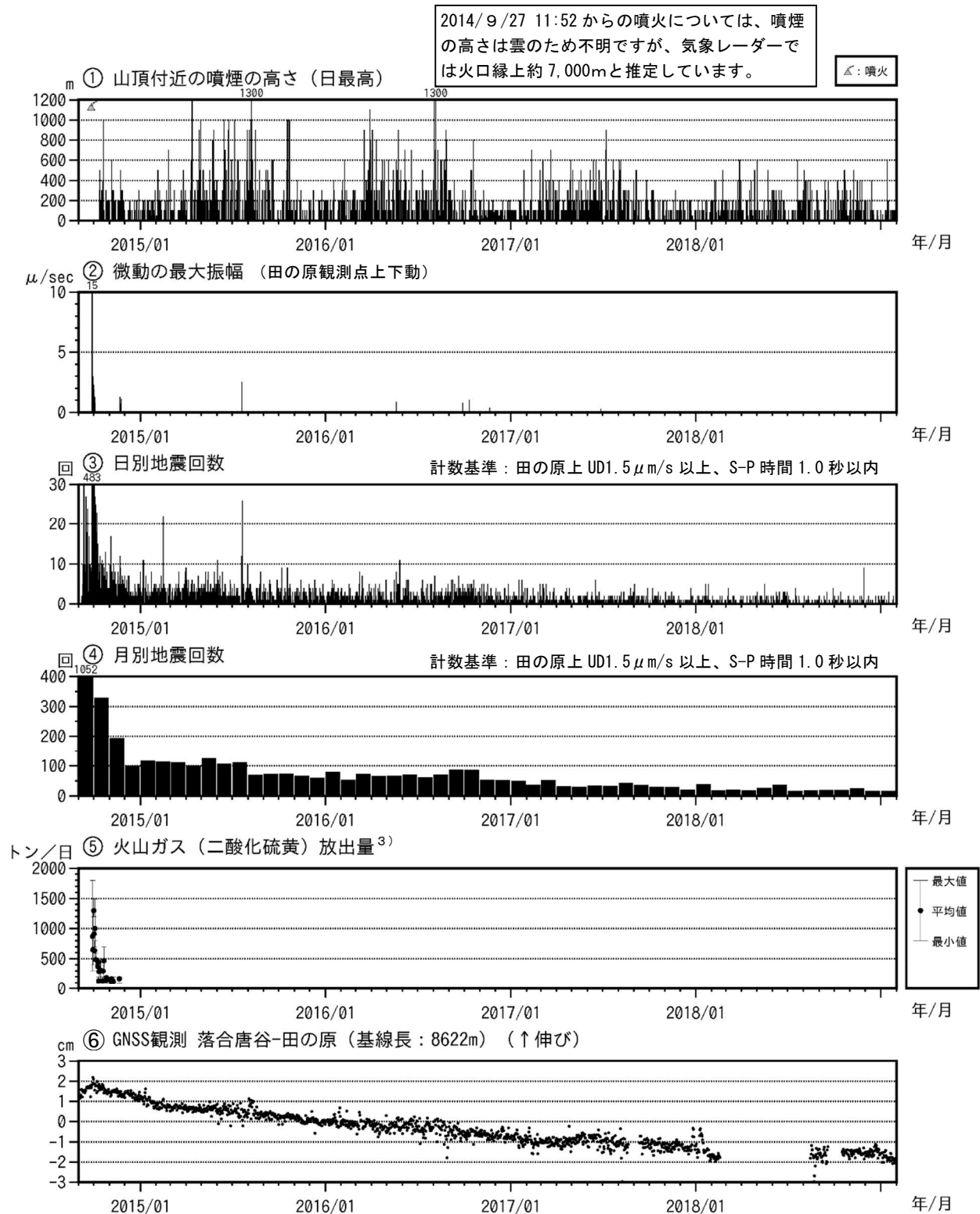
図 3 御嶽山 最近の火山活動経過図（2014 年 9 月 1 日～2019 年 1 月 31 日）
