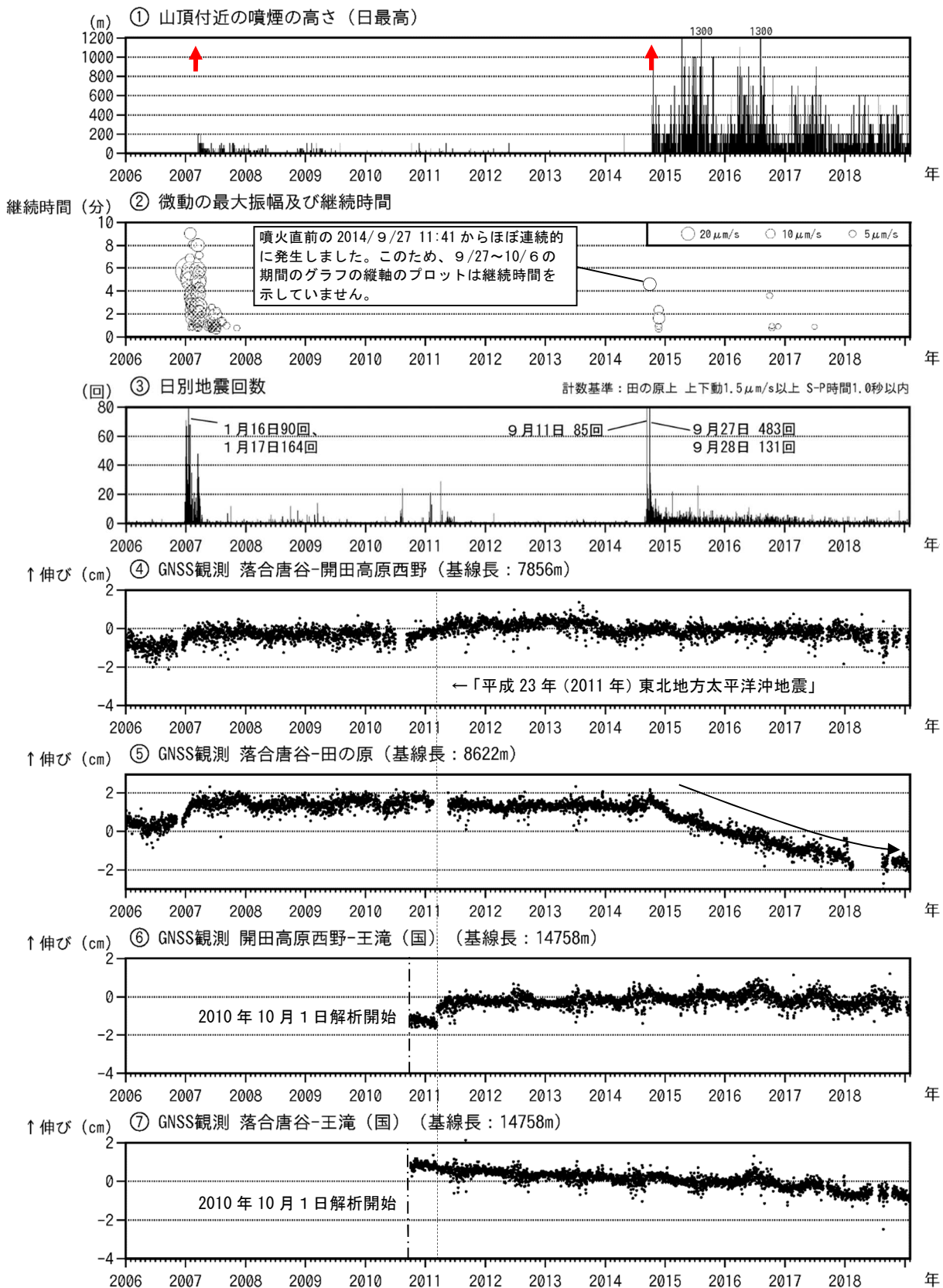
図 4 御嶽山 長期間の火山活動経過図（2006 年 1 月 1 日～2019 年 1 月 31 日）
