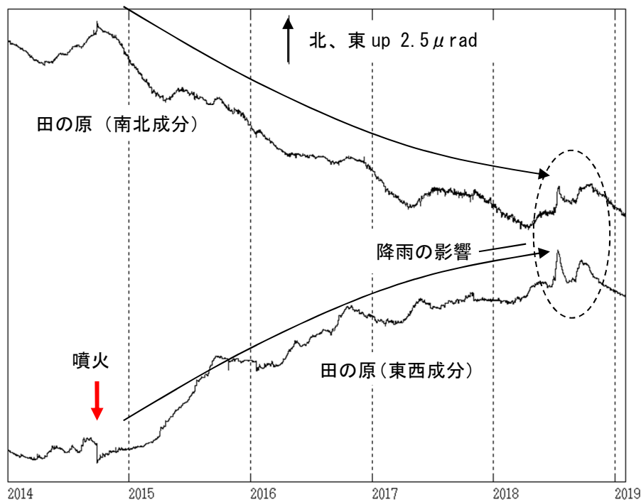
図 6 御嶽山 田の原観測点の傾斜変動（2014 年 1 月 1 日～2019 年 1 月 31 日）
