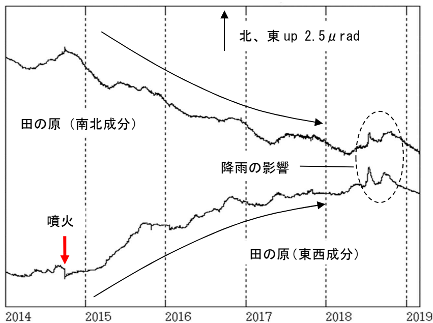
図 7 御嶽山 田の原観測点の傾斜変動（2014 年 1 月 1 日～2019 年 2 月 28 日）
