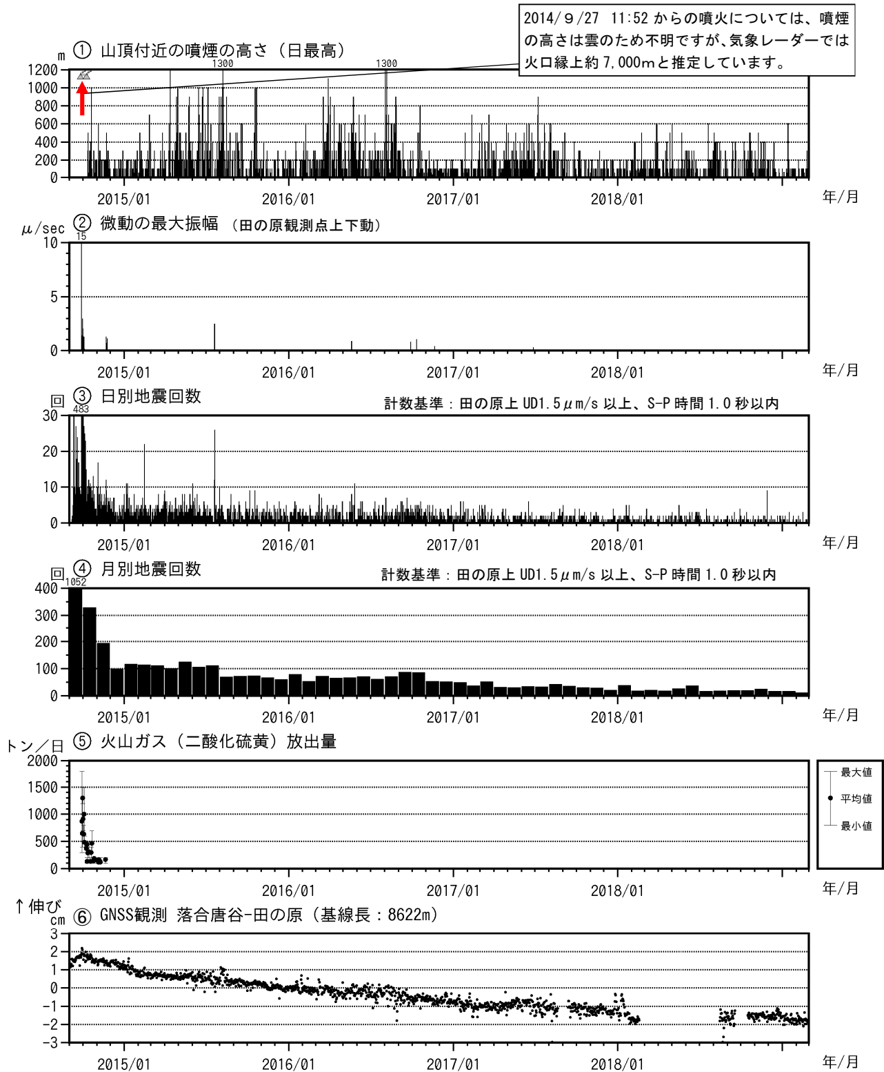
図 4 御嶽山 最近の火山活動経過図（2014 年 9 月 1 日～2019 年 2 月 28 日）
