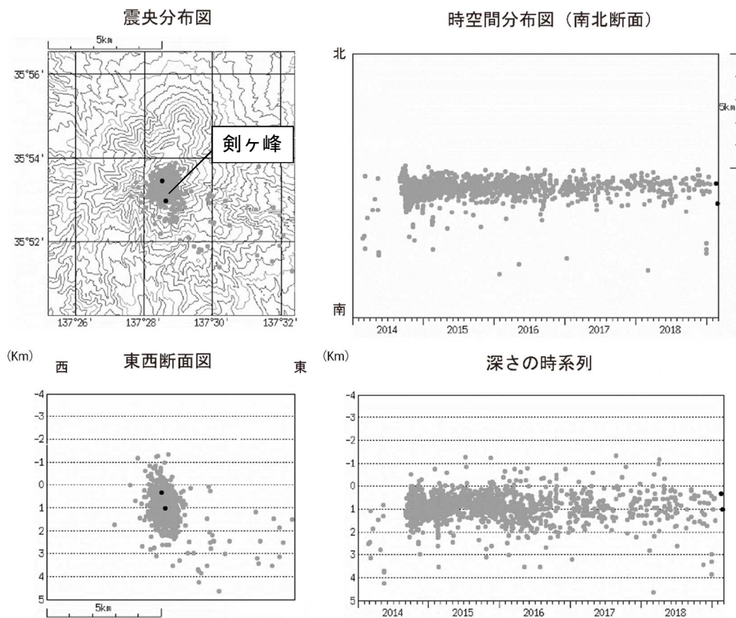
図 2 御嶽山 震源分布図（2014 年 1 月 1 日～2019 年 2 月 28 日）
