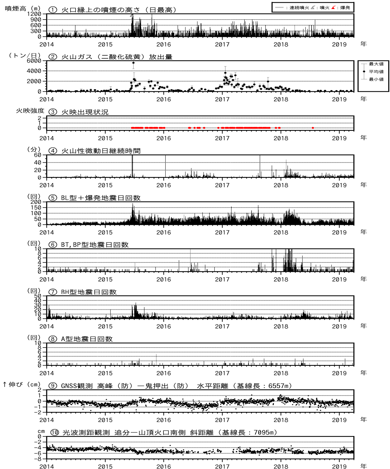
図4 浅間山 最近の火山活動経過図（2014 年 1 月 1 日～2019 年 3 月 31 日）
