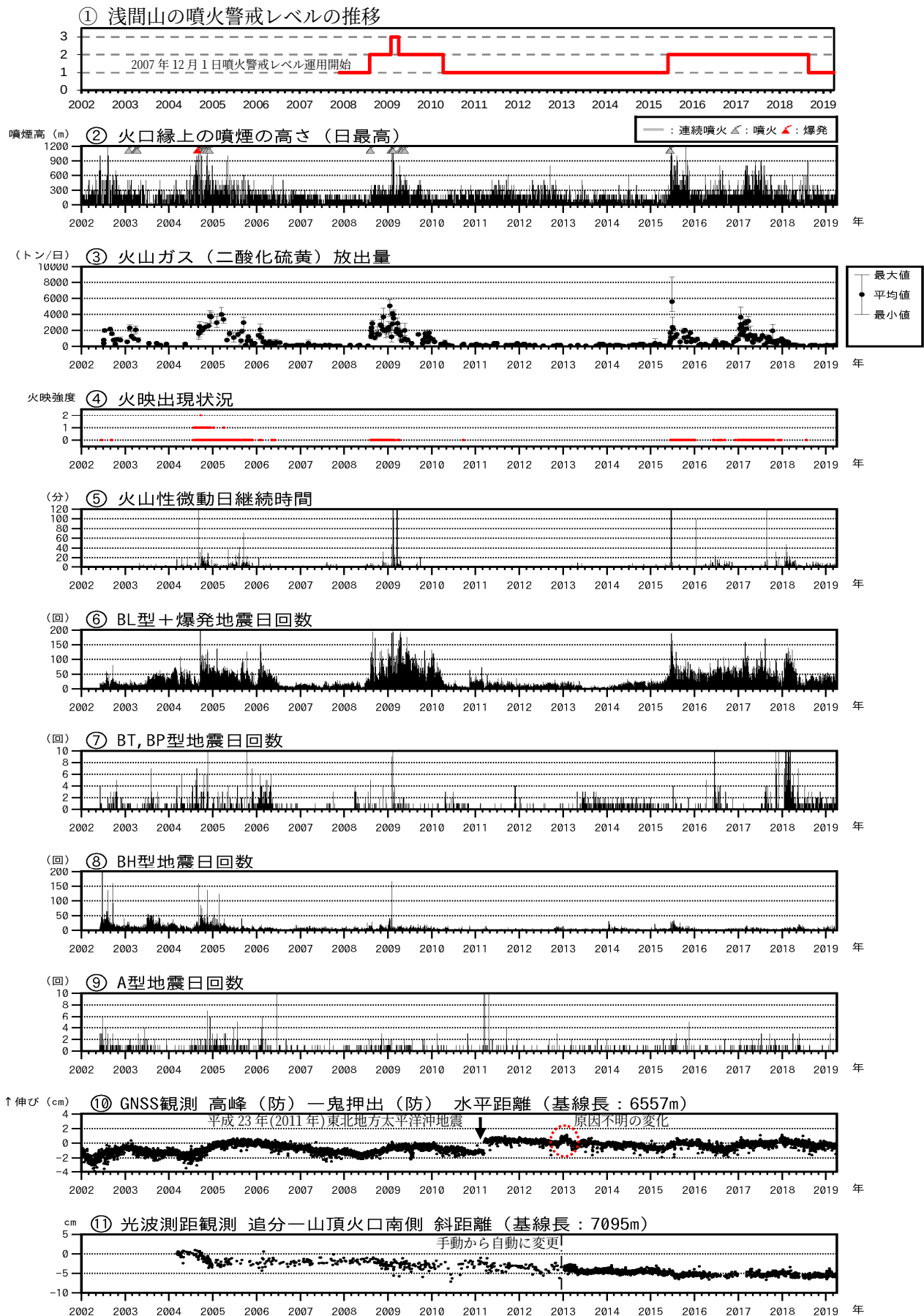
図3 浅間山 火山活動経過図（2002年1月1日～2019年3月31日）
