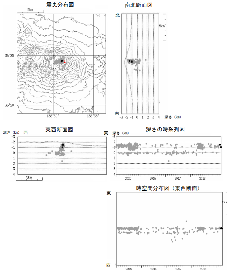
図6 浅間山 震源分布図（2015年1月1日～2019年3月31日）
