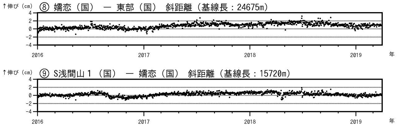
図 7-2 浅間山 GNSS 連続観測結果(2016 年 1 月 1 日～2019 年 3 月 31 日)
