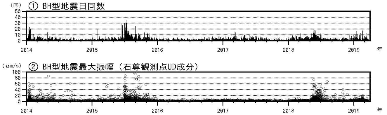
図5 浅間山 BH型地震の日別回数とその最大振幅（2014年1月1日～2019年3月31日）
