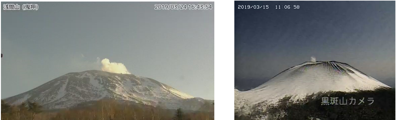
図1 浅間山 山頂部の状況
