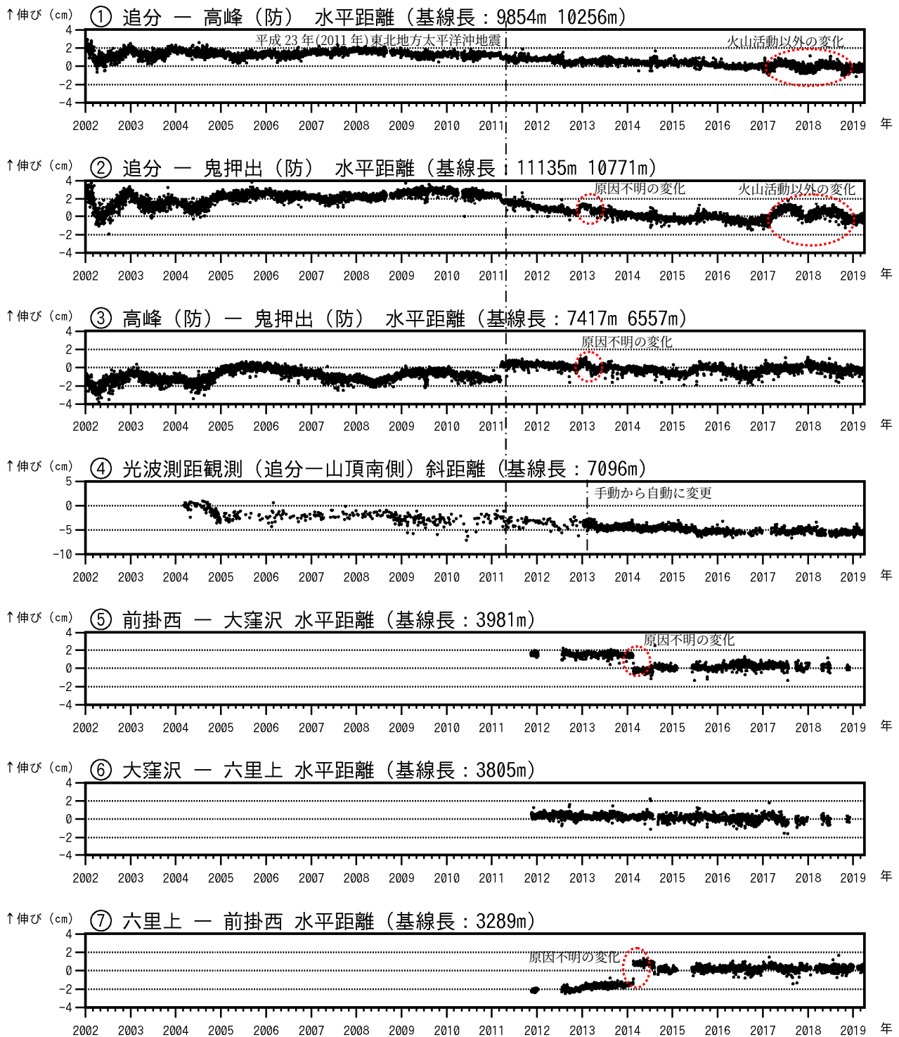
図 7-1 浅間山 GNSS 連続観測及び光波測距観測の結果(2002 年 1 月 1 日～2019 年 3 月 31 日) 2010 年 10 月及び 2016 年 1 月以降のデータについては、解析方法を改良しています。
