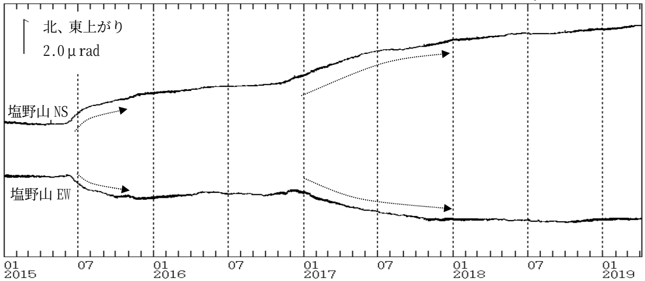
図9 浅間山 塩野山観測点における傾斜データ（2015 年 1 月 1 日～2019 年 3 月 31 日）
