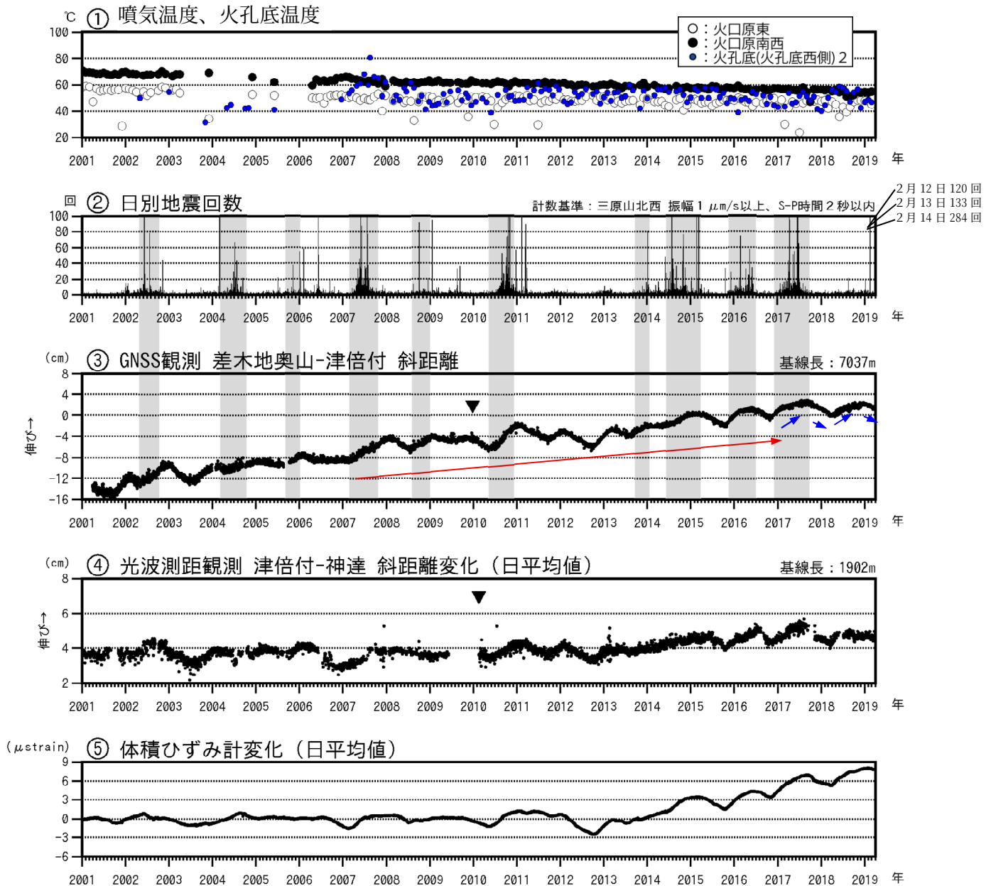
図2 伊豆大島 最近の火山活動経過図（2001年1月～2019年3月31日）
