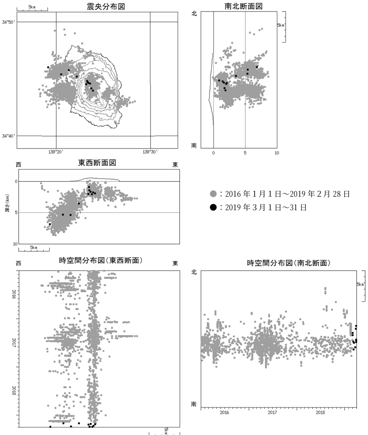
図4 伊豆大島 震源分布図（2016 年 1 月 1 日～2019 年 3 月 31 日）
