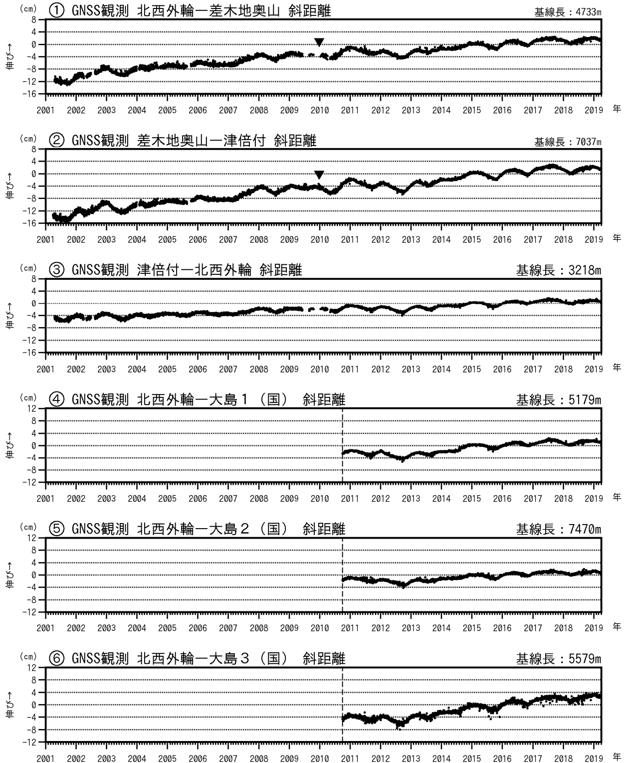
図3 伊豆大島 GNSS連続観測による基線長変化(2001年1月～2019年3月31日)
