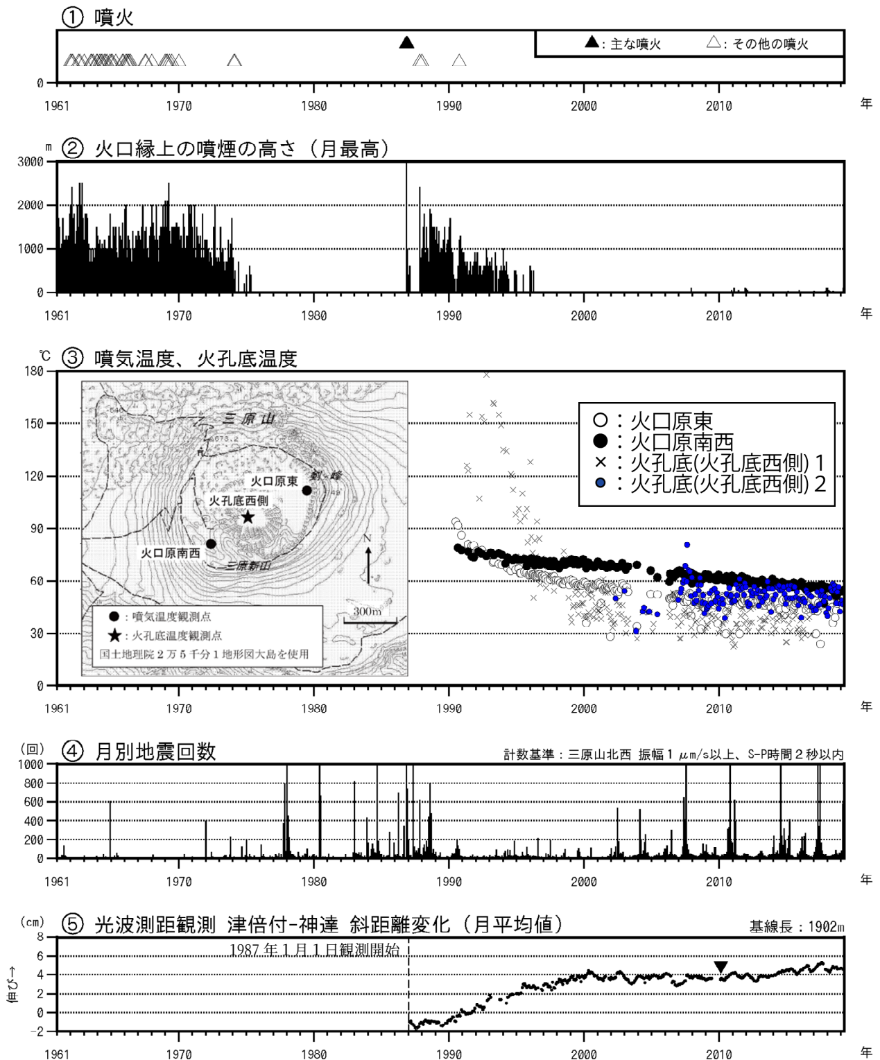
図 1 伊豆大島 長期間の火山活動経過図（1961 年 1 月～2019 年 3 月 31 日）
