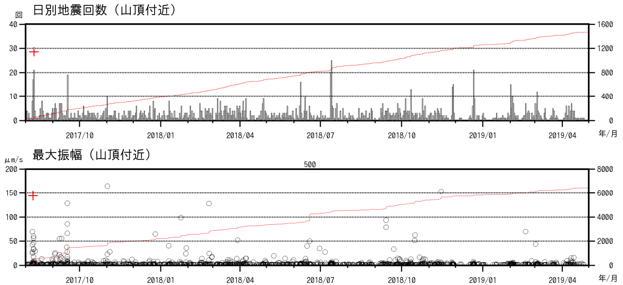
図2 焼岳 山頂付近の地震回数、および南峰南東観測点上下動最大振幅 (2017年8月1日～2019年4月30日)
