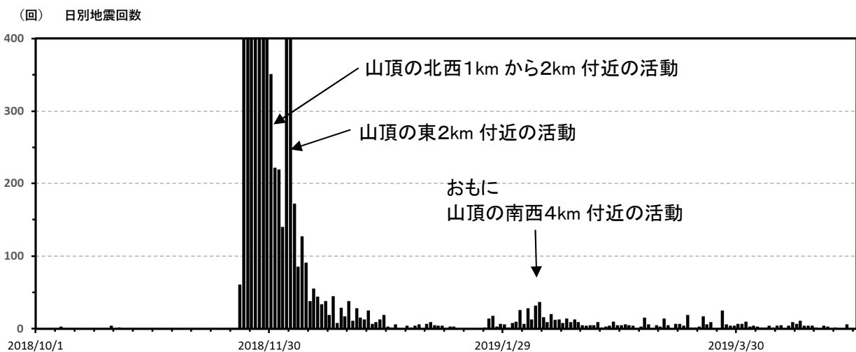
図3 焼岳 焼岳周辺の日別地震回数(2018年10月1日～2019年4月30日)
