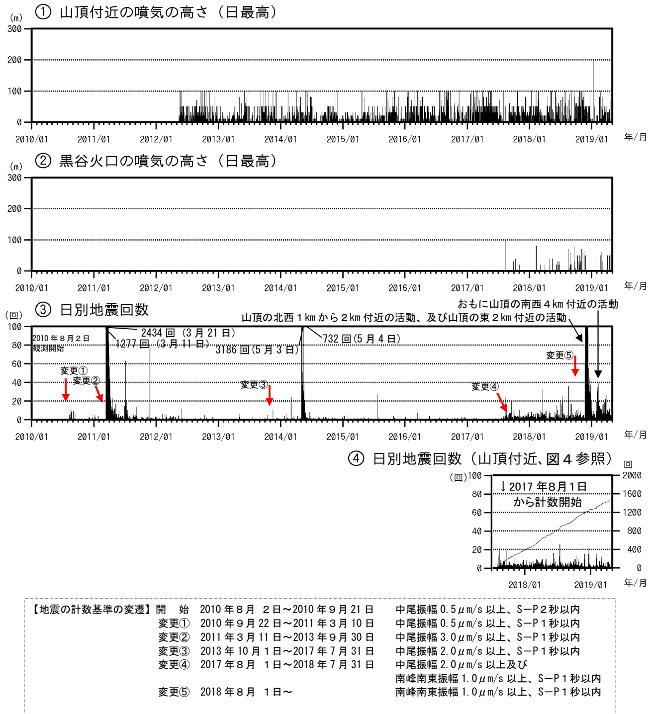
図 1 焼岳 噴気の高さと地震回数の推移 (2010 年 1 月 1 日～2019 年 4 月 30 日)
