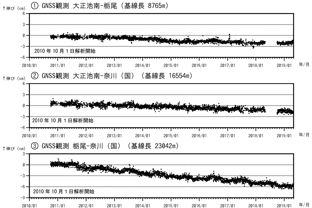
図7 焼岳 GNSS 連続観測による基線長変化（2010 年 10 月 1 日～2019 年 4 月 30 日）
