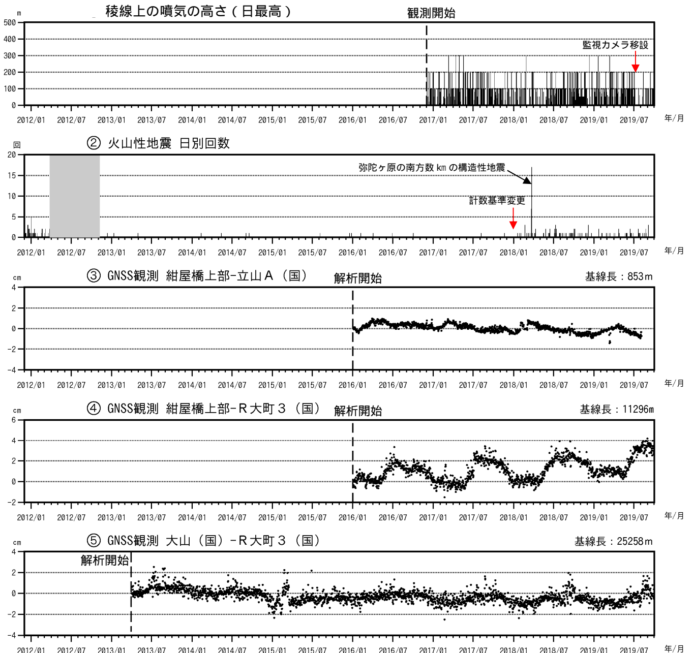
図3 弥陀ヶ原 火山活動経過図（2011年12月1日～2019年9月30日）
