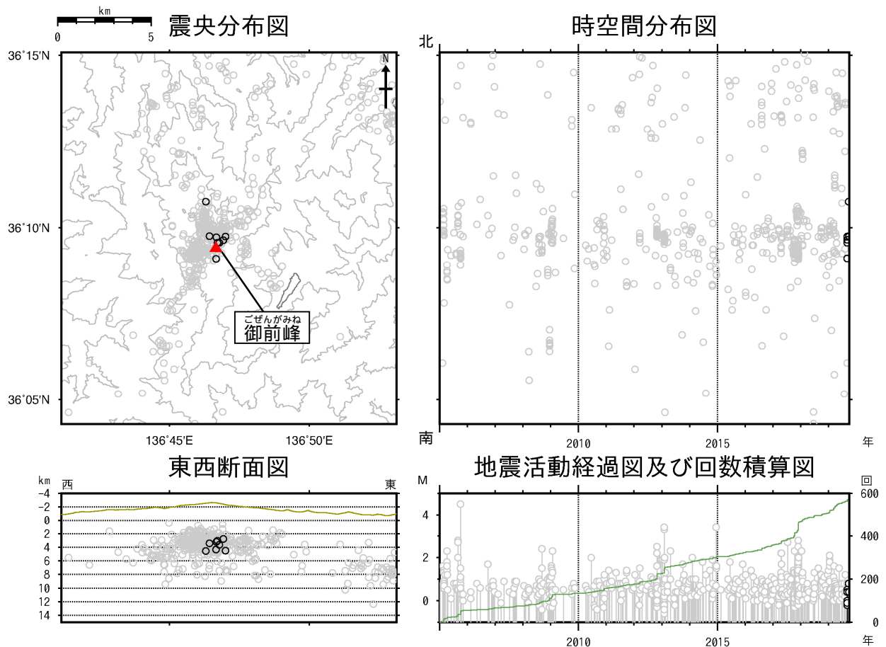
図4 白山 広域地震観測網による山体・周辺の地震活動（2005年1月1日～2019年9月30日）
