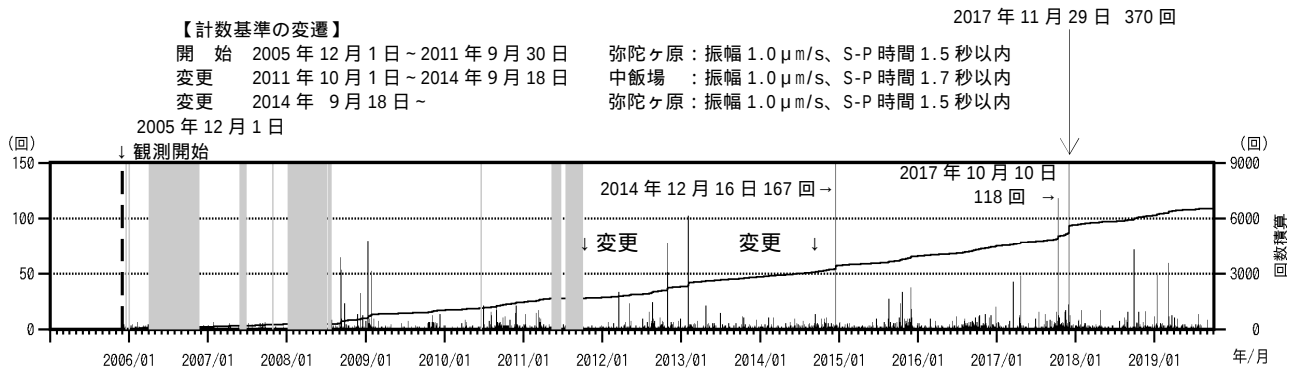
図3 白山 日別地震回数と積算回数（2005年12月1日～2019年9月30日） 図の灰色部分は機器障害による欠測期間
