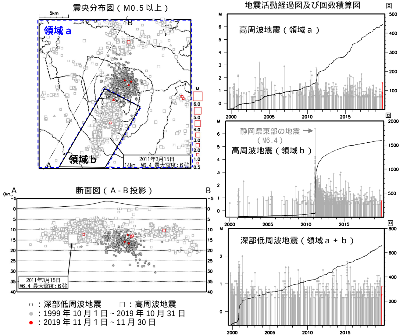
図3 富士山 広域地震観測網による山体及び周辺の地震活動（1999年10月1日～2019年11月30日）
