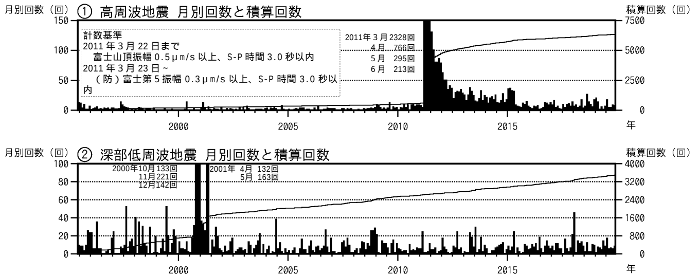
図2 富士山 月別地震回数（1995年6月1日～2019年11月30日）
