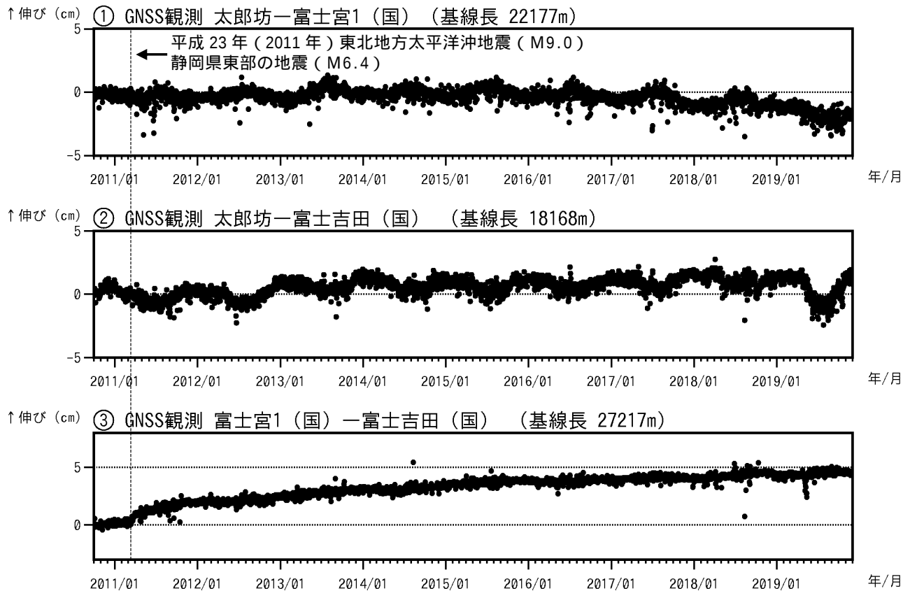
図 4 富士山 GNSS 連続観測による基線長変化 (2010 年 10 月 1 日 ~ 2019 年 11 月 30 日) (国): 国土地理院 「平成 23 年 (2011 年) 東北地方太平洋沖地震」及び 2011 年 3 月 15 日に発生した静岡県東部の地震 (M6.4) によるステップ状の変化を補正しています。 ～ は図 5 の GNSS 基線 ～ に対応しています。
