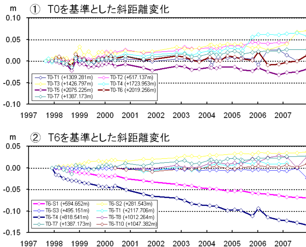
図5 伊豆大島 光波距離計の観測による斜距離変化（1997年12月～2007年12月）
