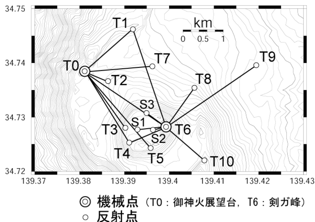
図6 伊豆大島 光波距離計繰り返し観測点配置図
