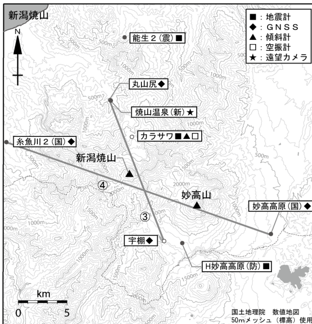
図 4 新潟焼山 観測点配置図 GNSS 基線 は図 2 の に対応しています。
