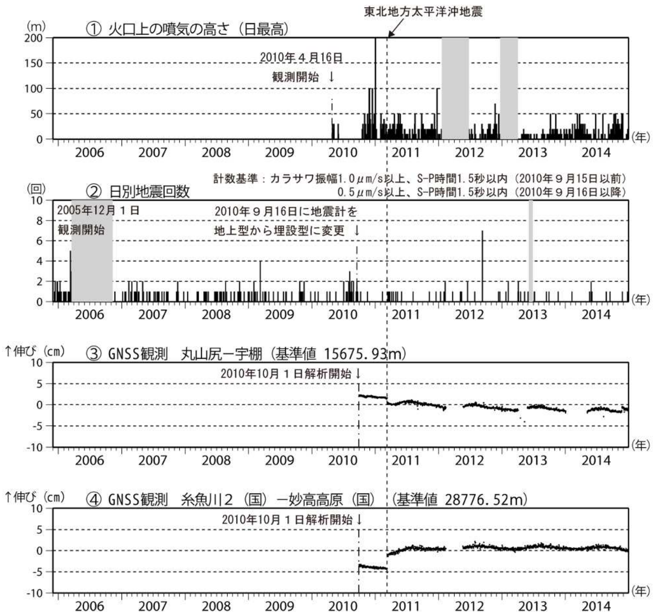
図2 新潟焼山 火山活動の推移 (2005年12月1日～2014年12月31日)
