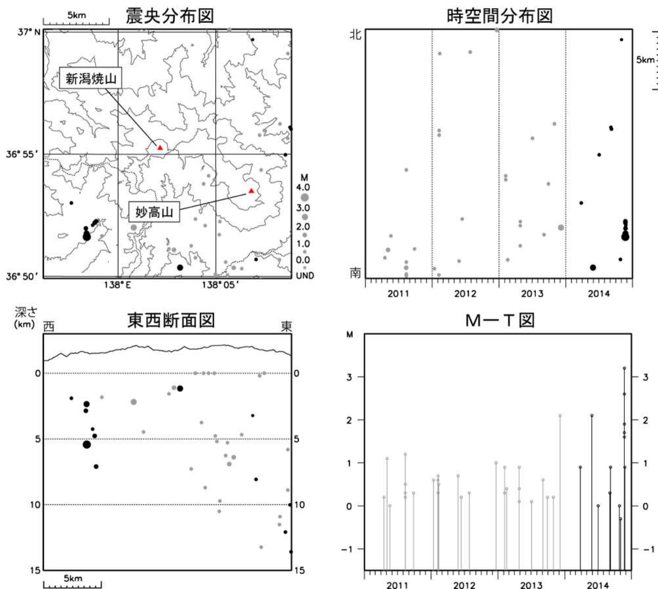
図3 新潟焼山 広域地震観測網による山体・周辺の地震活動(2011年1月1日～2014年12月31日)
