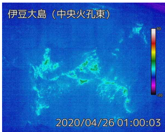
2020年4月26日、中央火孔東監視カメラによる
