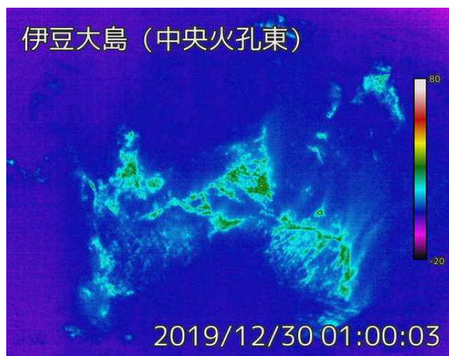
2019年12月30日、中央火孔東監視カメラによる
