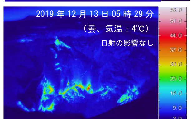
図6 伊豆大島 中央火口内の状況（撮影方向は図9参照）
