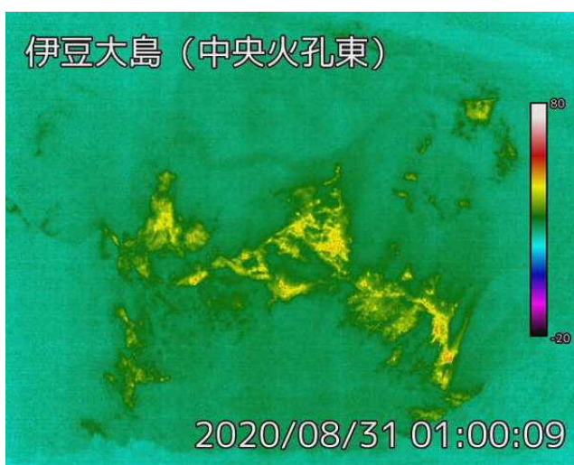
2020年8月31日、中央火孔東監視カメラによる
