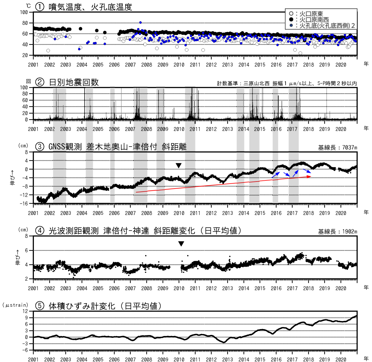
図2 伊豆大島 最近の火山活動経過図(2001年1月～2020年12月)
