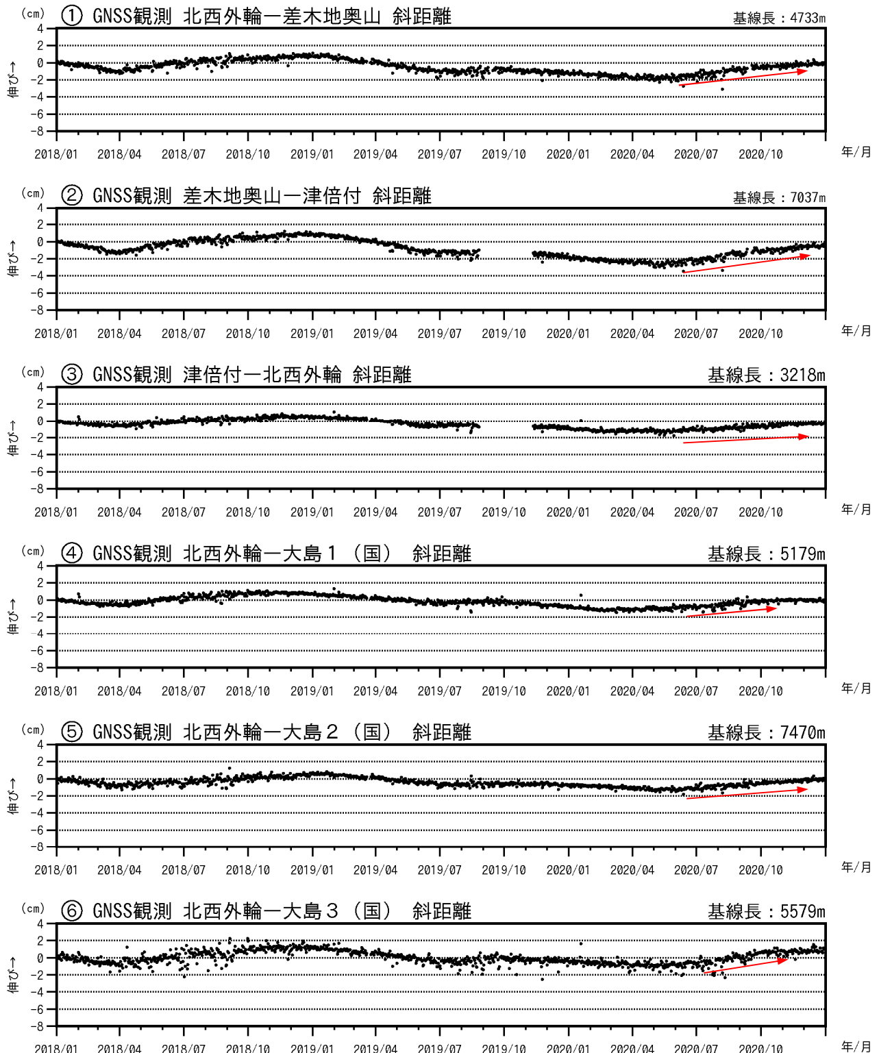
図 3-2 伊豆大島 GNSS 連続観測による基線長変化 (2018 年 1 月～2020 年 12 月 31 日)
