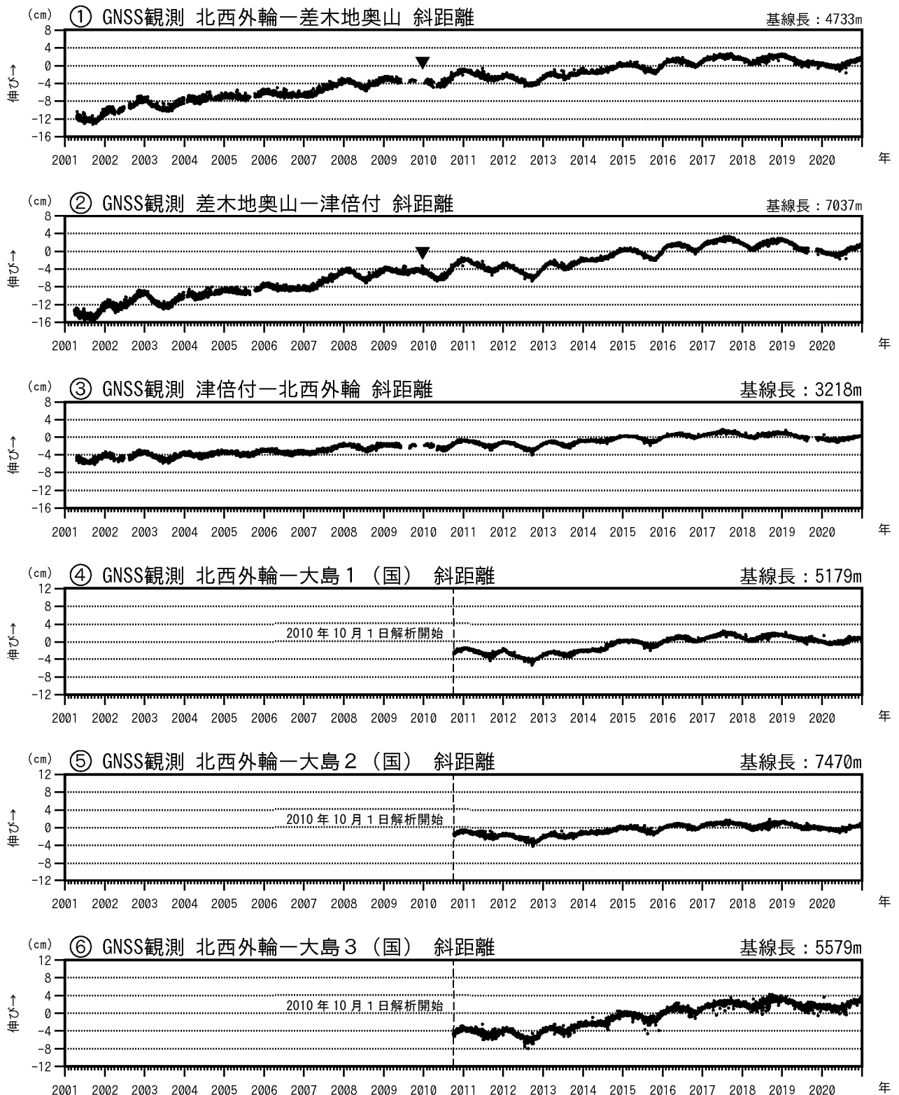
図3-1 伊豆大島 GNSS連続観測による基線長変化（2001年1月～2020年12月31日）
