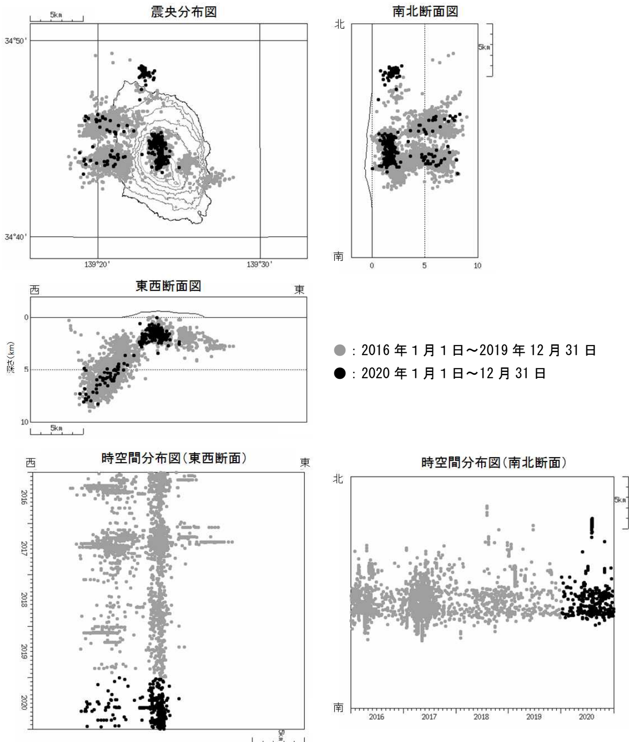
図4 伊豆大島 最近の火山性地震の震源分布(2016年1月1日～2020年12月31日)
