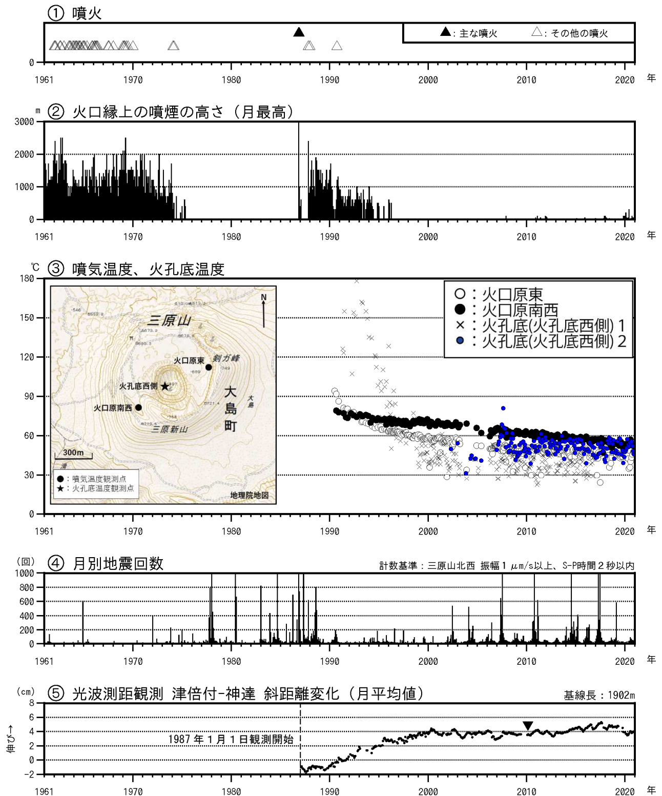
図1 伊豆大島 長期間の火山活動経過図（1961年1月～2020年12月31日）
