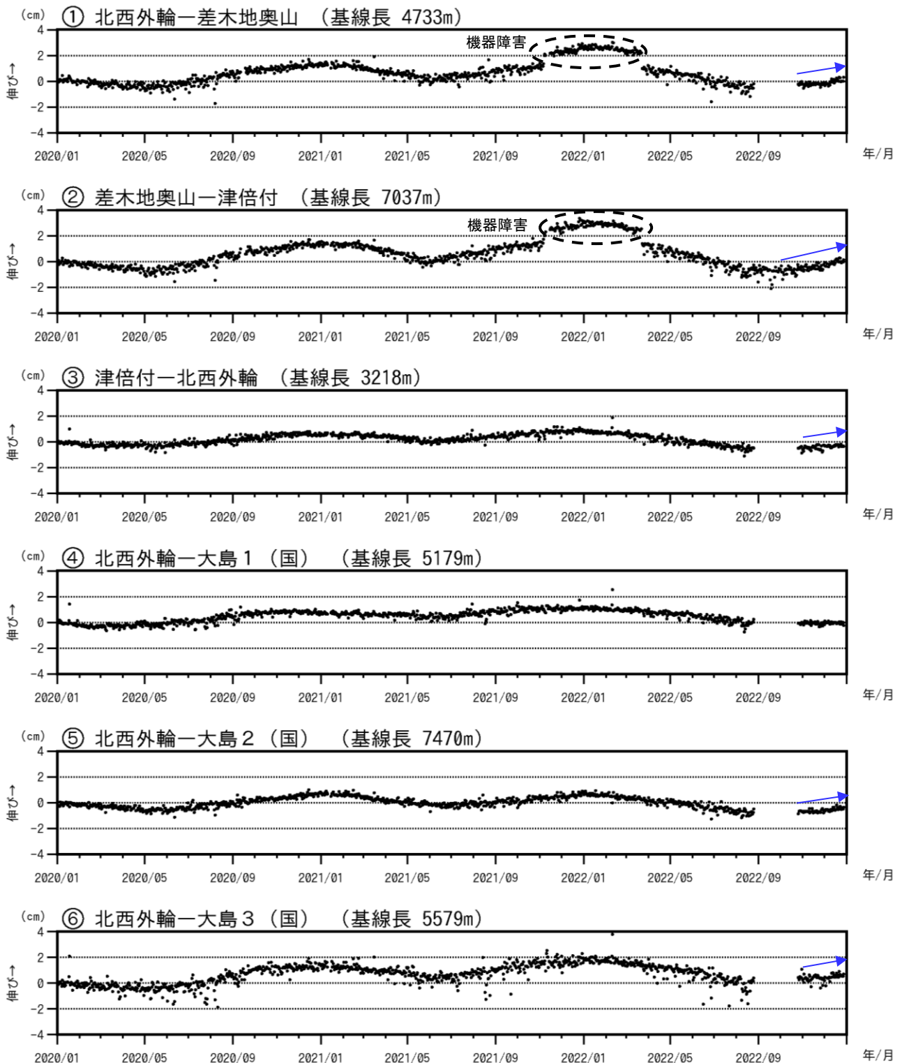
図3-2 伊豆大島 GNSS 連続観測による基線長変化(2020年1月～2022年12月31日)
