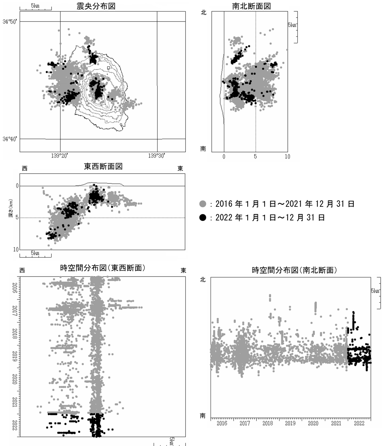
図4 伊豆大島 最近の火山性地震の震源分布(2016年1月1日～2022年12月31日)
