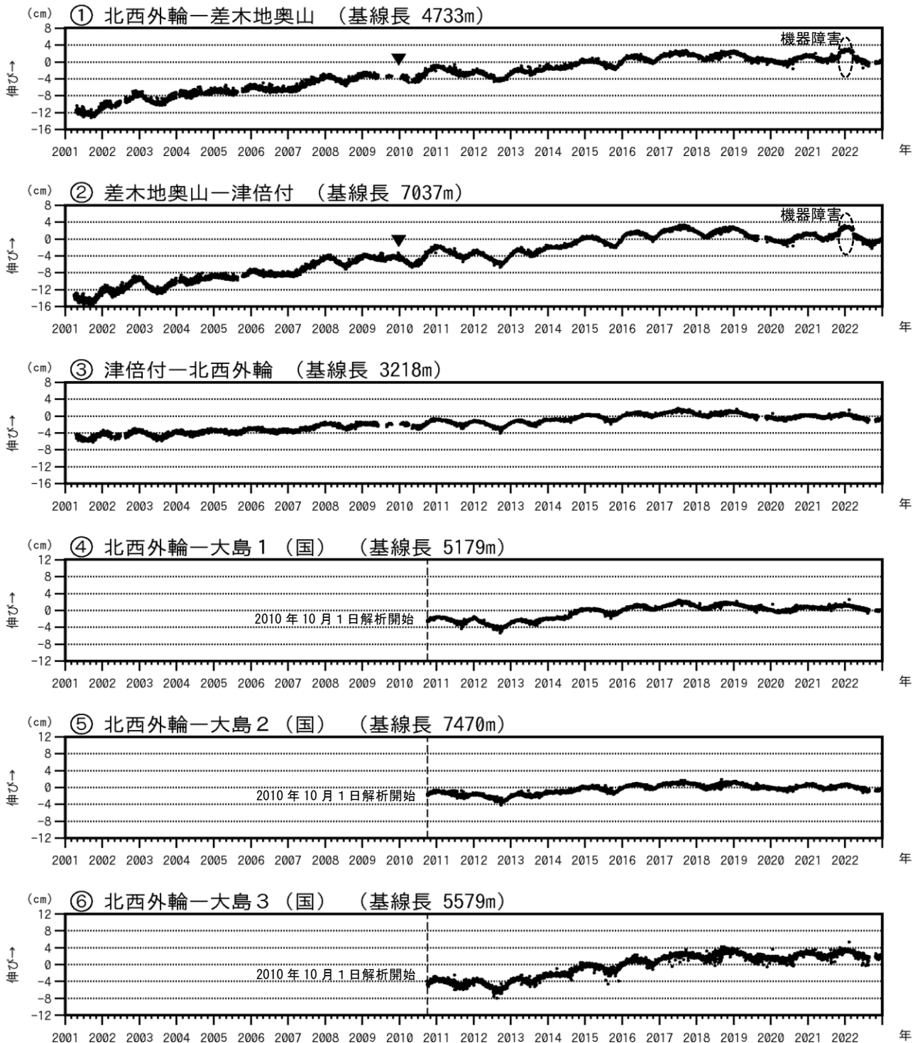
図3-1 伊豆大島 GNSS 連続観測による基線長変化(2001年1月～2022年12月31日)
