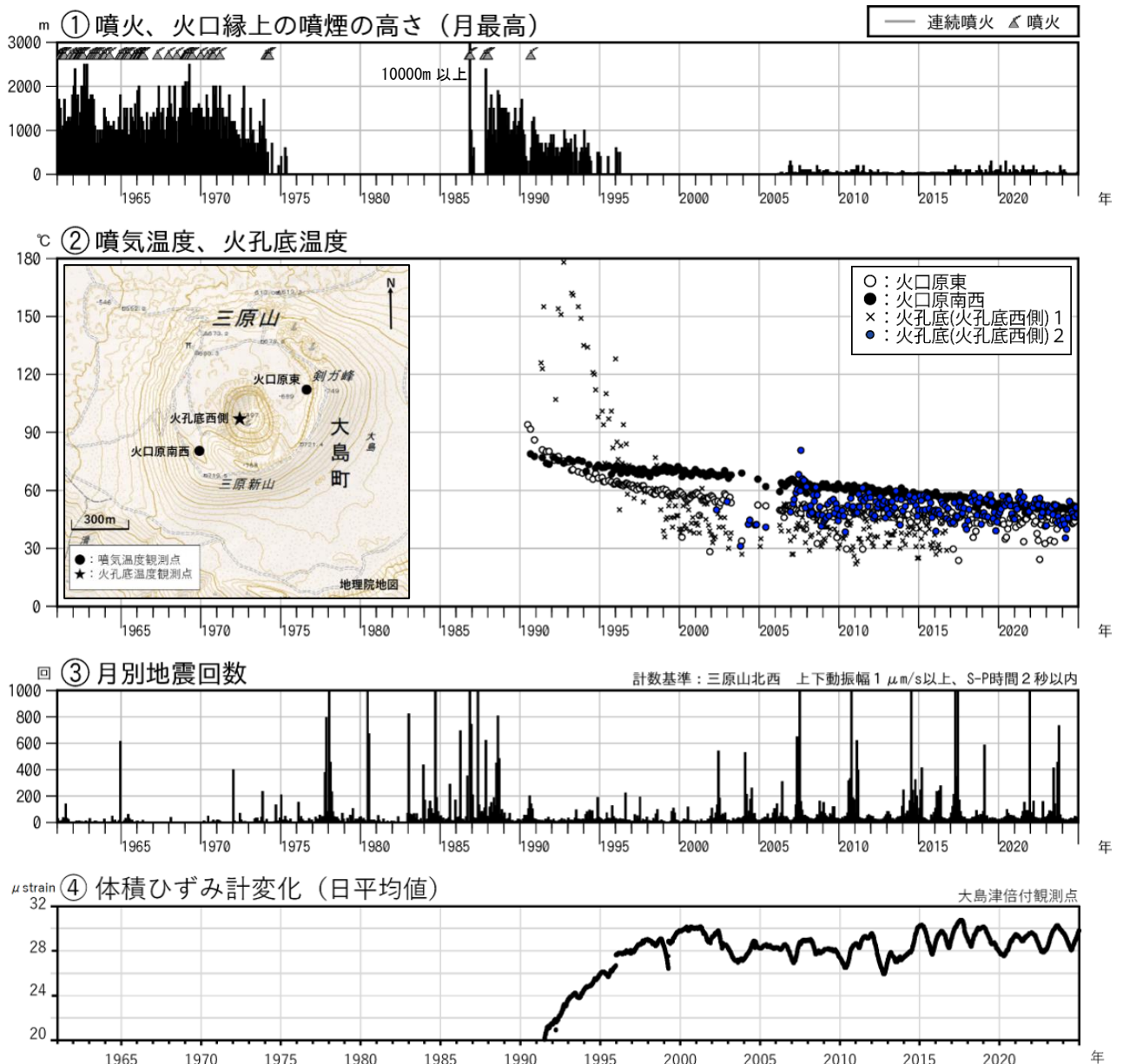
図 1 伊豆大島 長期間の火山活動経過図（1961 年 1 月～2024 年 12 月 31 日）
