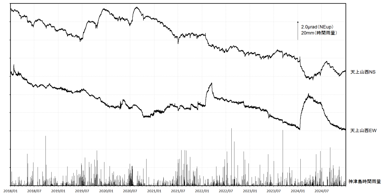
図4 神津島 天上山西観測点の傾斜変動（2018年1月1日～2024年12月31日） 地震等による一部のステップを除去しています。図中の空白部分は欠測を示します。
