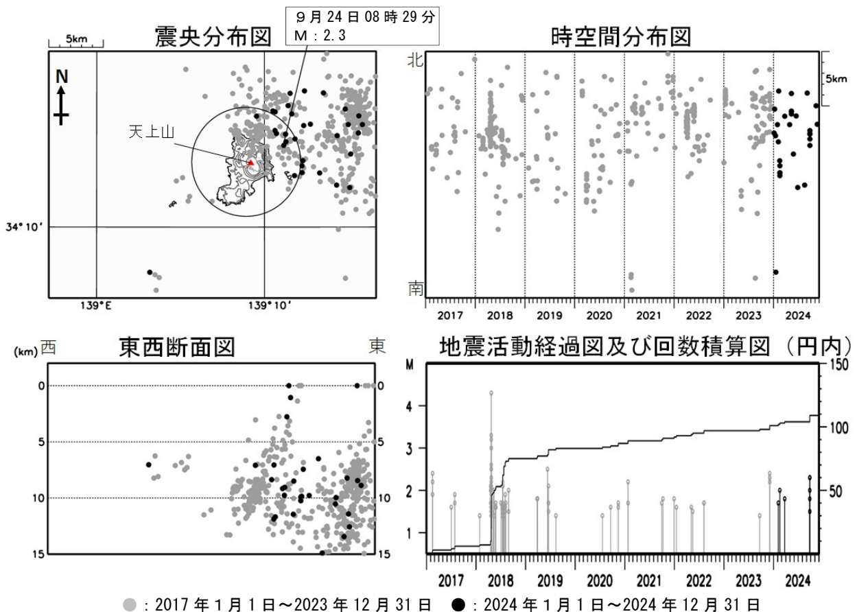
図3 神津島 広域地震観測網による山体・周辺の地震活動（2017年1月1日～2024年12月31日）
