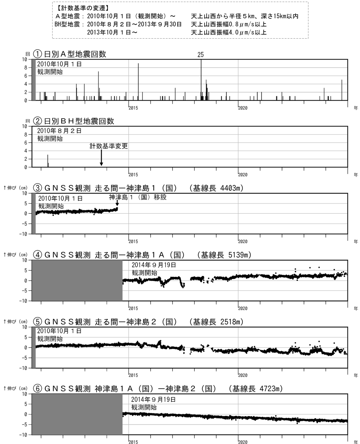
図2 神津島 火山活動経過図(2010年8月2日～2024年12月31日)
