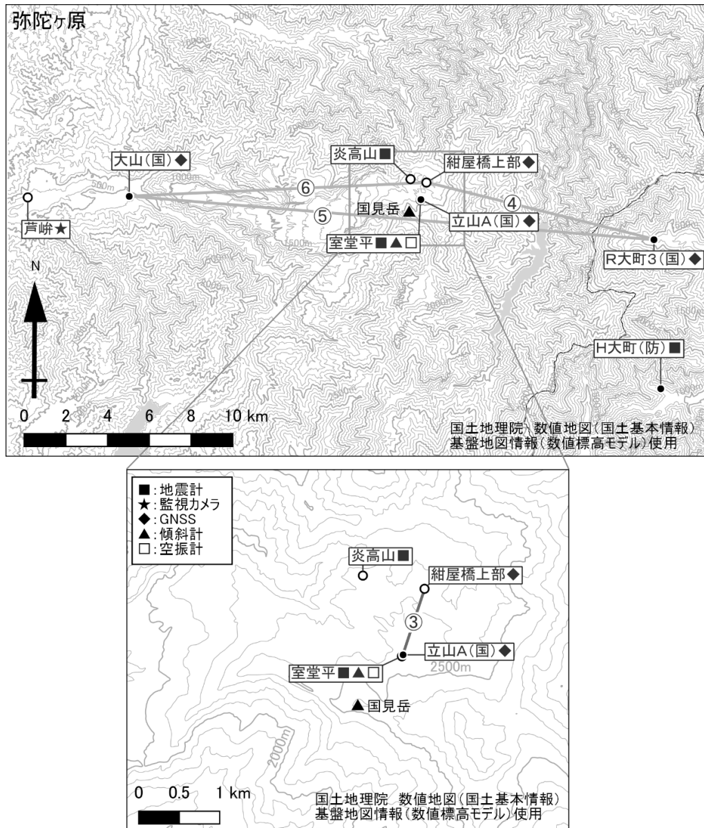
図5 弥陀ヶ原 観測点配置図
