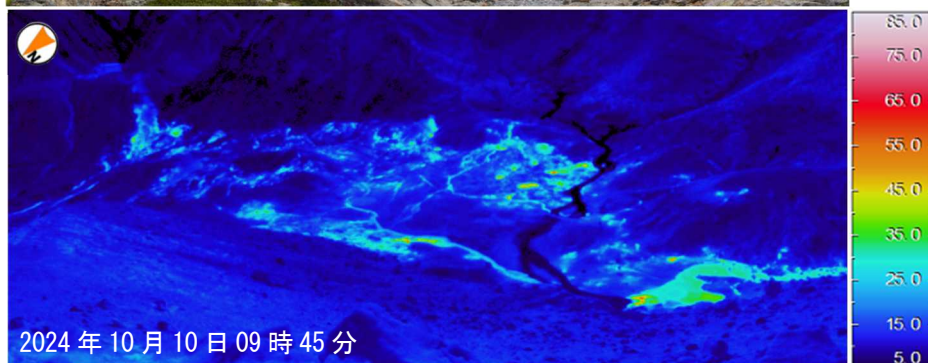
図4-3 弥陀ヶ原 地獄谷(鍛冶屋地獄及び百姓地獄)の状況(撮影位置及び撮影方向は図4-1参照) ・前年同月(2024年10月)の観測結果と比較して、高温領域の分布に目立った変化は認められませんでした。
