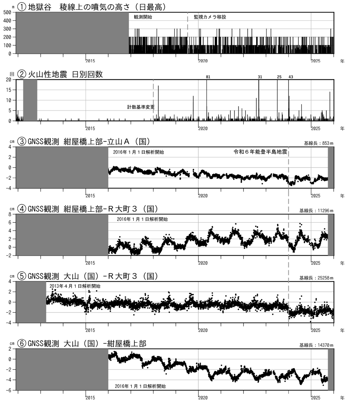
図3 弥陀ヶ原 火山活動経過図 (2011年12月1日~2025年12月31日)
