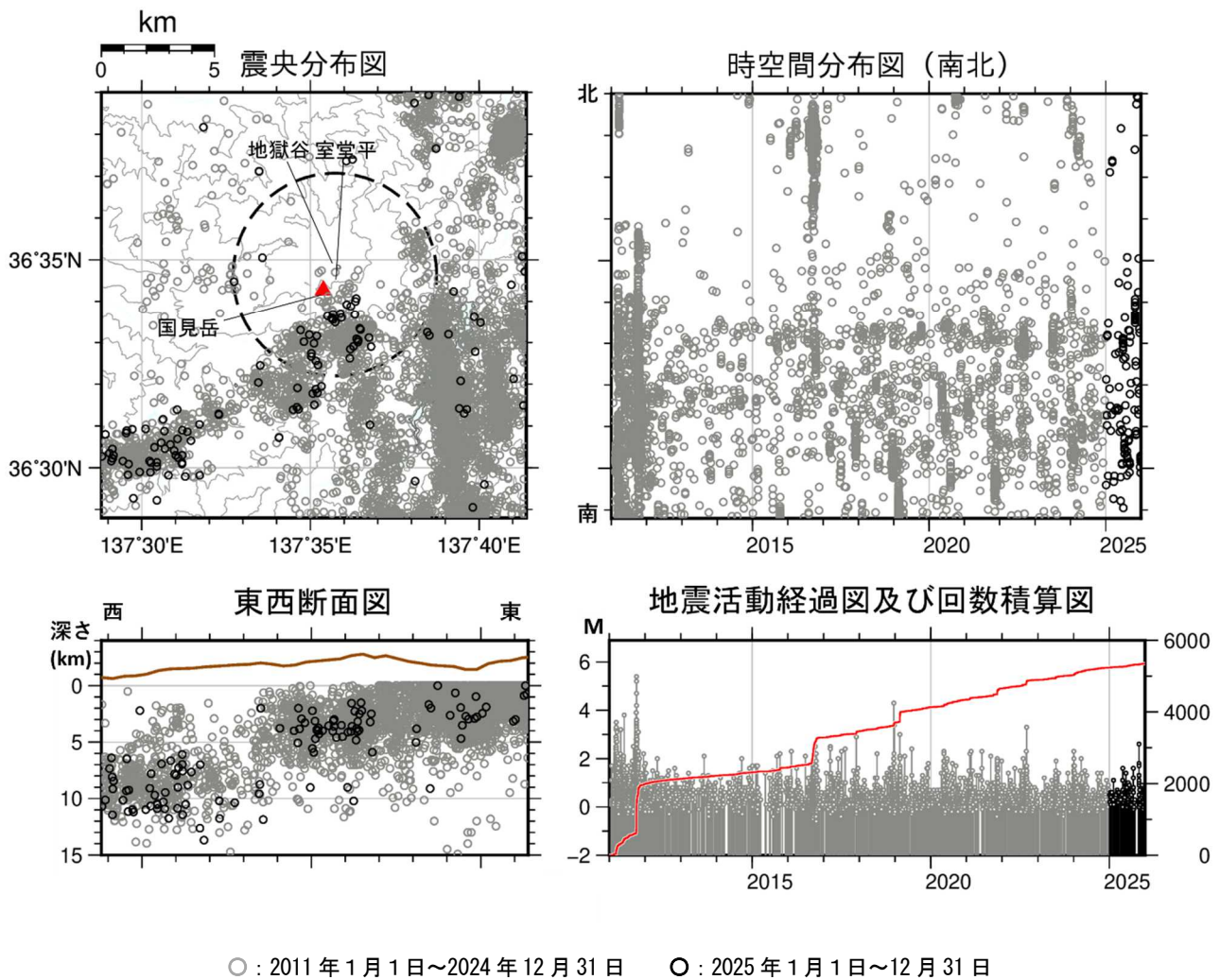
図2 弥陀ヶ原 広域地震観測網による山体・周辺の地震活動（2011年1月1日～2025年12月31日） 震央分布図中の円は弥陀ヶ原の計数対象地震（室堂平でS-P時間1秒以内）のおよその範囲を示しています。 広域地震観測網により震源決定したもので、深さは全て海面以下として決定しています。なお、2020年9月以降については、地震観測点の標高を考慮する等、震源決定の手法を変更しております。 図中の震源要素は一部暫定値が含まれており、後日変更することがあります。 M（マグニチュード）は地震の規模を表します。
