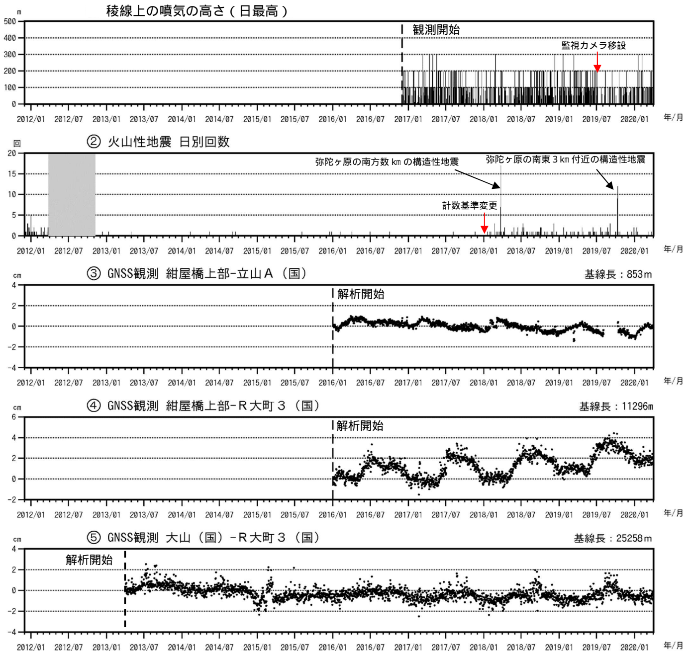
図3 弥陀ヶ原 火山活動経過図（2011年12月1日～2020年3月31日）
