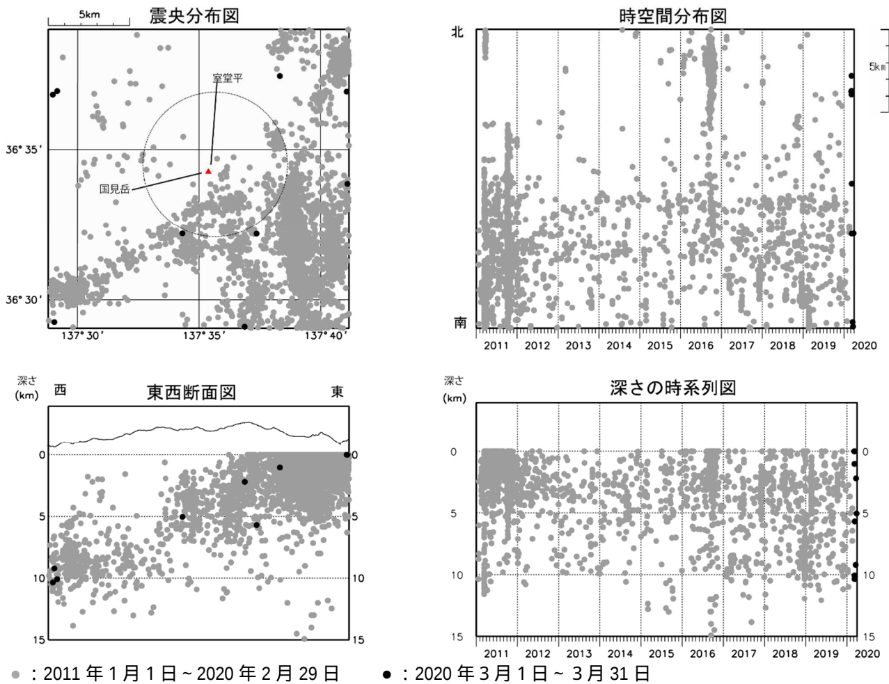
図2 弥陀ヶ原 広域地震観測網による山体・周辺の地震活動（2011年1月1日～2020年3月31日）
