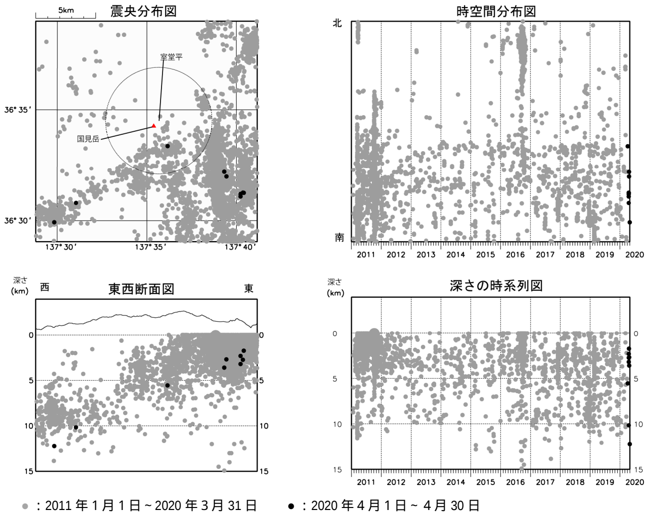
図2 弥陀ヶ原 広域地震観測網による山体・周辺の地震活動（2011年1月1日～2020年4月30日）
