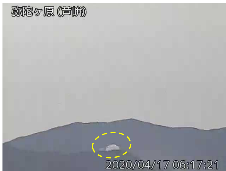
図1 弥陀ヶ原 地獄谷からの噴気の状況（黄丸）（4月17日、芦峯監視カメラによる）
