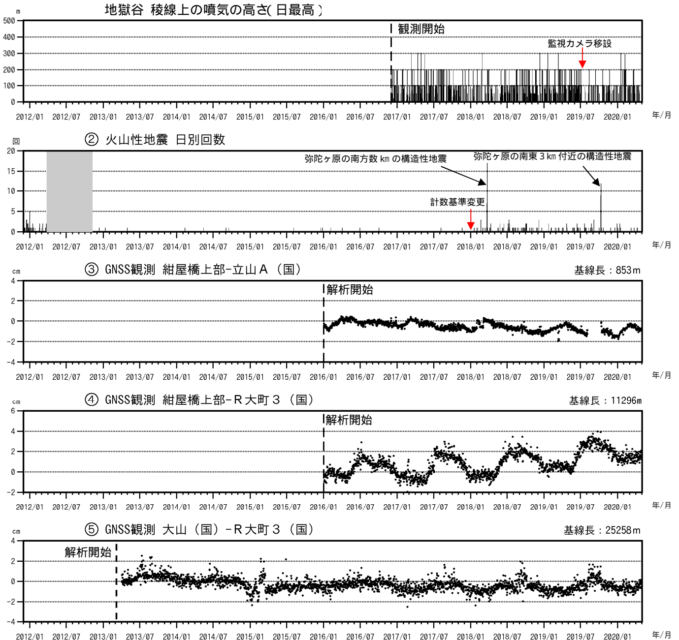
図3 弥陀ヶ原 火山活動経過図（2011年12月1日～2020年4月30日）
