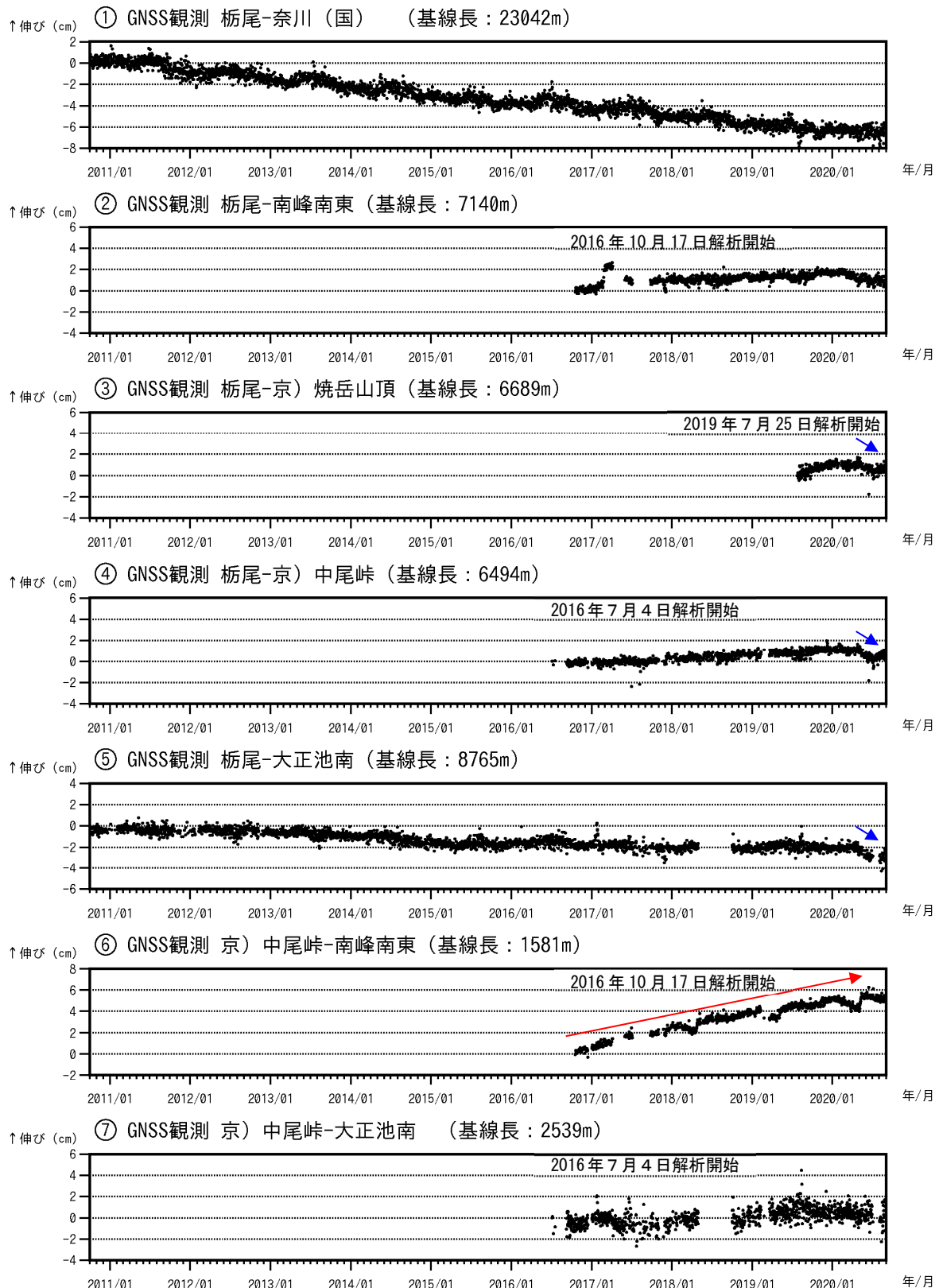
図7 焼岳 GNSS連続観測による基線長変化（2010年10月1日～2020年8月31日）
