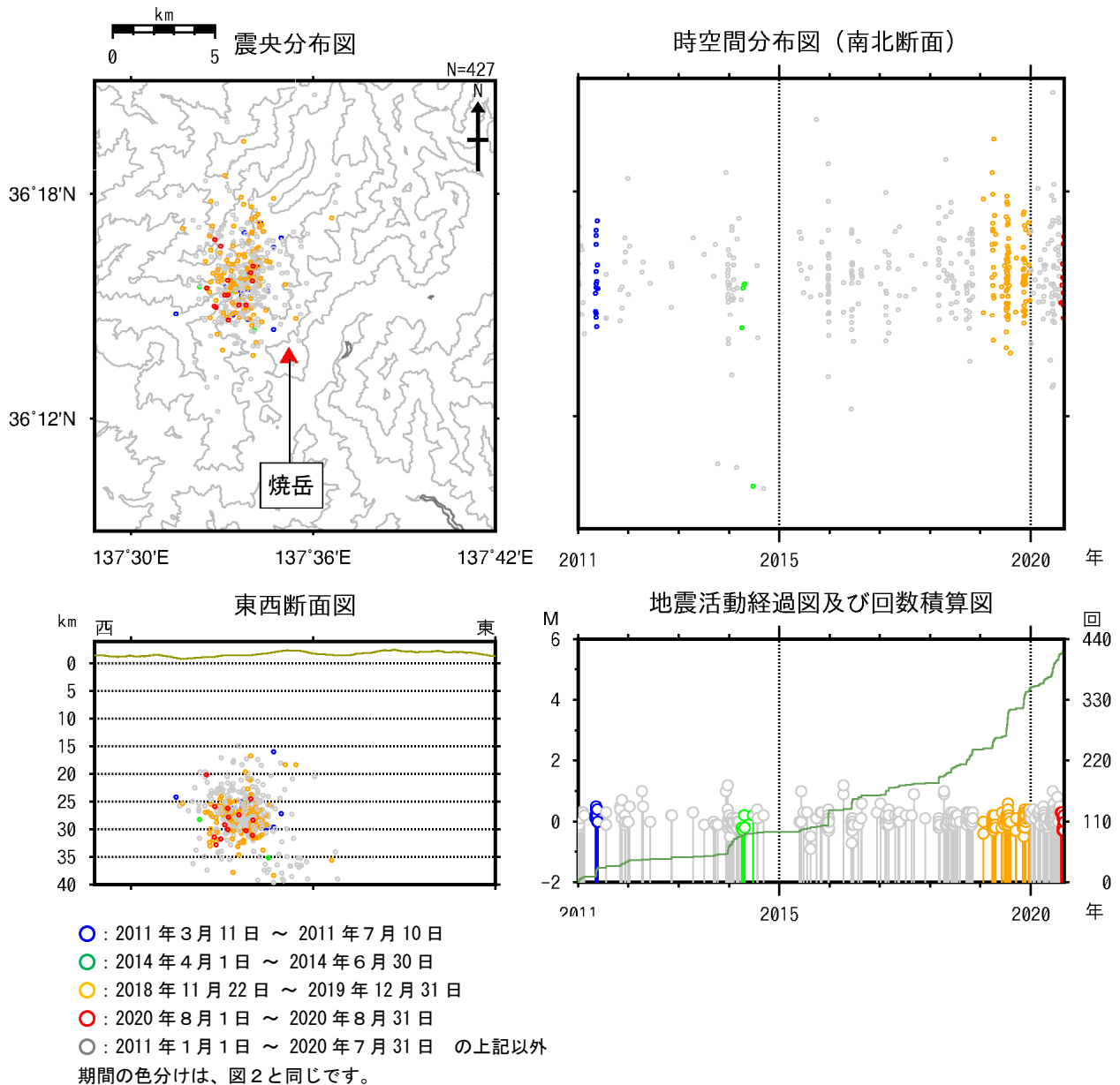
図3 焼岳 深部低周波地震の震源分布図（広域地震観測網による）（2011年1月1日～2020年8月31日）
