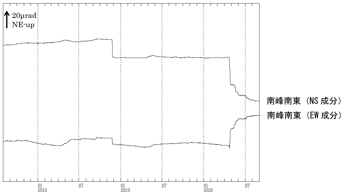
図9 焼岳 南峰南東観測点における傾斜データ（2017年8月1日～2020年8月31日）
