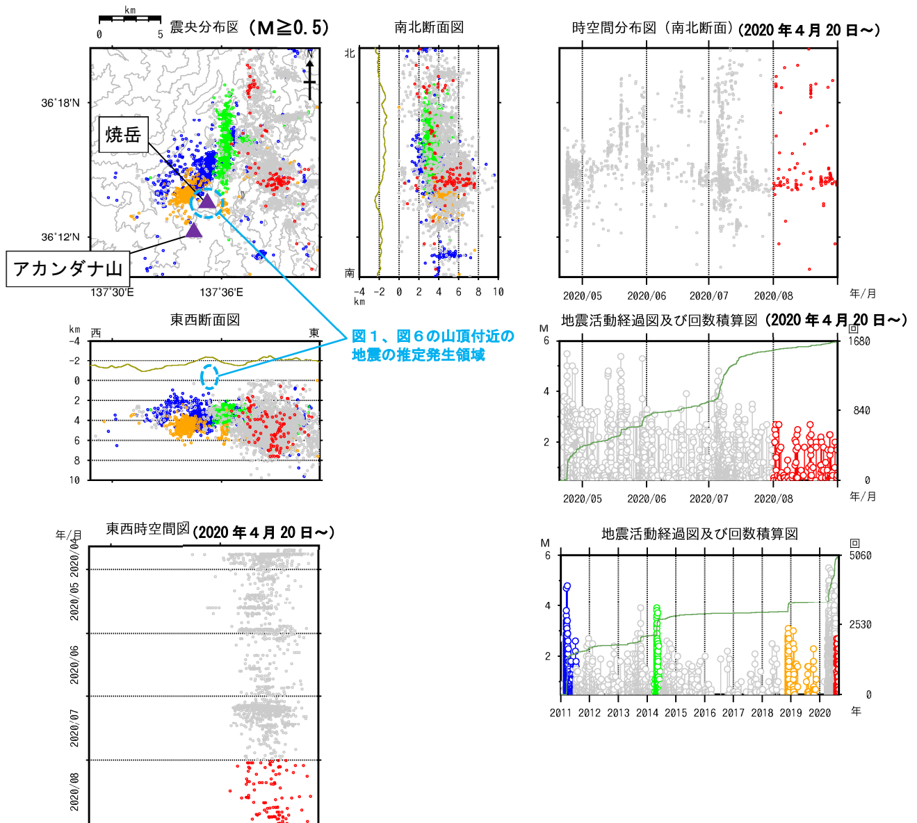
図2 焼岳 広域地震観測網による山体及び周辺の地震活動(2011年1月1日～2020年8月31日)
