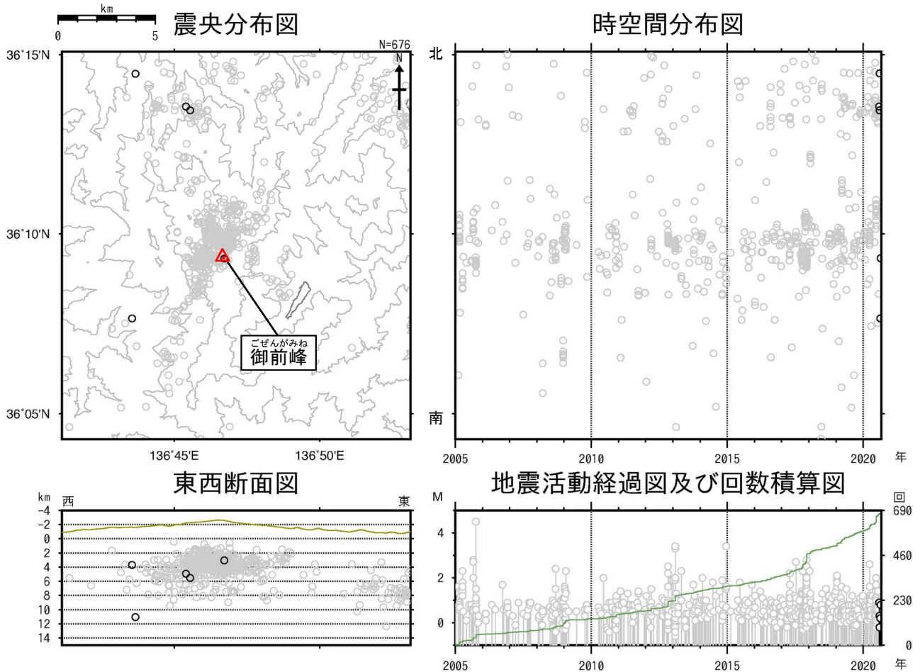
図4 白山 広域地震観測網による山体・周辺の地震活動（2005年1月1日～2020年8月31日）
