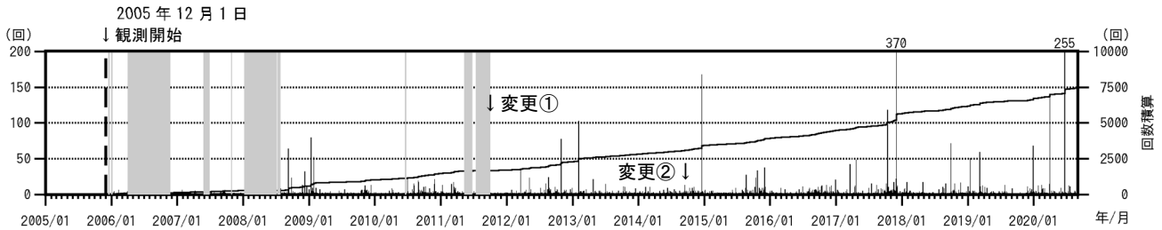
図3 白山 日別地震回数と積算回数（2005年12月1日～2020年8月31日）
