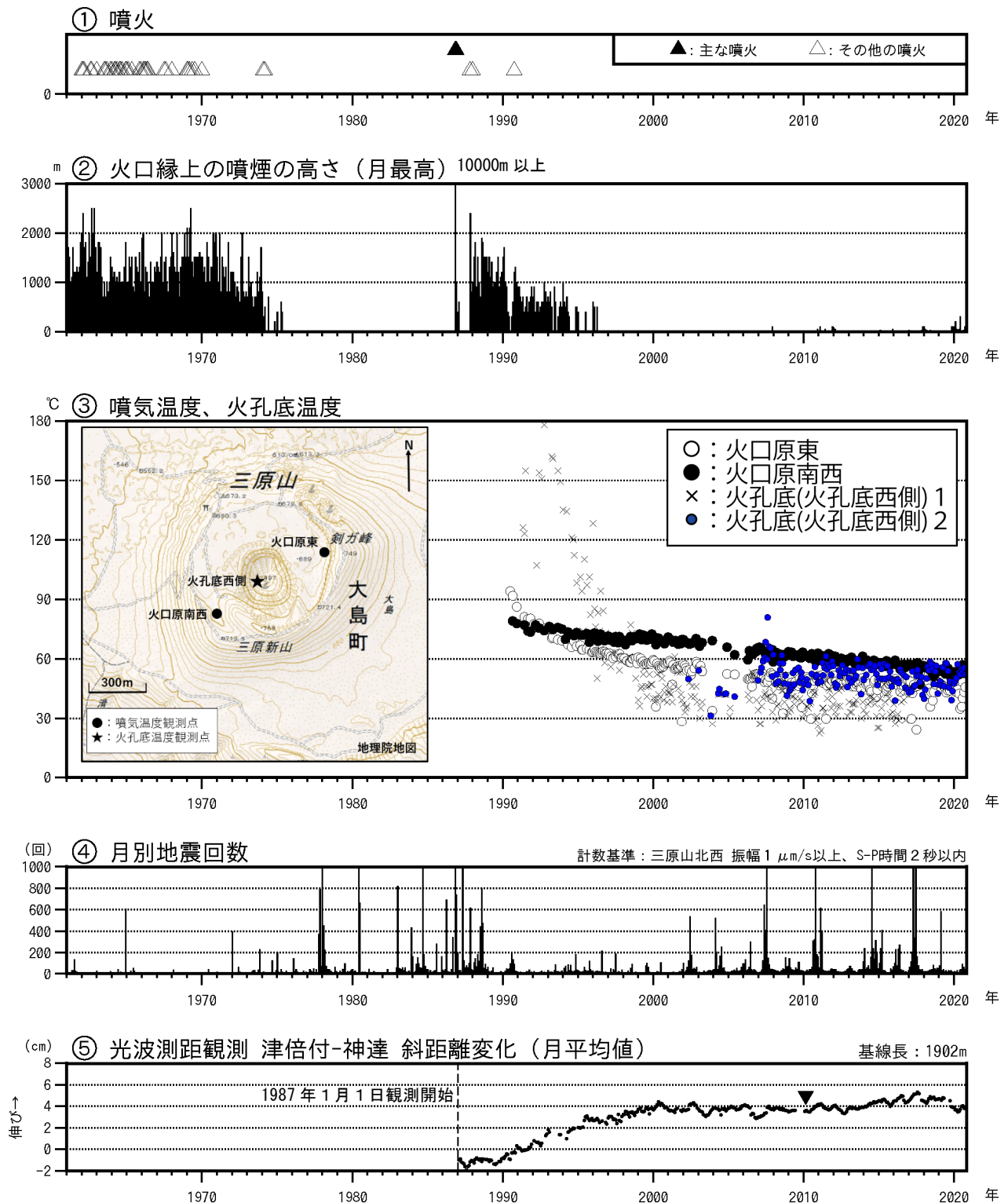
図1 伊豆大島 長期間の火山活動経過図（1961年1月～2020年10月31日）
