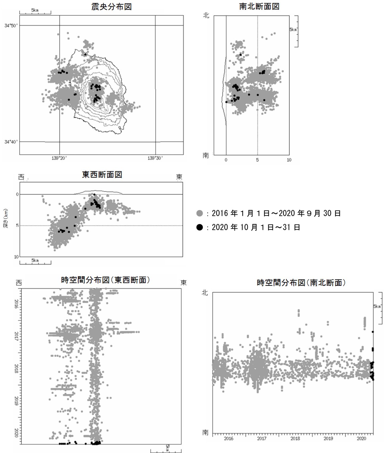
図4 伊豆大島 震源分布図（2016 年 1 月 1 日～2020 年 10 月 31 日）
