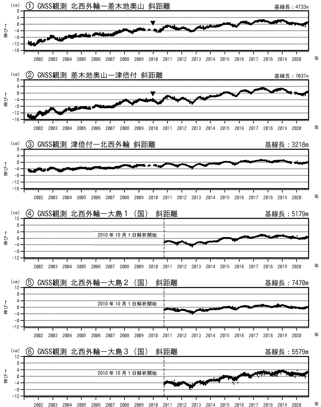
図3-1 伊豆大島 GNSS連続観測による基線長変化(2001年1月～2020年10月31日)
