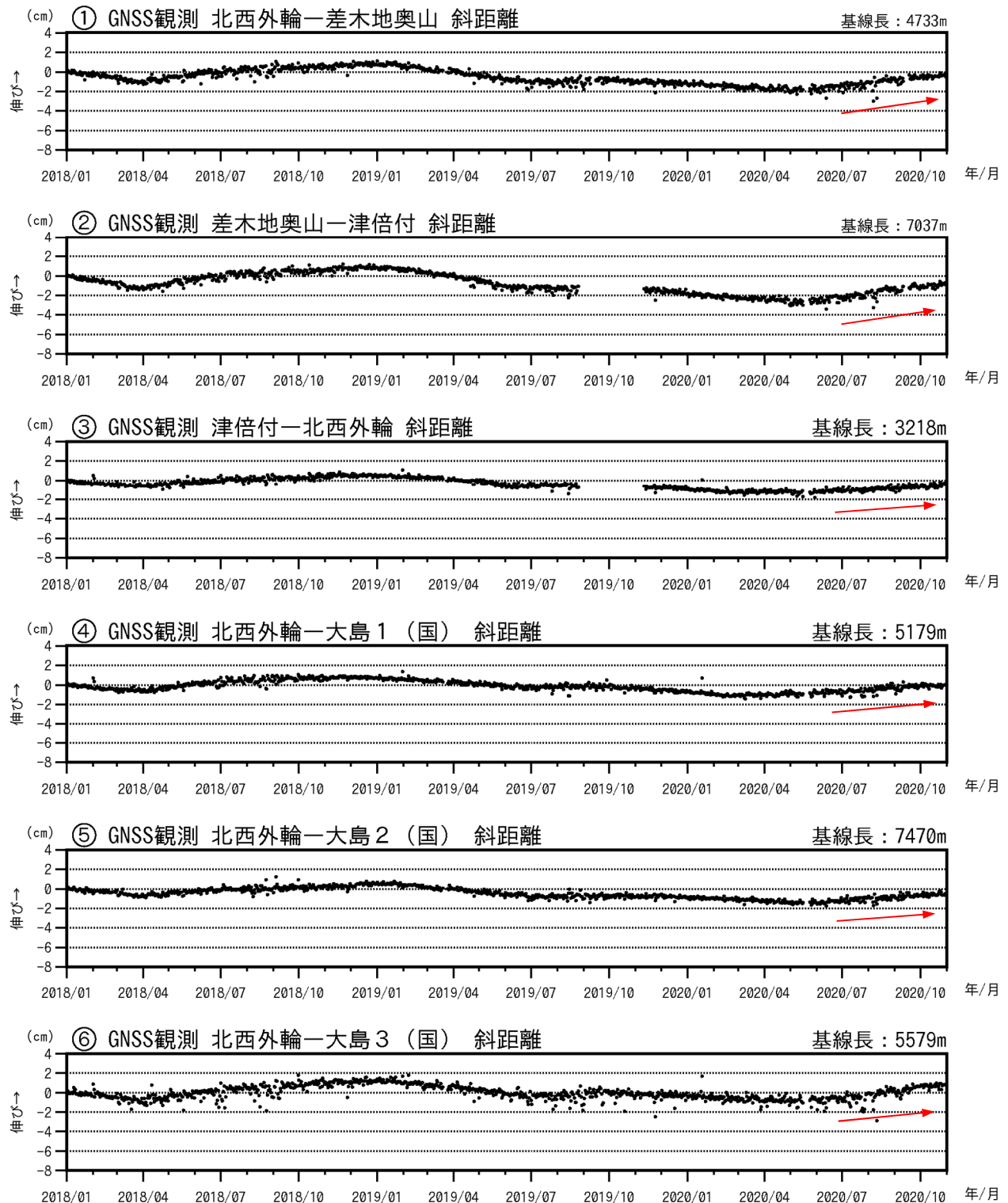
図3-2 伊豆大島 GNSS連続観測による基線長変化(2018年1月～2020年10月31日)
