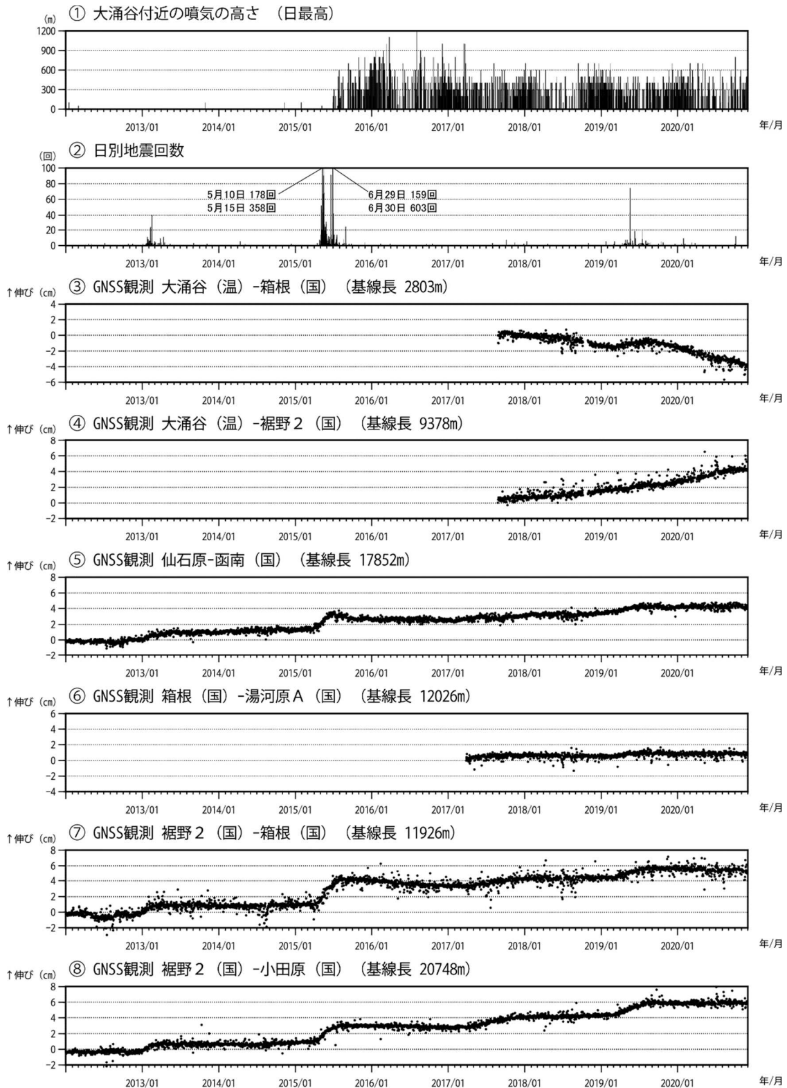
図6 箱根山 火山活動経過図（2012年1月1日～2020年11月30日）
