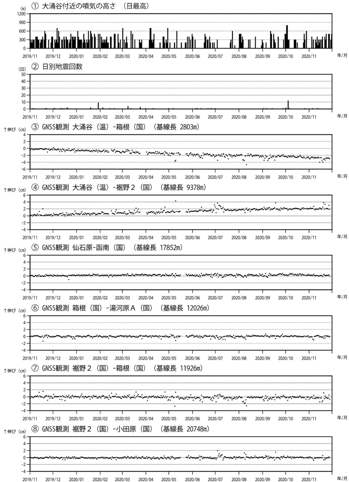
図7 箱根山 火山活動経過図（2019年11月1日～2020年11月30日）
