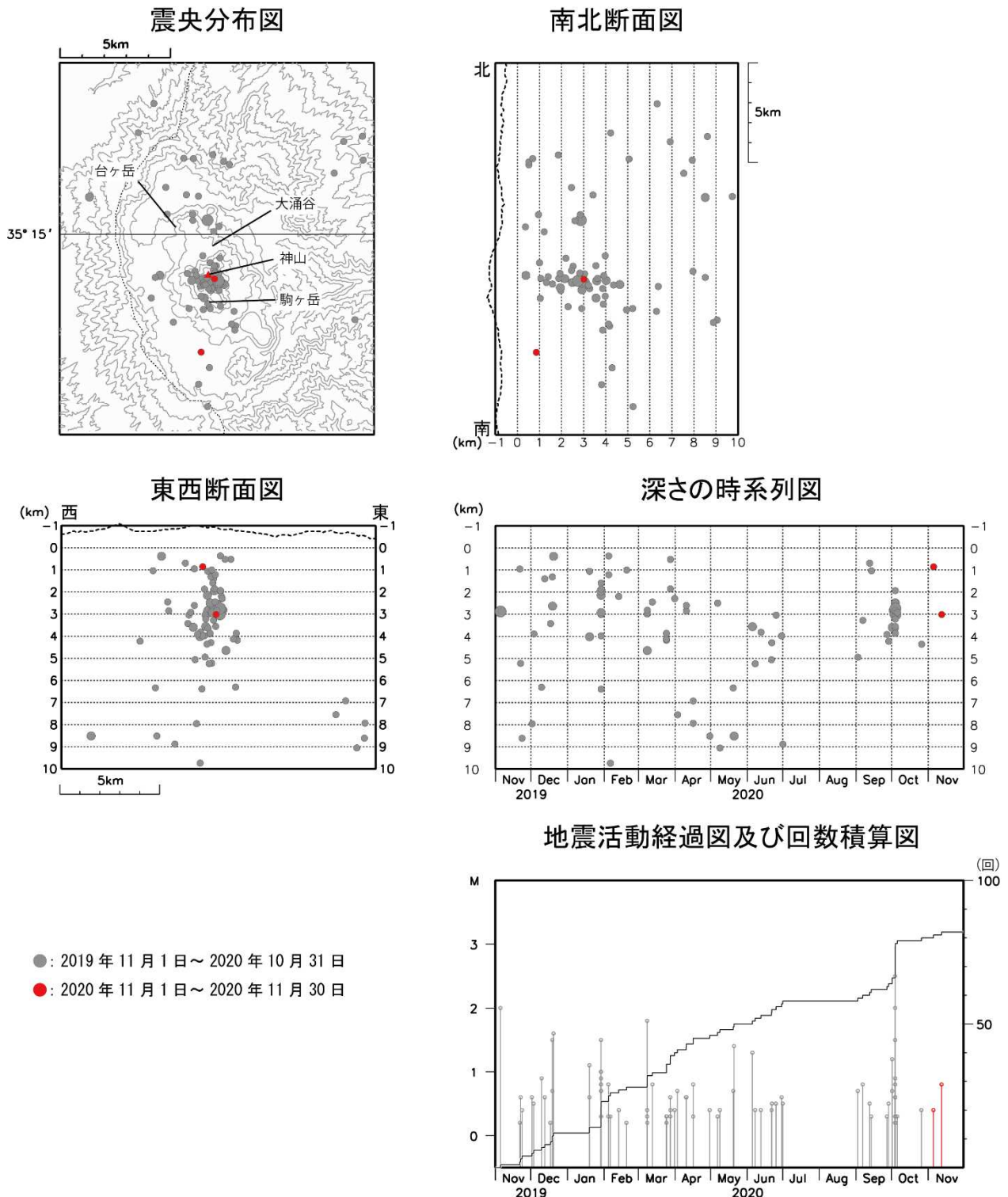
図8 箱根山 広域地震観測網による山体周辺の震源分布図（2019年11月1日～2020年11月30日）
