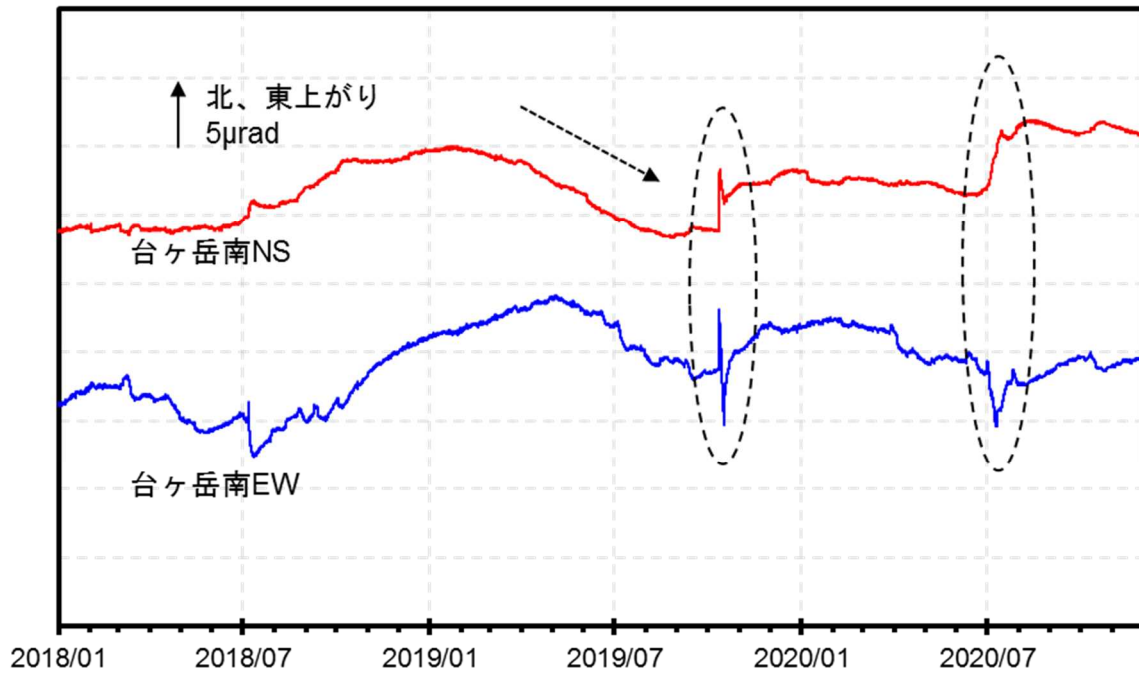
図9 箱根山 台ヶ岳南観測点における傾斜データ（2018年1月1日～2020年11月30日）
