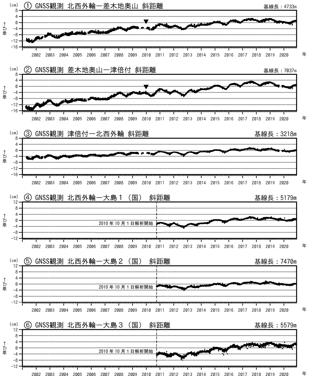
図3-1 伊豆大島 GNSS連続観測による基線長変化(2001年1月～2020年11月30日)
