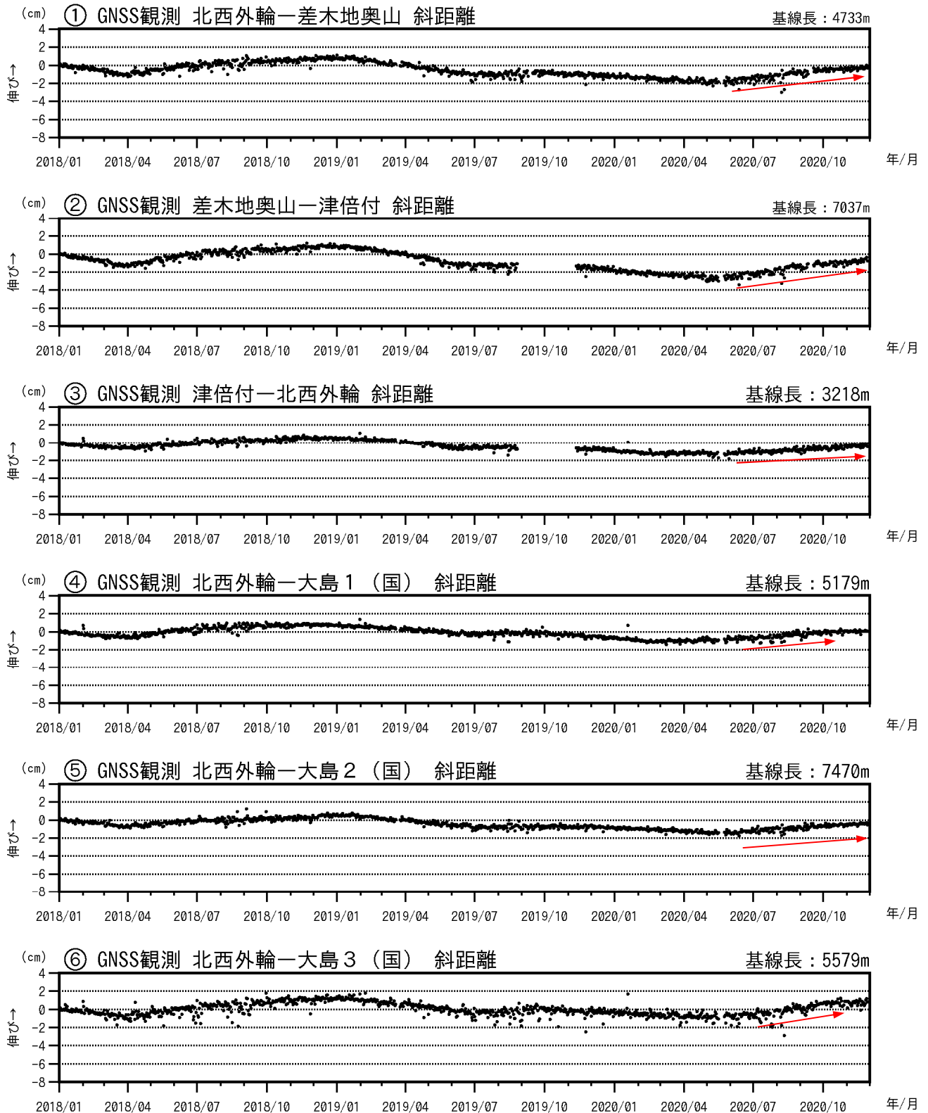
図3-2 伊豆大島 GNSS連続観測による基線長変化(2018年1月~2020年11月30日)
