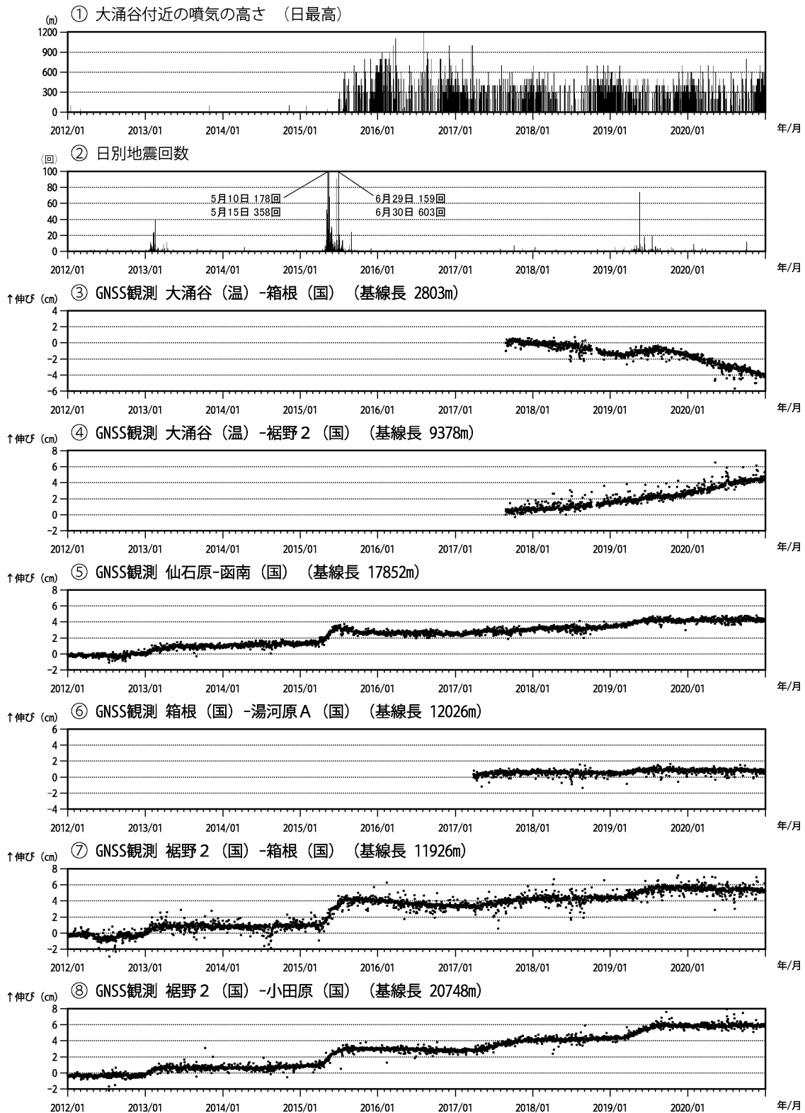
図6 箱根山 火山活動経過図（2012年1月1日～2020年12月31日）
