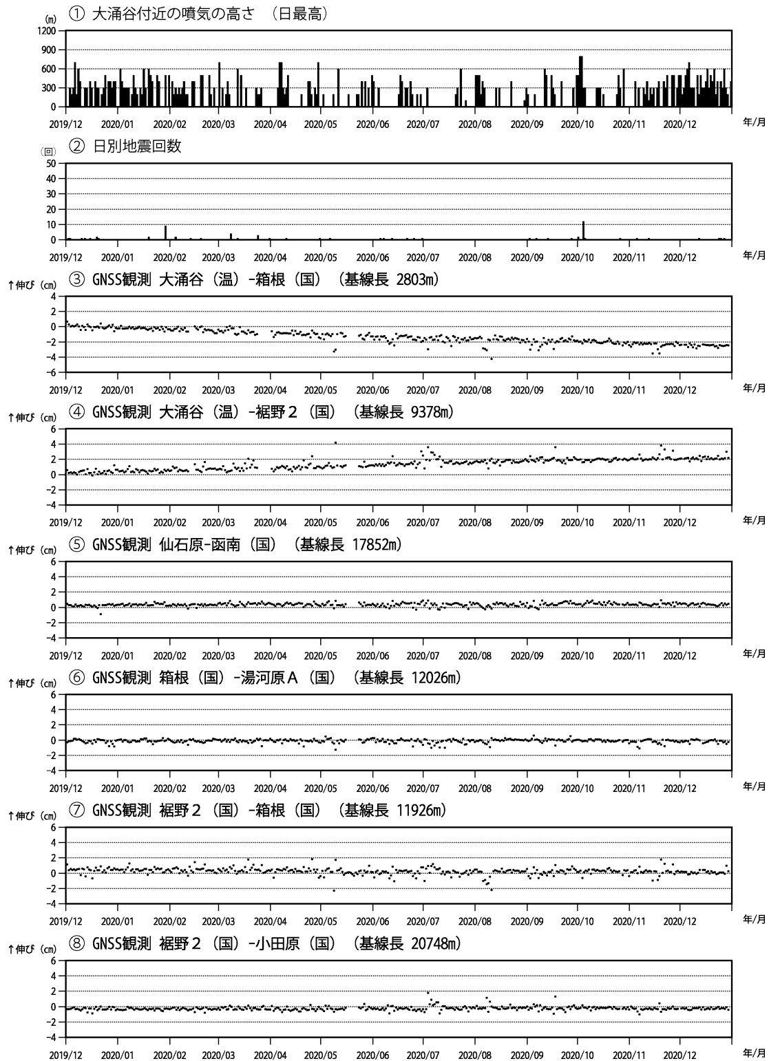
図7 箱根山 火山活動経過図（2019年12月1日～2020年12月31日）
