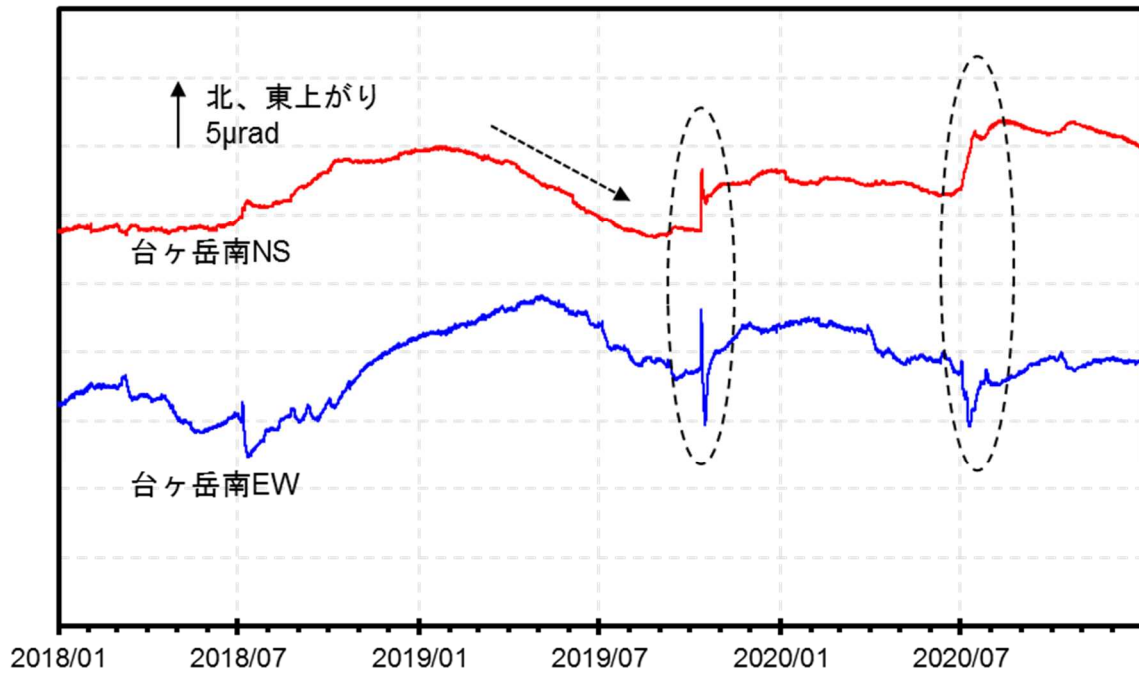
図9 箱根山 台ヶ岳南観測点における傾斜データ（2018年1月1日～2020年12月31日）
