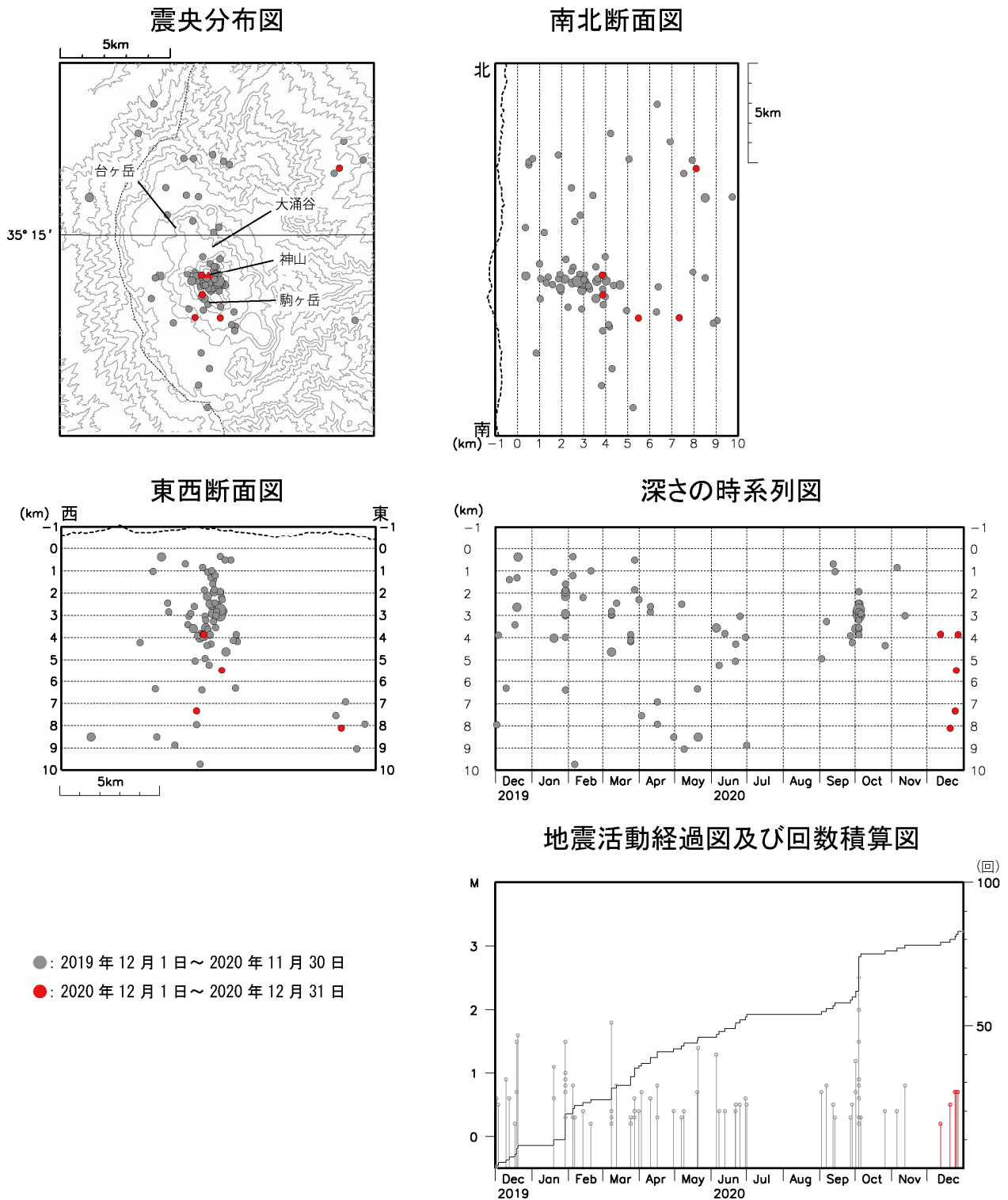
図8 箱根山 広域地震観測網による山体周辺の震源分布図（2019年12月1日～2020年12月31日）
