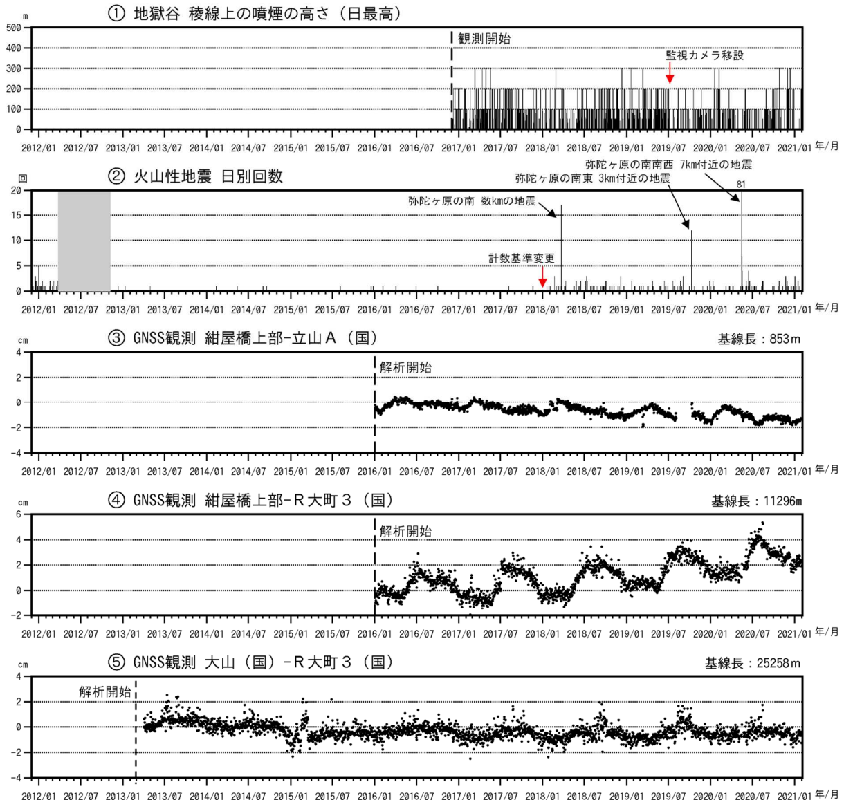
図3 弥陀ヶ原 火山活動経過図（2011年12月1日～2021年1月31日）
