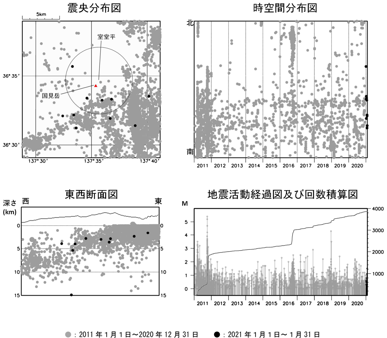
図2 弥陀ヶ原 広域地震観測網による山体・周辺の地震活動（2011年1月1日～2021年1月31日） 震央分布図中の円は弥陀ヶ原の計数対象地震（室堂平でS-P時間1秒以内）のおよその範囲を示しています。 広域地震観測網により震源決定したもので、深さは全て海面以下として決定しています。 図中の震源要素は一部暫定値が含まれており、後日変更することがあります。 この図では、関係機関の地震波形を一元的に処理し、地震観測点の標高を考慮する等した新手法で得られた震源を用いています（ただし、2020年8月以前の地震については火山活動評価のための参考震源です）。 2021年2月8日現在、2020年4月18日から10月23日まで、及び2021年1月9日以降の地震について、暫定的に震源精査の基準を変更しているため、その前後の期間と比較して微小な地震での震源決定数の変化（増減）が見られます。
