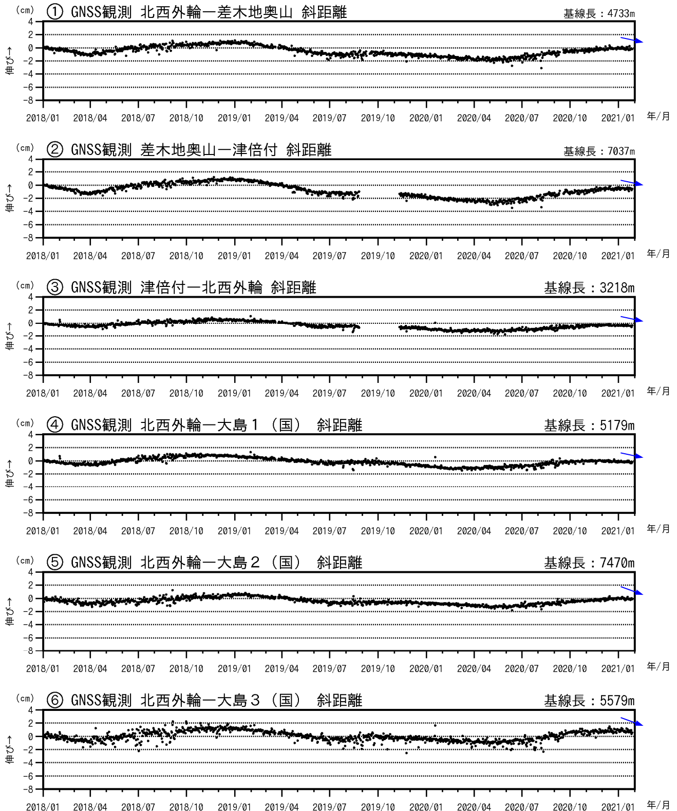
図3-2 伊豆大島 GNSS連続観測による基線長変化(2018年1月～2021年1月31日)
