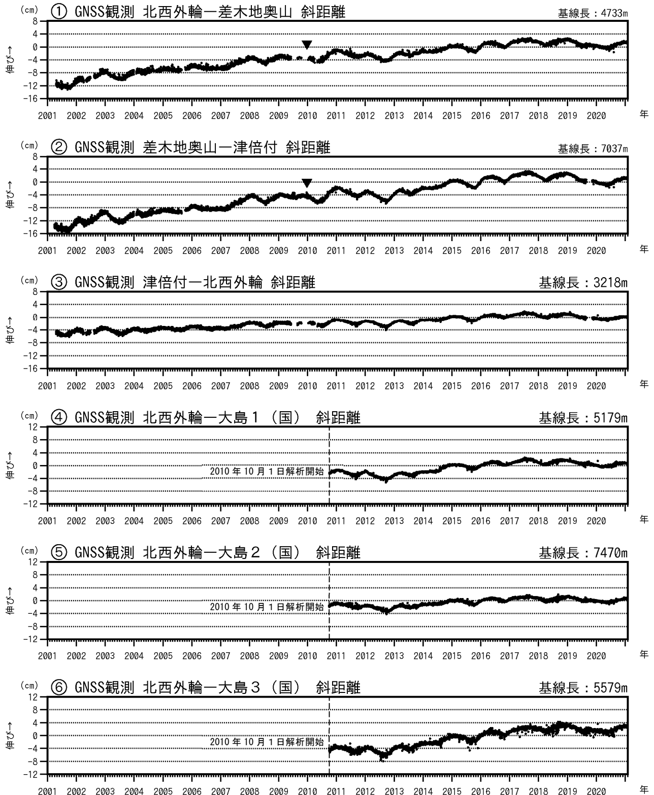
図3-1 伊豆大島 GNSS 連続観測による基線長変化(2001年1月～2021年1月31日)
