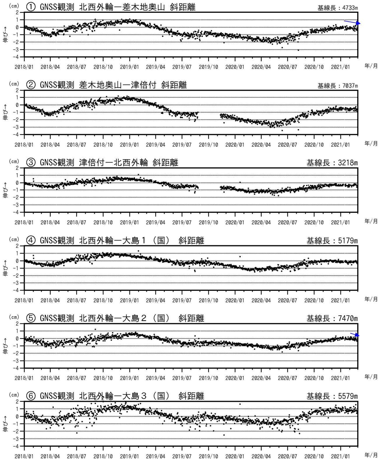
図3-2 伊豆大島 GNSS連続観測による基線長変化(2018年1月～2021年2月28日)
