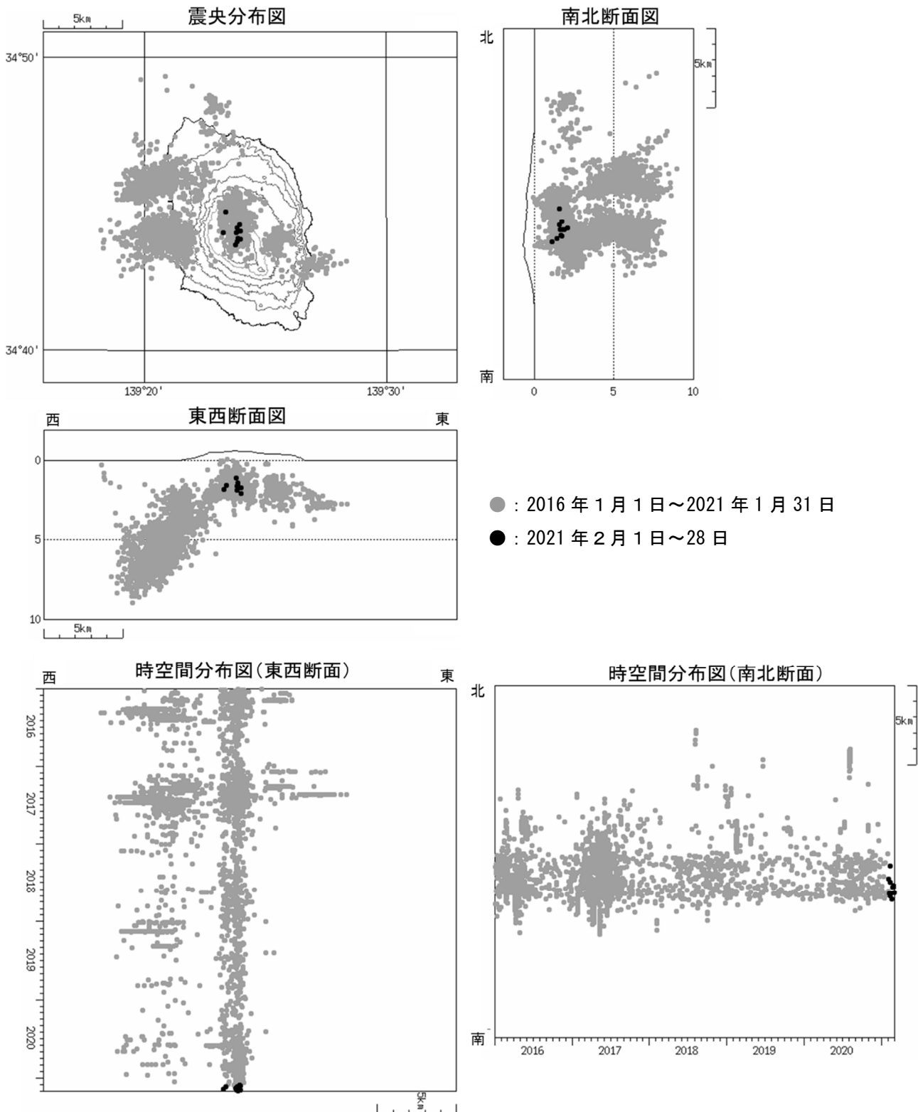
図4 伊豆大島 震源分布図（2016 年 1 月 1 日～2021 年 2 月 28 日） ・長期的には、地震活動は活発な時期と静穏な時期を繰り返しています。 ・今期間、震源はカルデラ内の深さ 1 ～ 2 km 付近に分布しました。
