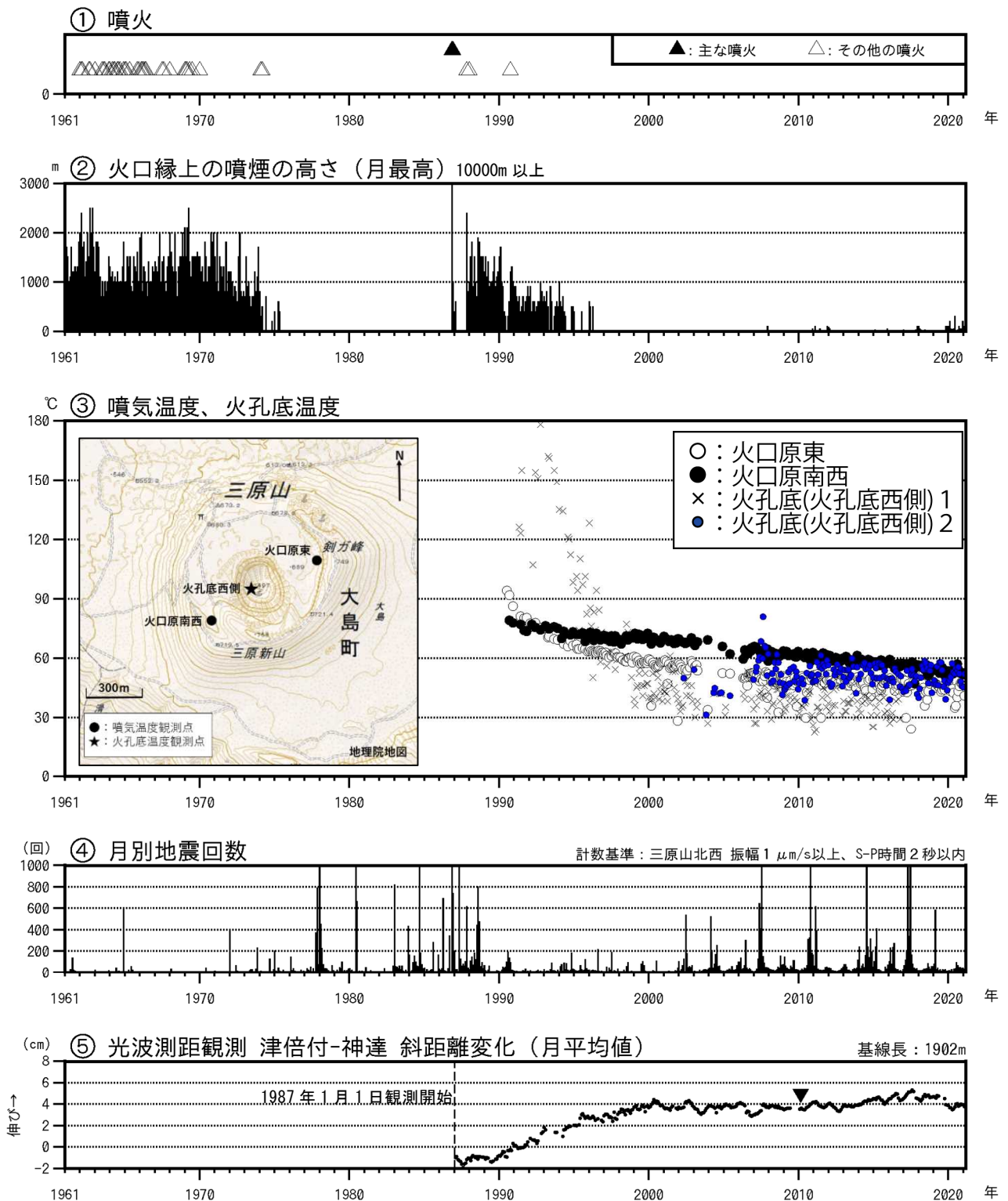
図1 伊豆大島 長期間の火山活動経過図（1961年1月～2021年2月28日）
