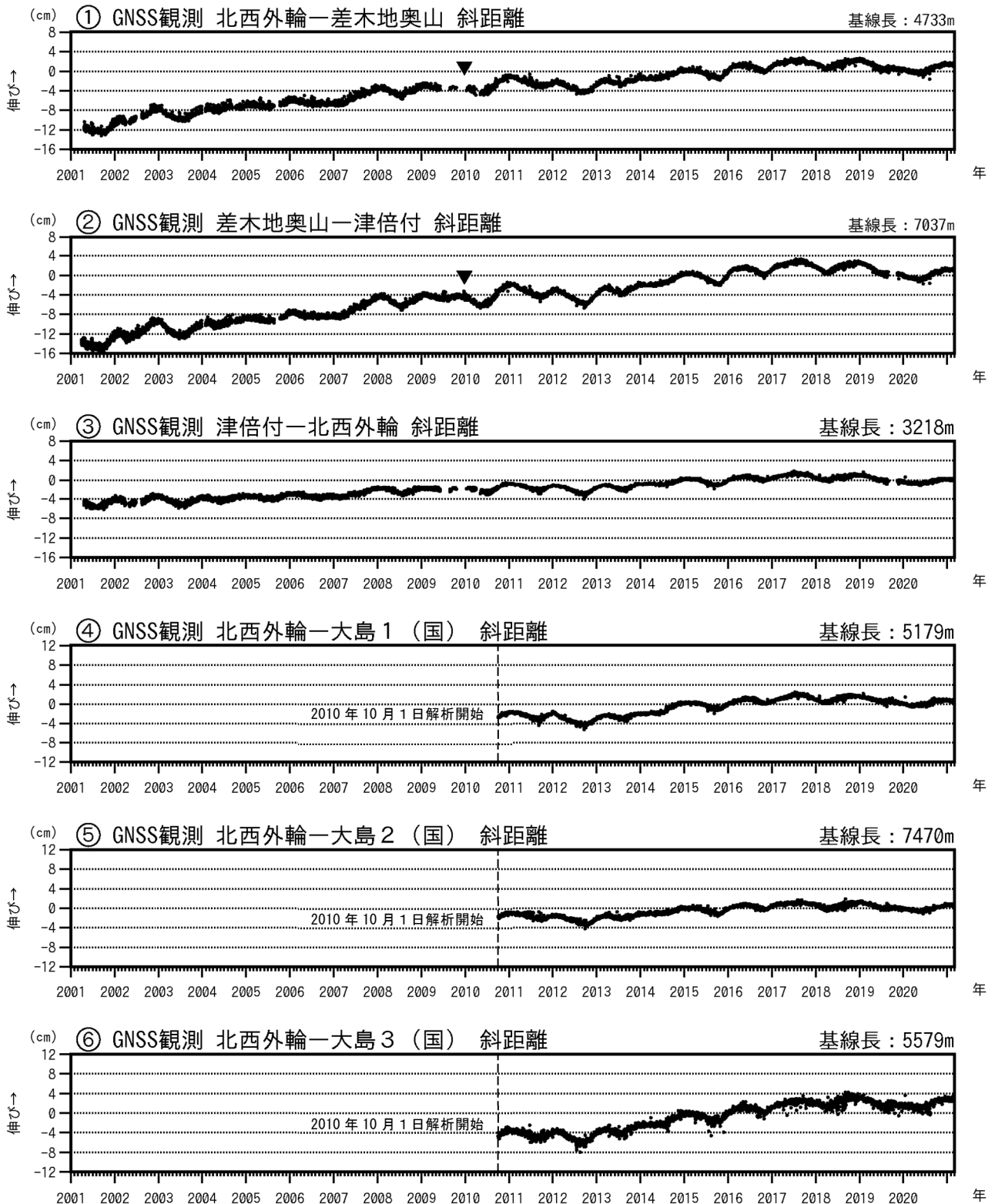
図3-1 伊豆大島 GNSS 連続観測による基線長変化(2001年1月～2021年2月28日)
