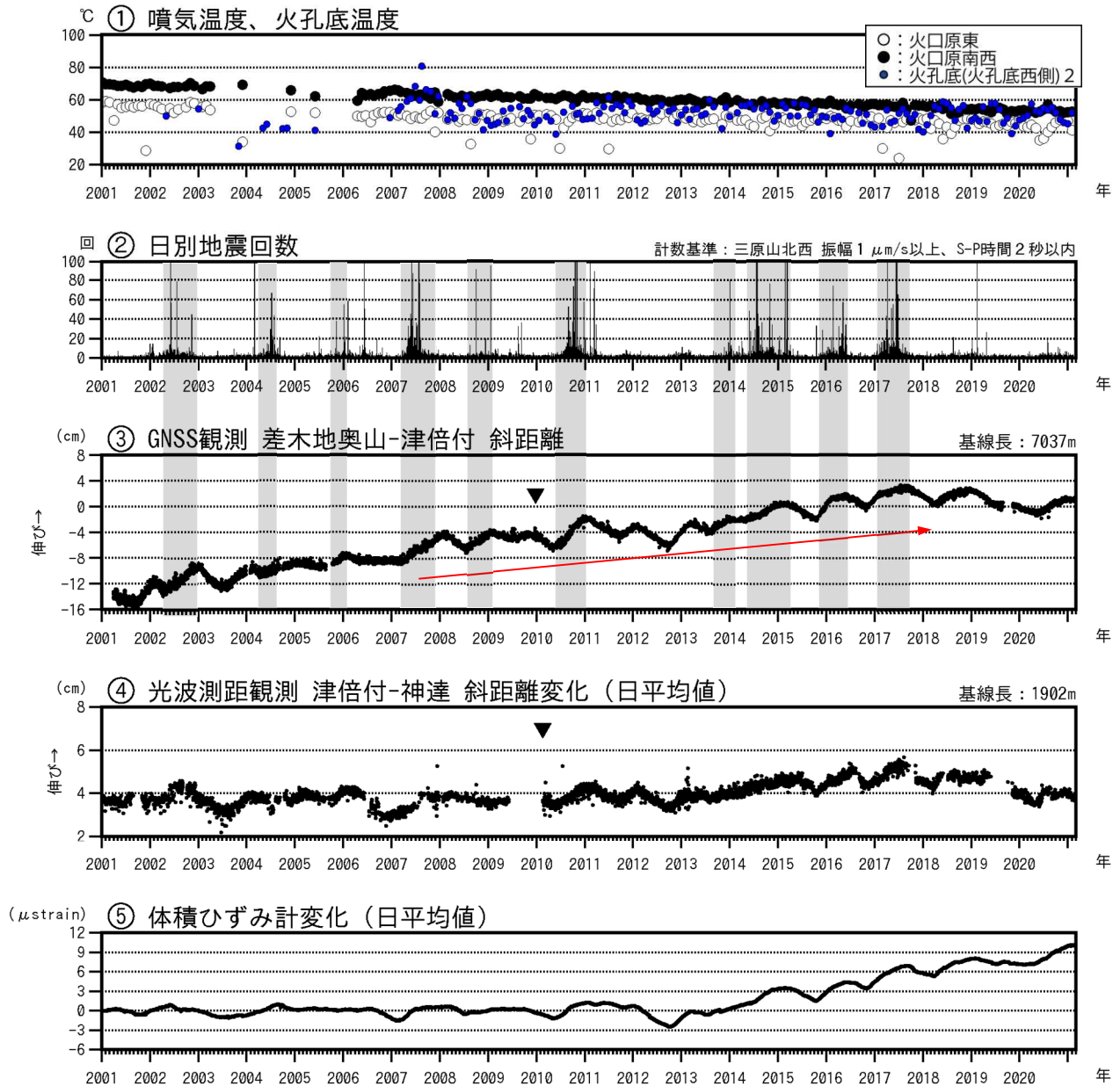
図2 伊豆大島 最近の火山活動経過図（2001年1月～2021年2月28日）
