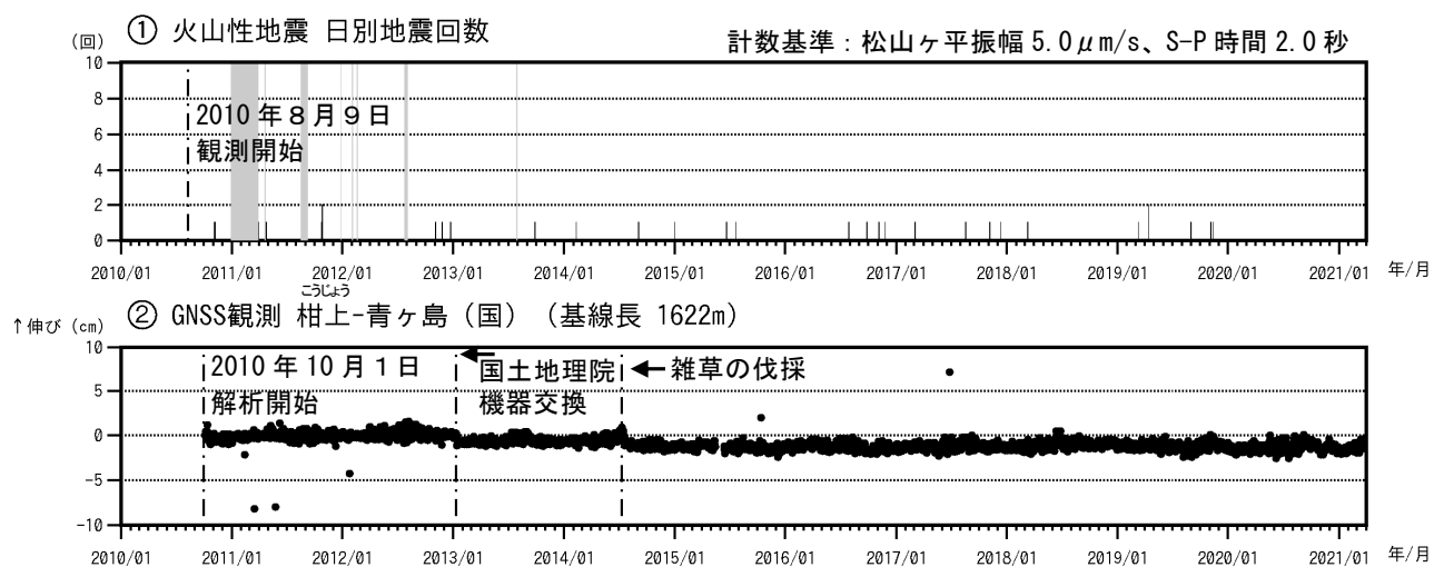
図3 青ヶ島 火山活動経過図（2010年8月9日～2021年3月31日） ① グラフの灰色部分は機器障害による欠測を示す。 ② (国)：国土地理院、図4のGNSS基線②に対応。グラフの空白部分は欠測を示す。
