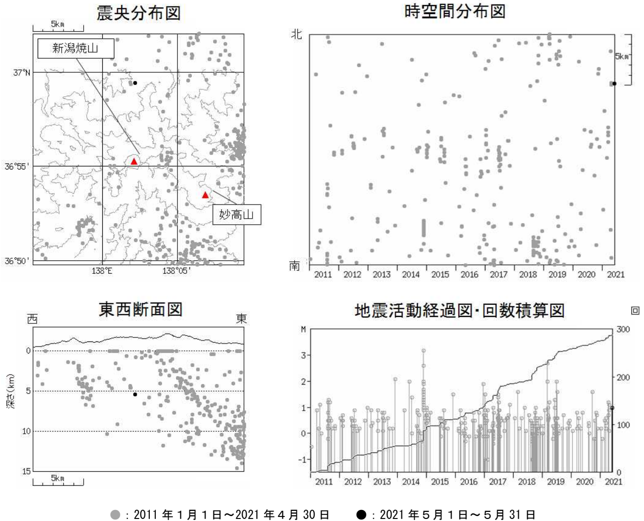
図4 新潟焼山 広域地震観測網による山体・周辺の地震活動（2011 年 1 月 1 日～2021 年 5 月 31 日）
