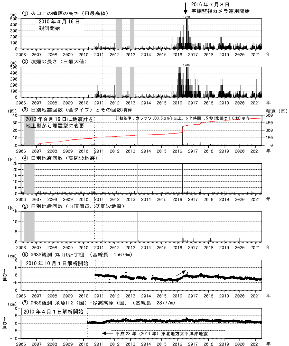
図2 新潟焼山 火山活動経過図（2006年1月1日～2021年5月31日）
