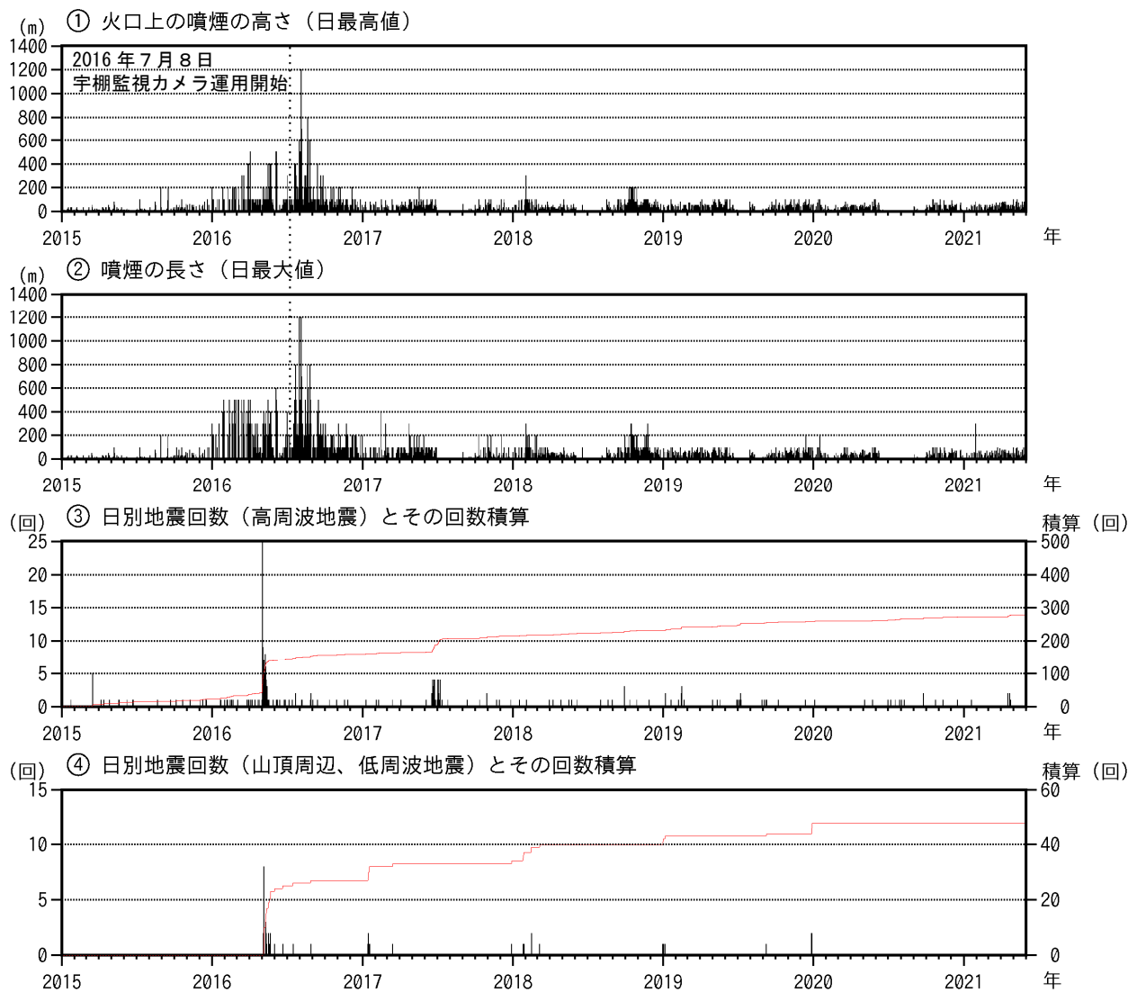
図3 新潟焼山 火山活動経過図（短期）（2015年1月1日～2021年5月31日）
