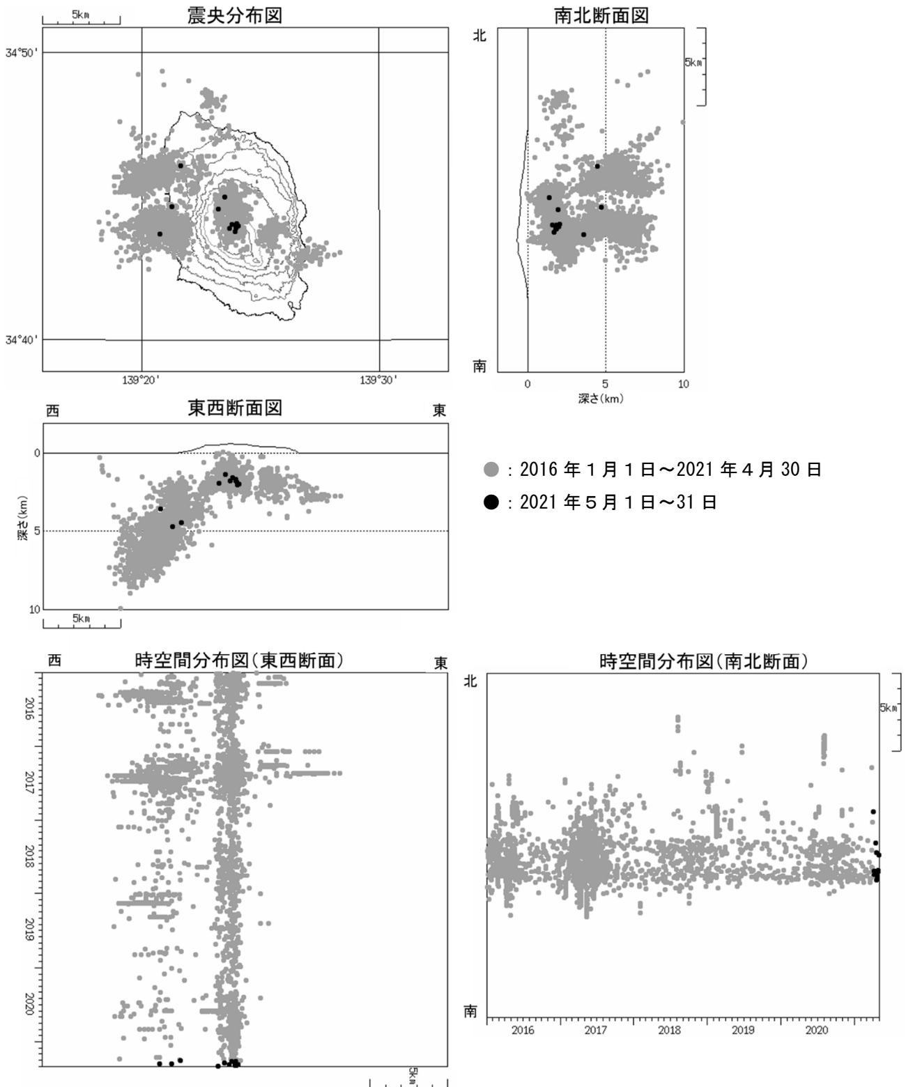
図4 伊豆大島 震源分布図（2016 年 1 月 1 日～2021 年 5 月 31 日）
