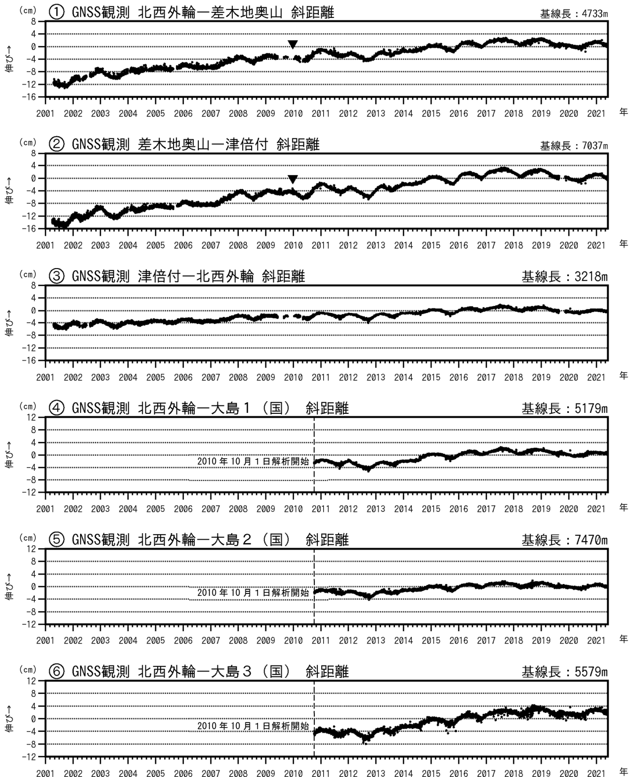
図3-1 伊豆大島 GNSS 連続観測による基線長変化(2001年1月～2021年5月31日)
