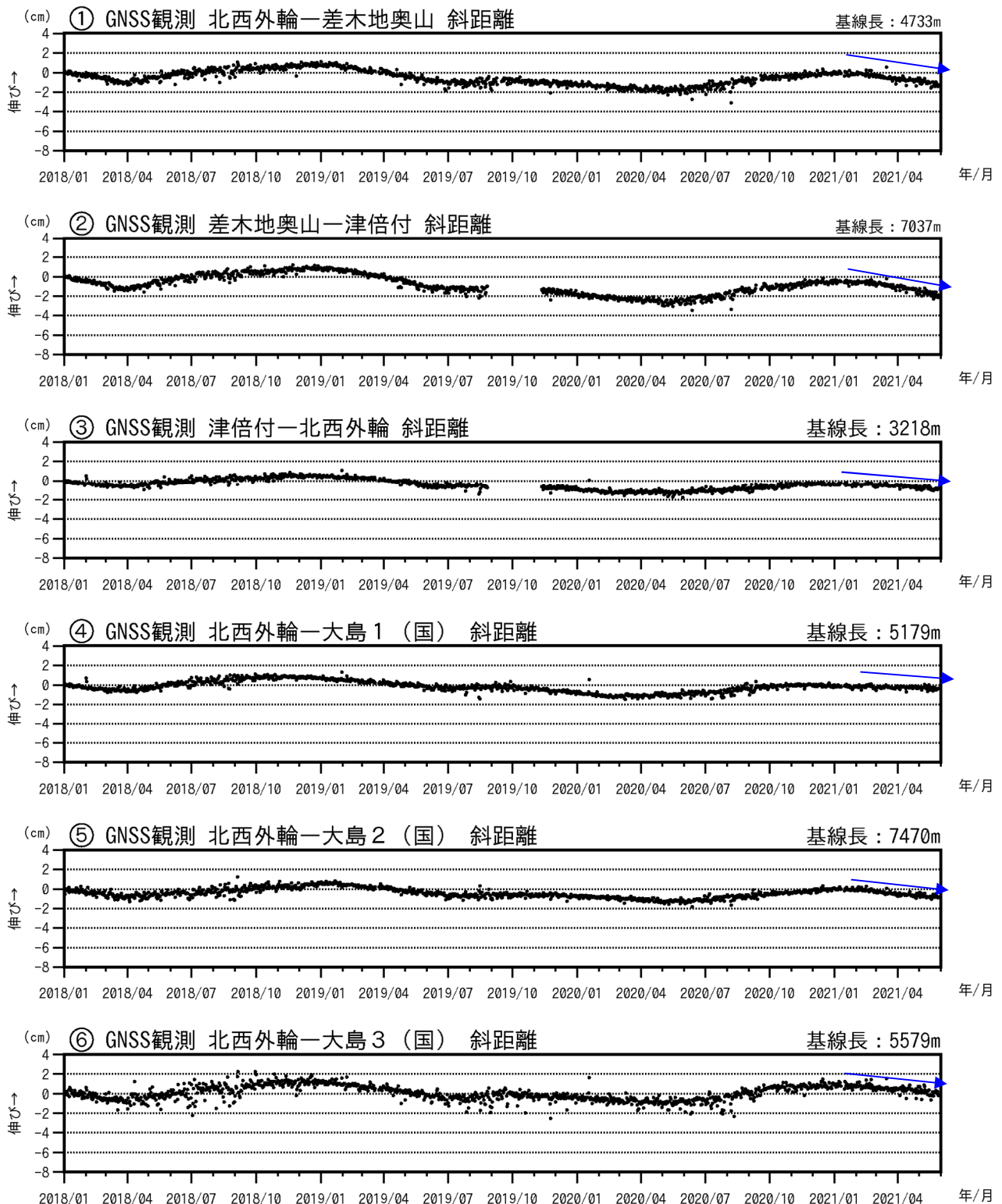
図3-2 伊豆大島 GNSS 連続観測による基線長変化(2018年1月～2021年5月31日)
