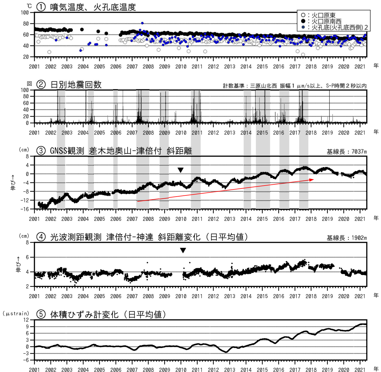
図2 伊豆大島 最近の火山活動経過図（2001年1月～2021年5月31日）
