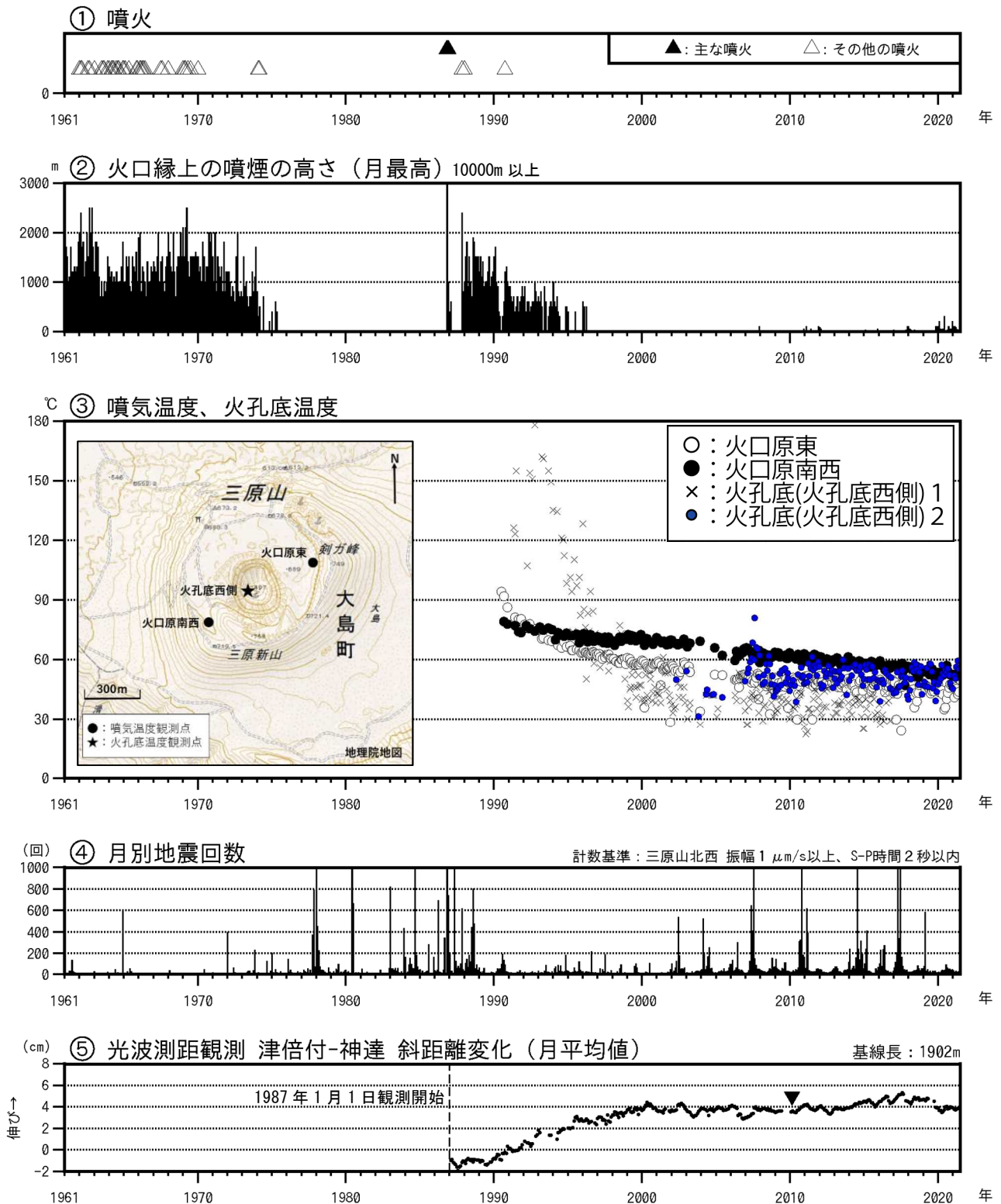
図1 伊豆大島 長期間の火山活動経過図（1961年1月～2021年6月30日）
