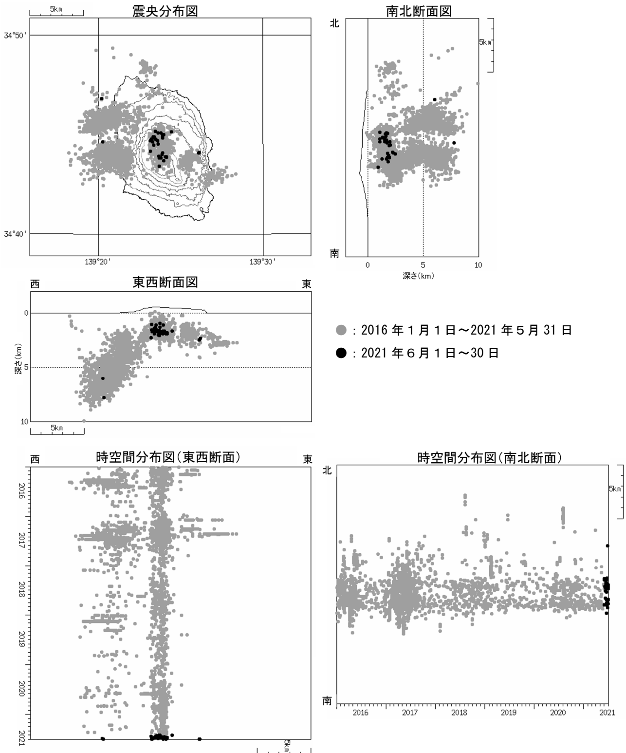
図4 伊豆大島 震源分布図（2016 年 1 月 1 日～2021 年 6 月 30 日）
