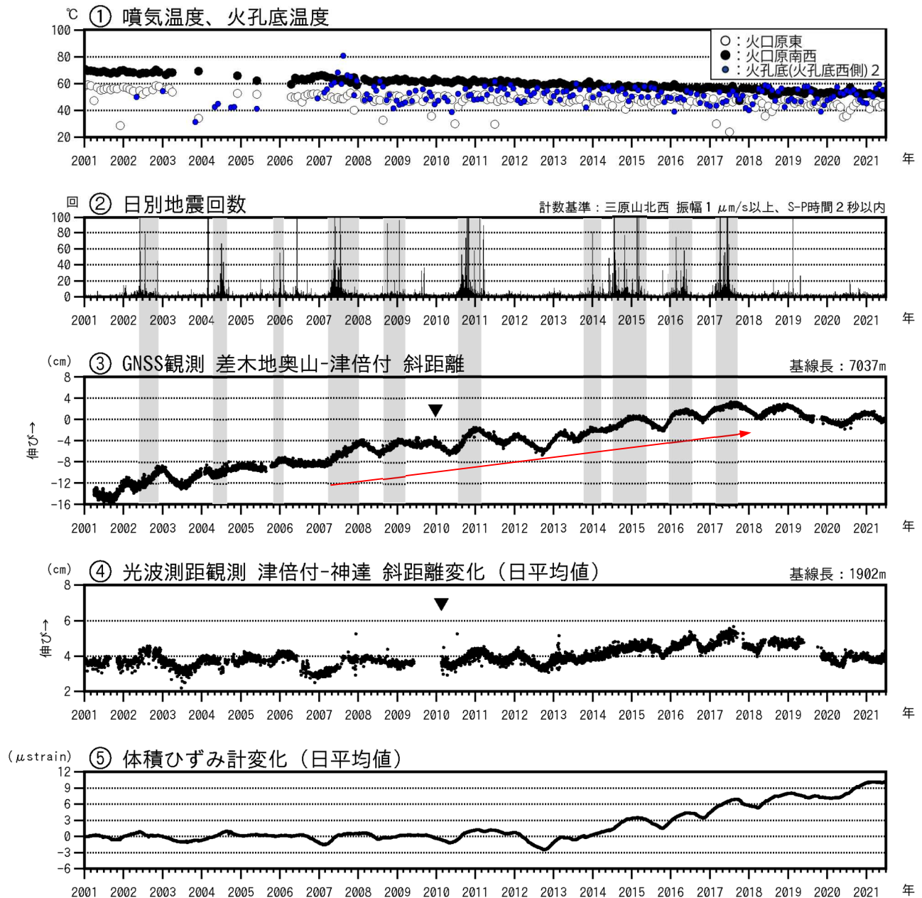
図2 伊豆大島 最近の火山活動経過図（2001年1月～2021年6月30日）
