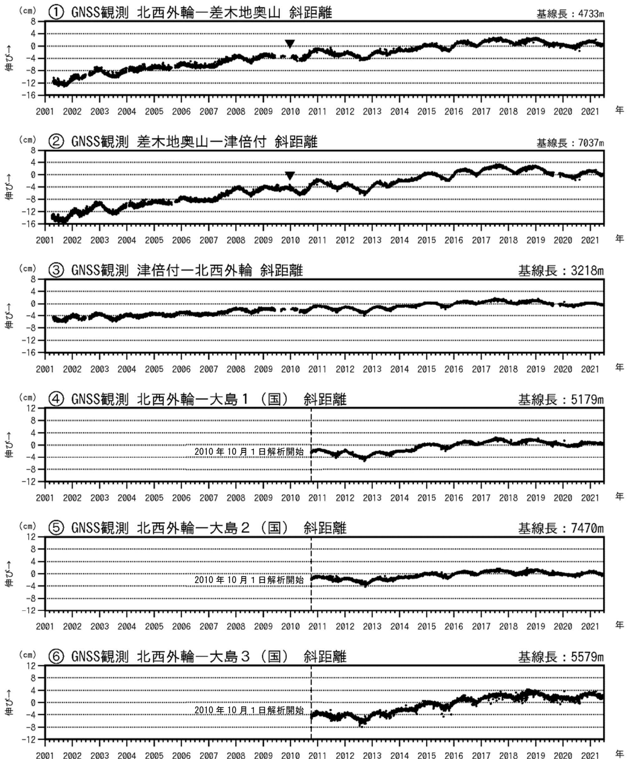
図3-1 伊豆大島 GNSS連続観測による基線長変化(2001年1月～2021年6月30日)
