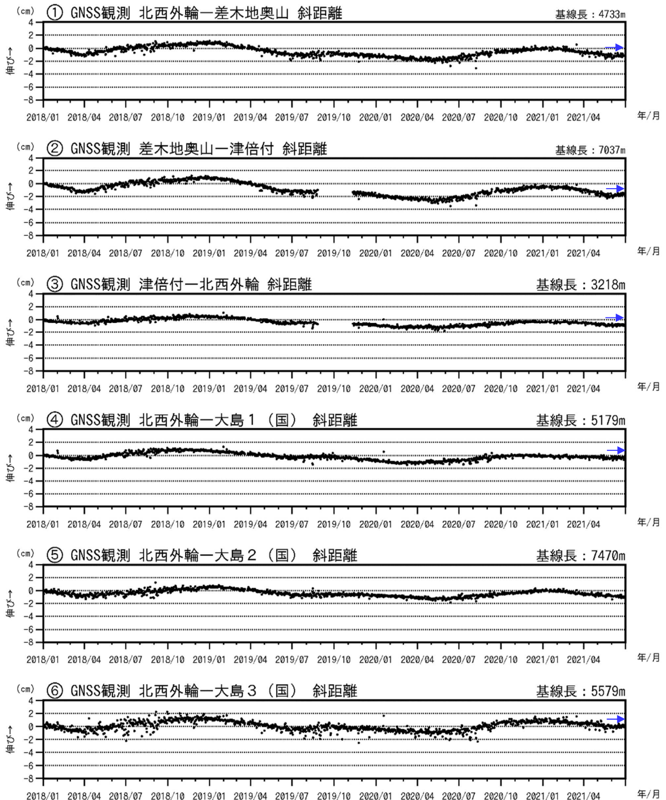
図3-2 伊豆大島 GNSS 連続観測による基線長変化(2018年1月～2021年6月30日)
