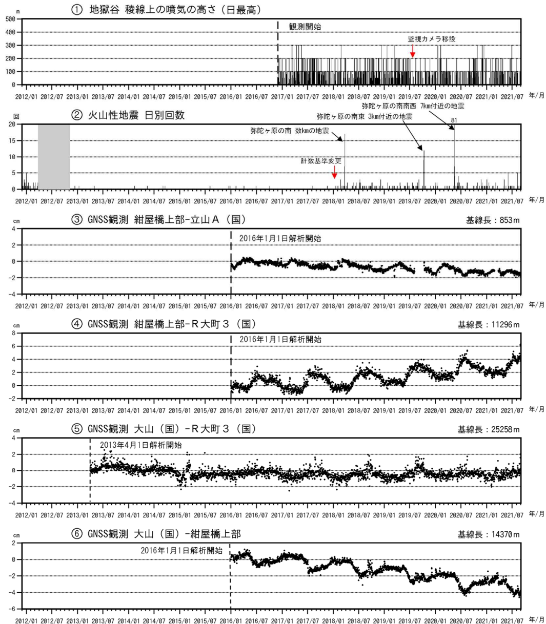
図3 弥陀ヶ原 火山活動経過図（2011年12月1日～2021年8月31日）
