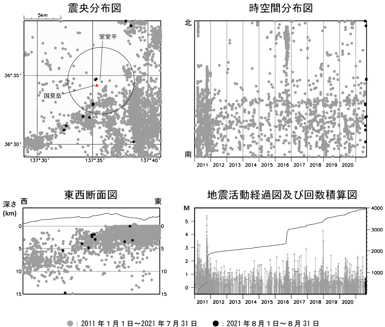
図2 弥陀ヶ原 広域地震観測網による山体・周辺の地震活動（2011 年 1 月 1 日～2021 年 8 月 31 日） 震央分布図中の円は弥陀ヶ原の計数対象地震（室堂平で S-P 時間 1 秒以内）のおよその範囲を示しています。 広域地震観測網により震源決定したもので、深さは全て海面以下として決定しています。 図中の震源要素は一部暫定値が含まれており、後日変更することがあります。 この図では、関係機関の地震波形を一元的に処理し、地震観測点の標高を考慮する等した新手法で得られた震源を用いています（ただし、2020 年 8 月以前の地震については火山活動評価のための参考震源です）。 2021 年 9 月 8 日現在、次の期間の地震について、暫定的に震源精査の基準を変更しているため、その前後の期間と比較して微小な地震での震源決定数の変化（増減）が見られます。 (1) 2020 年 4 月 18 日から 10 月 23 日まで、(2) 2021 年 1 月 9 日から 3 月 7 日まで、(3) 2021 年 4 月 19 日以降
