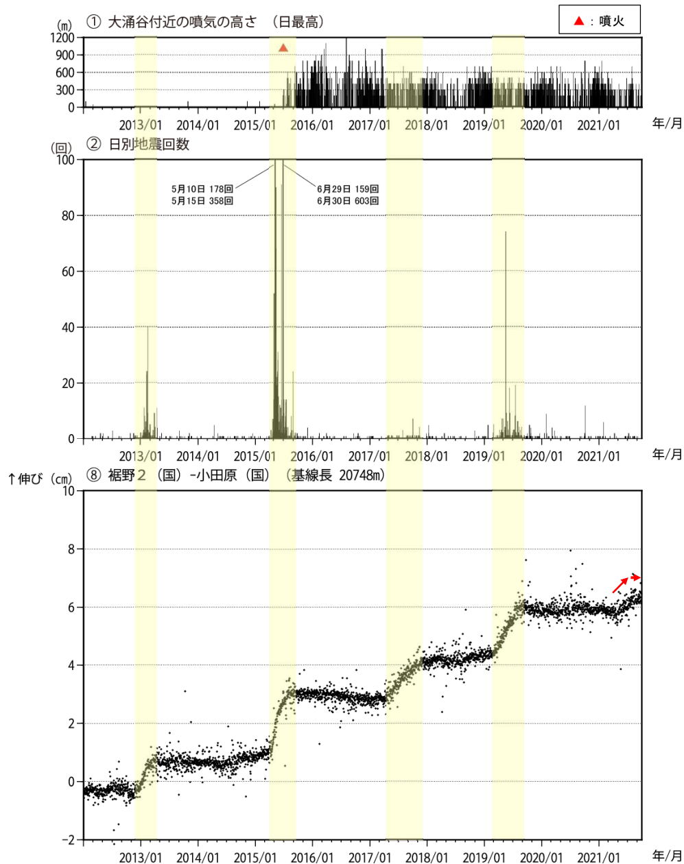
図5-1 箱根山 火山活動経過図（2012年1月1日～2021年9月30日）
