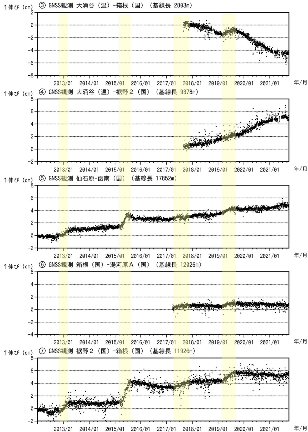
図5-2 箱根山 GNSS連続観測による基線長変化（2012年1月1日～2021年9月30日）
