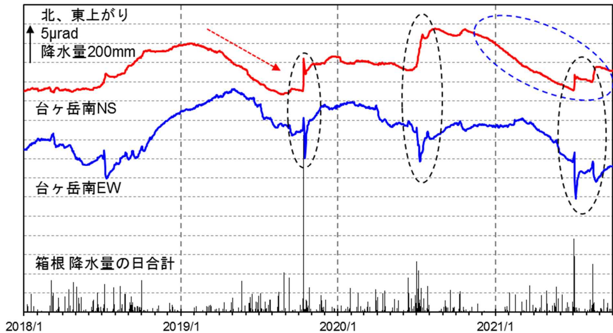
図7 箱根山 台ヶ岳南観測点における傾斜データ（2018年1月1日～2021年9月30日）
