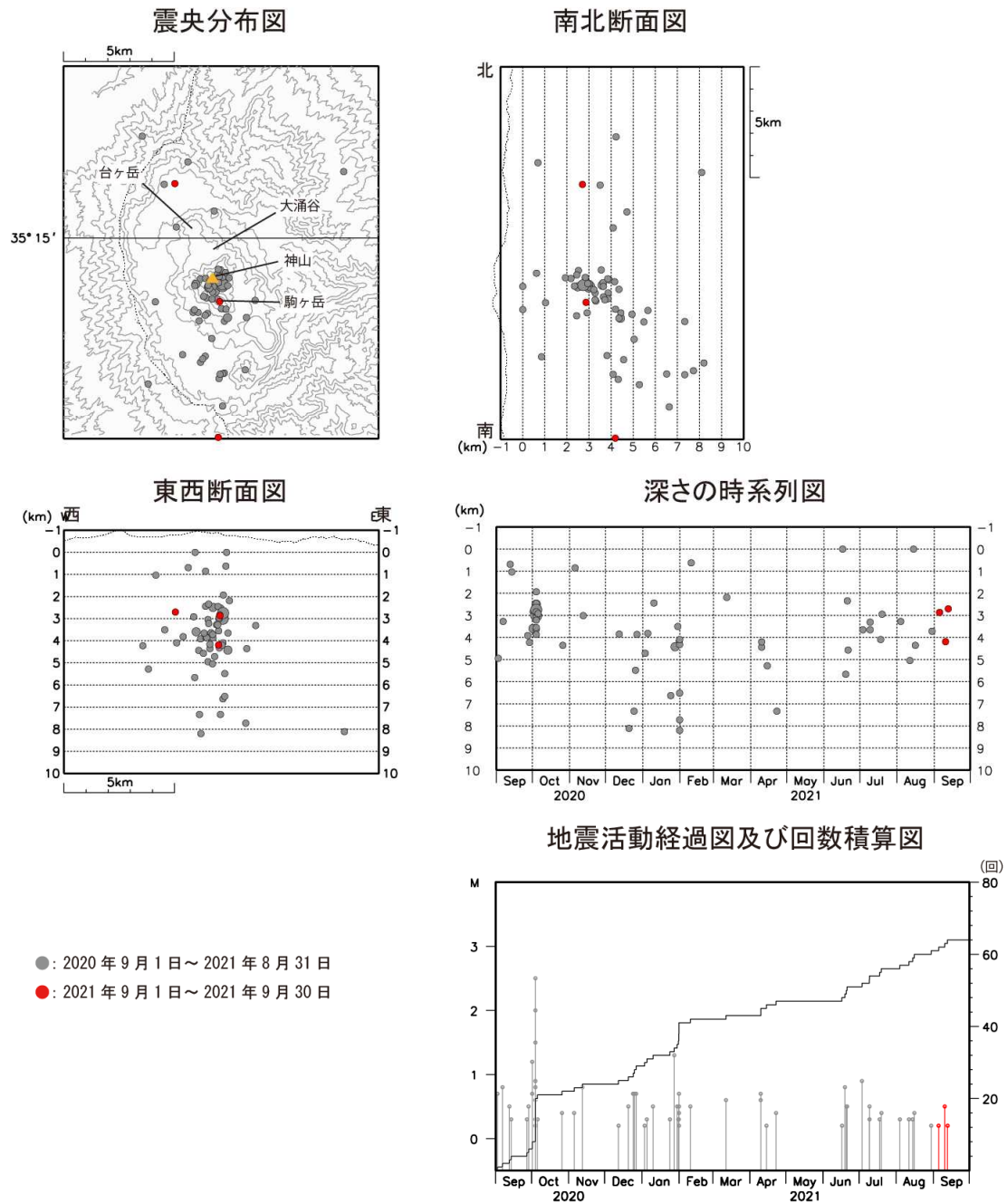
図6 箱根山 広域地震観測網による山体周辺の震源分布図（2020年9月1日～2021年9月30日）
