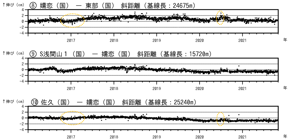
図6-2 浅間山 GNSS 連続観測結果(2016年1月1日~2021年10月31日)
