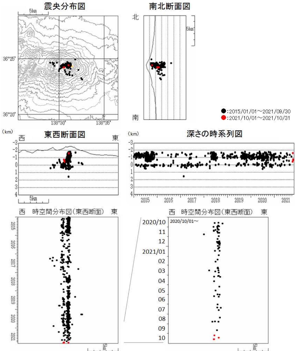
図5 浅間山 震源分布図（2015年1月1日～2021年10月31日） ・火山性地震の震源は、従来からみられている山頂直下の海拔0～2km付近に分布しています。
