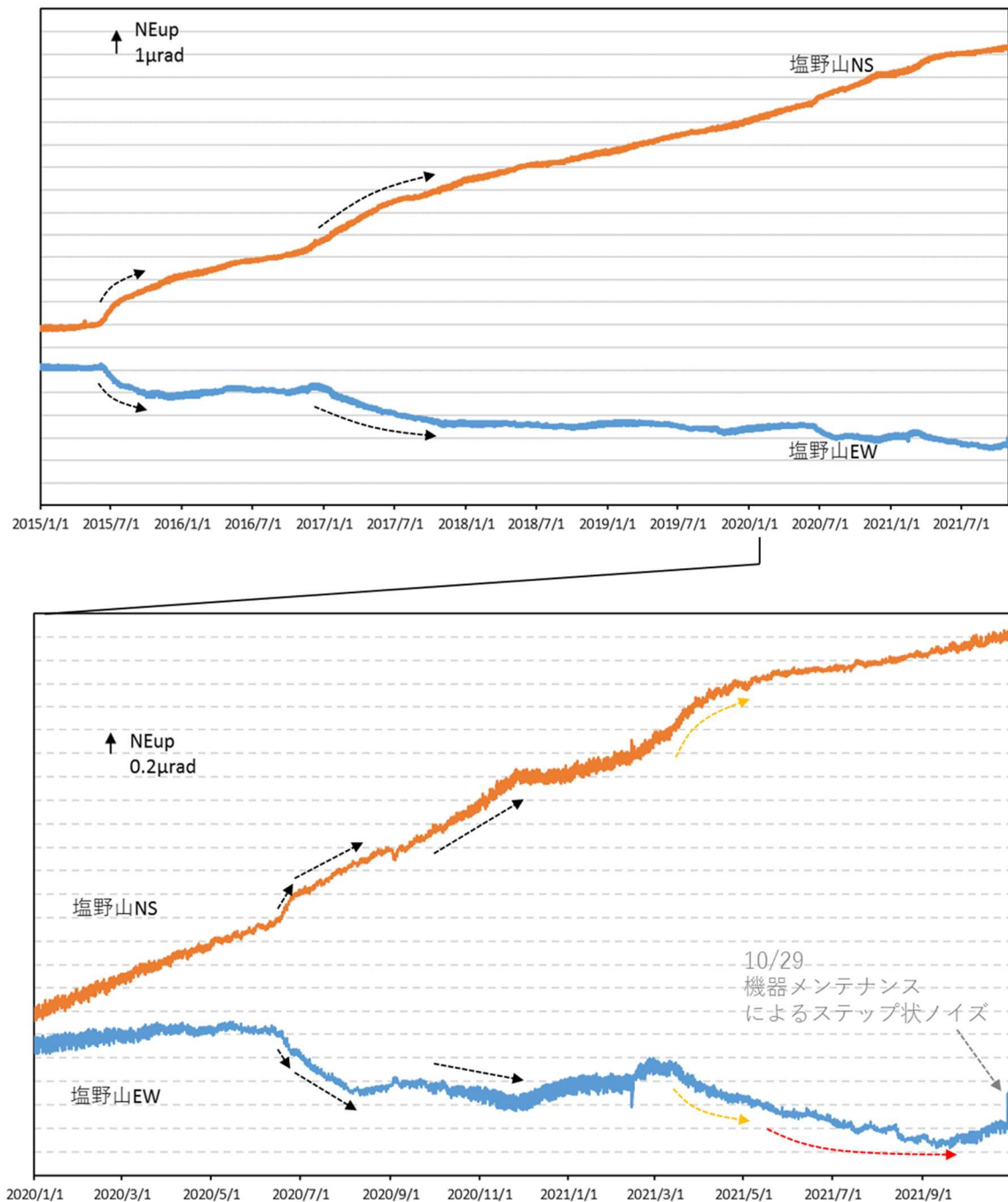
図8 浅間山 塩野山観測点における傾斜データ（2015年1月1日～2021年10月31日） データは時間平均値を使用しており、長期にわたるトレンドを補正しています。 下段は上段に比べて縦軸を拡大しています。
