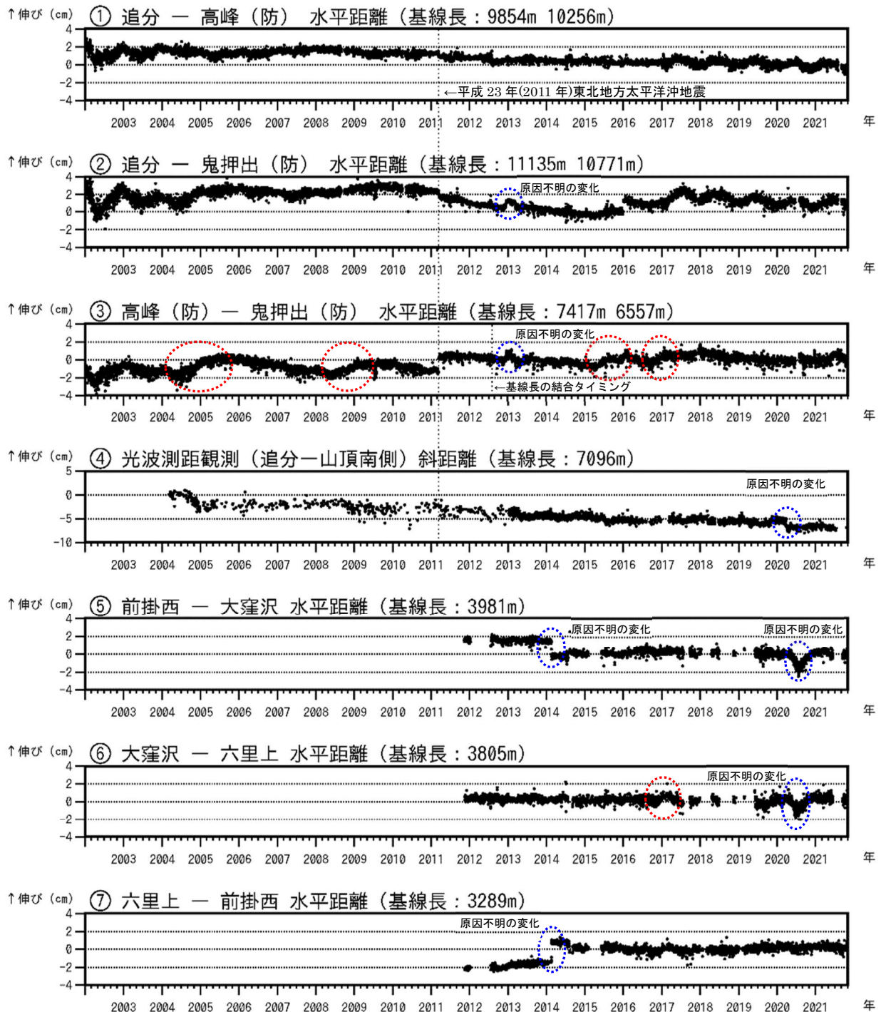
図6-1 浅間山 GNSS連続観測及び光波測距観測の結果(2002年1月1日～2021年10月31日) 2010年10月及び2016年1月に、解析方法を変更しています。
