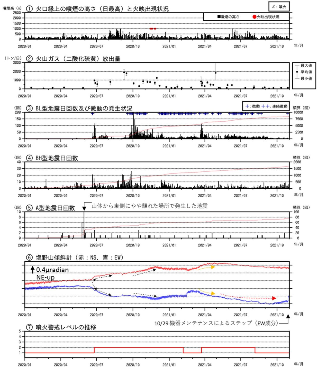
図3 浅間山 火山活動経過図（2020年1月1日～2021年10月31日）
