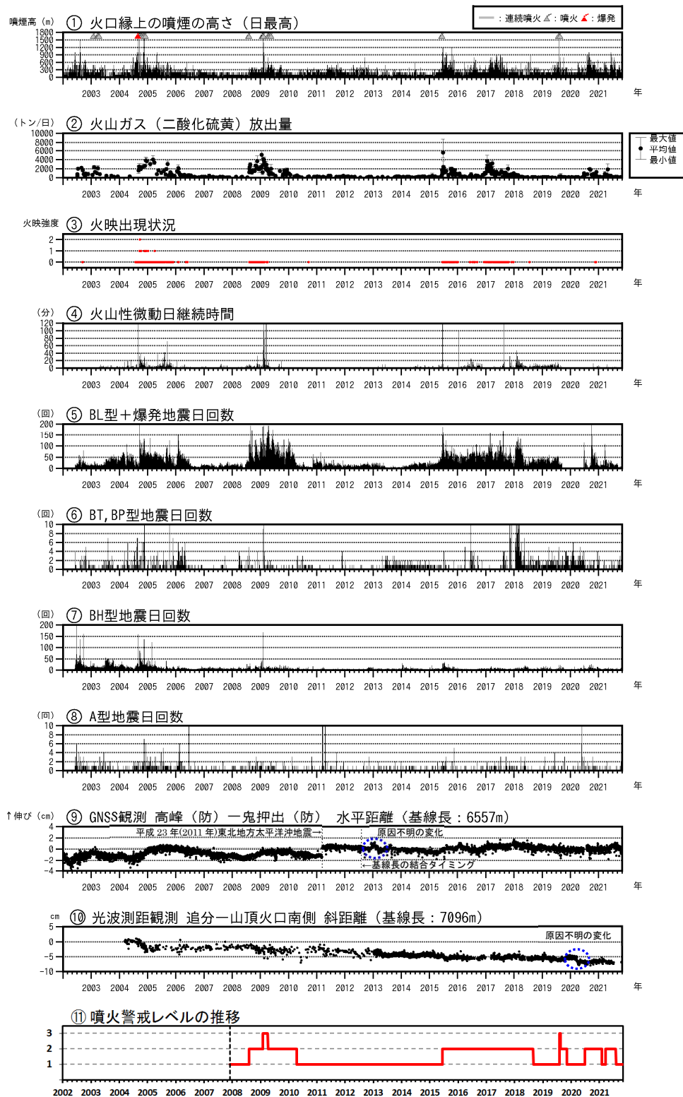
図4 浅間山 火山活動経過図（2002年1月1日～2021年10月31日）
