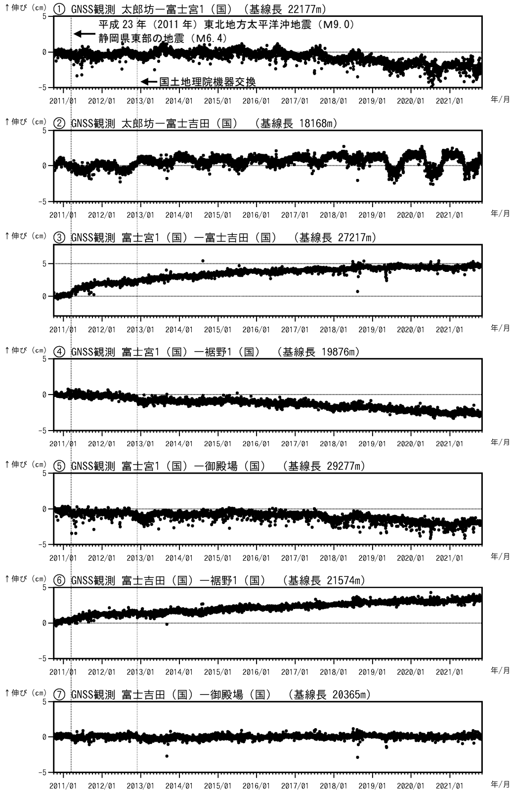
図4 富士山 GNSS 連続観測による基線長変化 (2010 年 10 月 1 日～2021 年 10 月 31 日)
