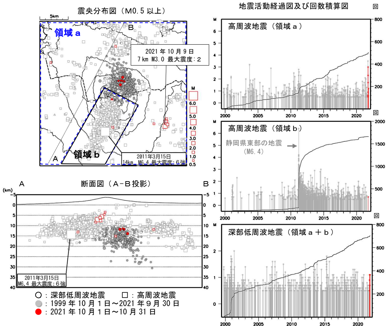
図3 富士山 広域地震観測網による山体及び周辺の地震活動(1999年10月1日～2021年10月31日)
