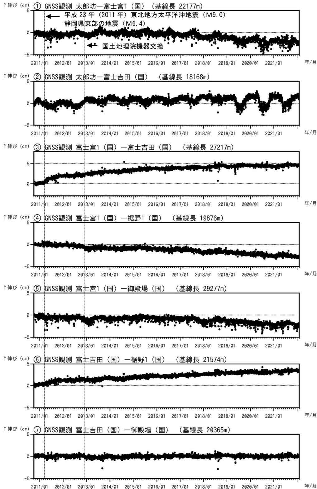
図4 富士山 GNSS 連続観測による基線長変化 (2010 年 10 月 1 日～2022 年 1 月 31 日) (国): 国土地理院 「平成 23 年 (2011 年) 東北地方太平洋沖地震」及び 2011 年 3 月 15 日に発生した静岡県東部の地震 (M 6.4) によるステップ状の変化を補正しています。 ①～⑦は図5の GNSS 基線①～⑦に対応しています。
