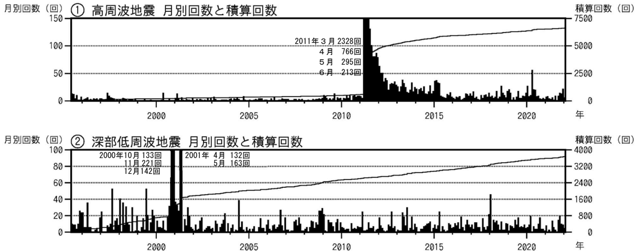
図2 富士山 月別地震回数（1995年6月1日～2022年1月31日）
