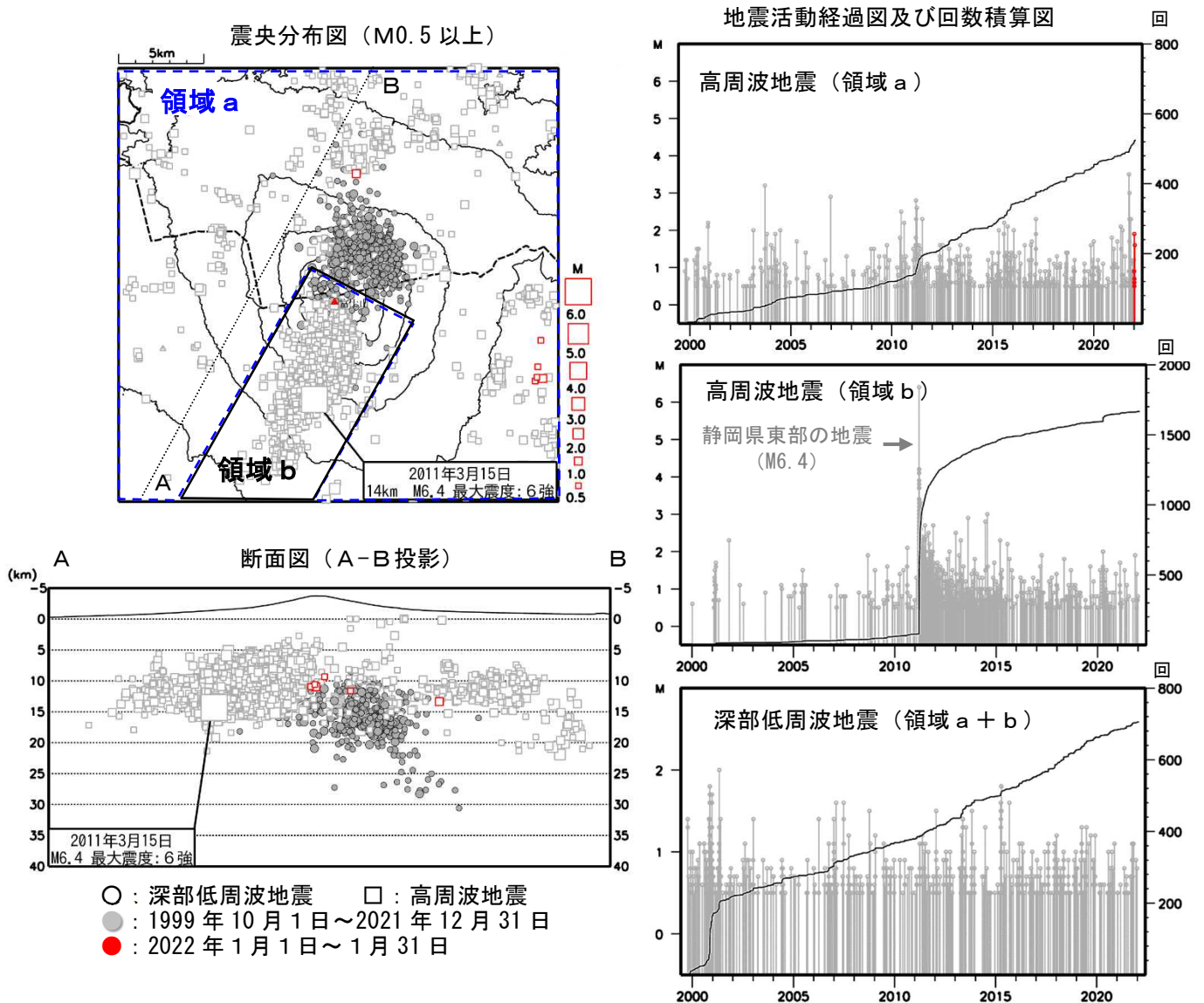
図3 富士山 広域地震観測網による山体及び周辺の地震活動（1999年10月1日～2022年1月31日）
