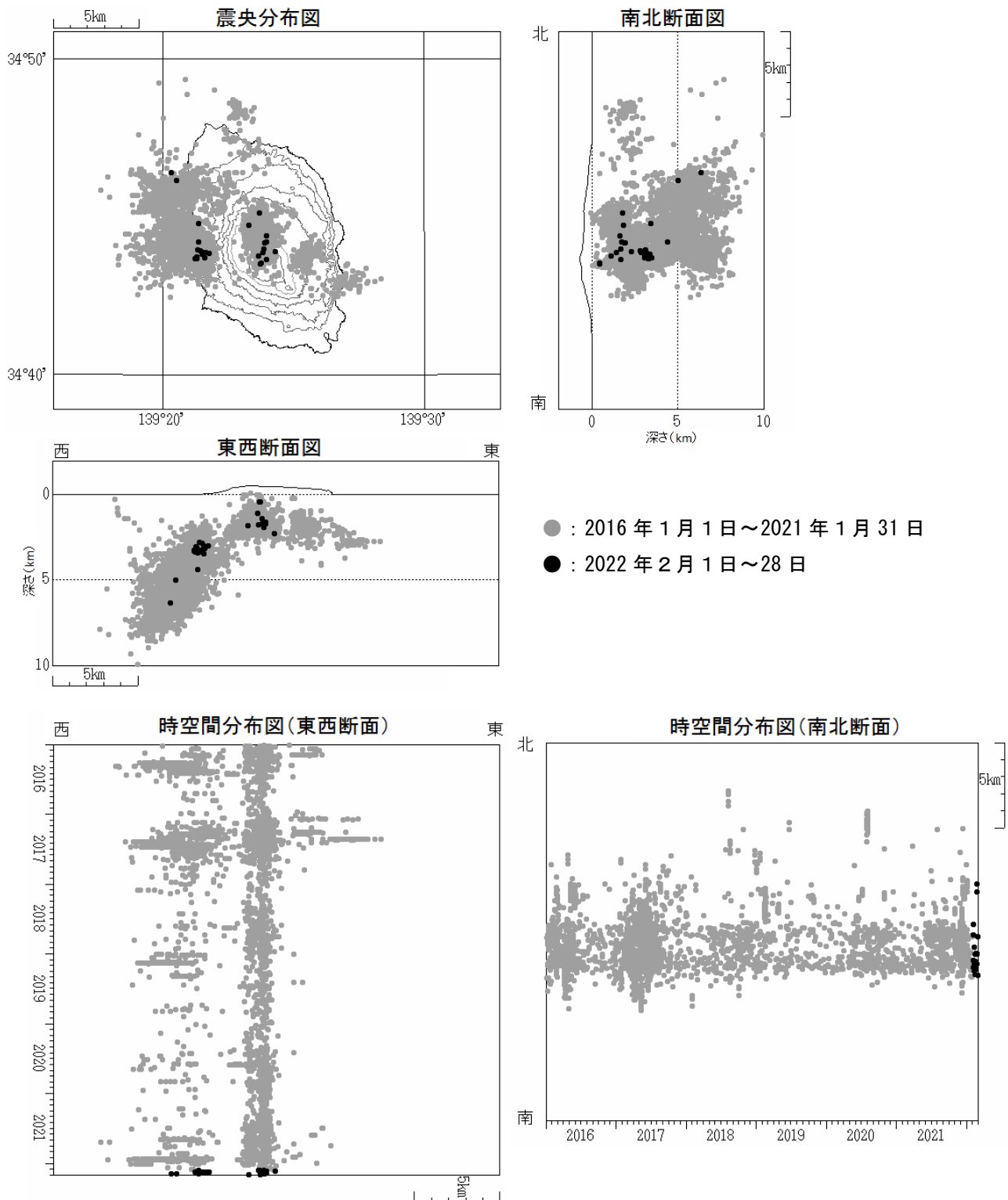
図4 伊豆大島 震源分布図（2016 年 1 月 1 日～2022 年 2 月 28 日）
