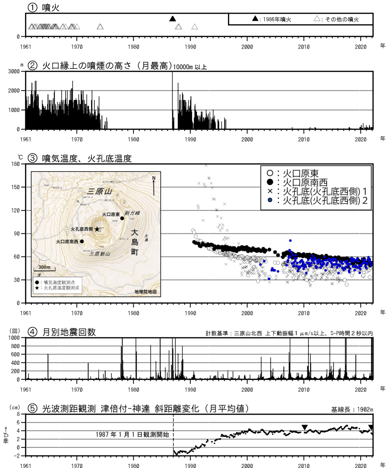
図1 伊豆大島 長期間の火山活動経過図（1961年1月～2022年2月28日）
