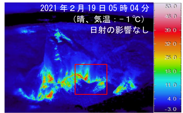
図6 伊豆大島 中央火口内の状況（撮影方向は図8参照）
