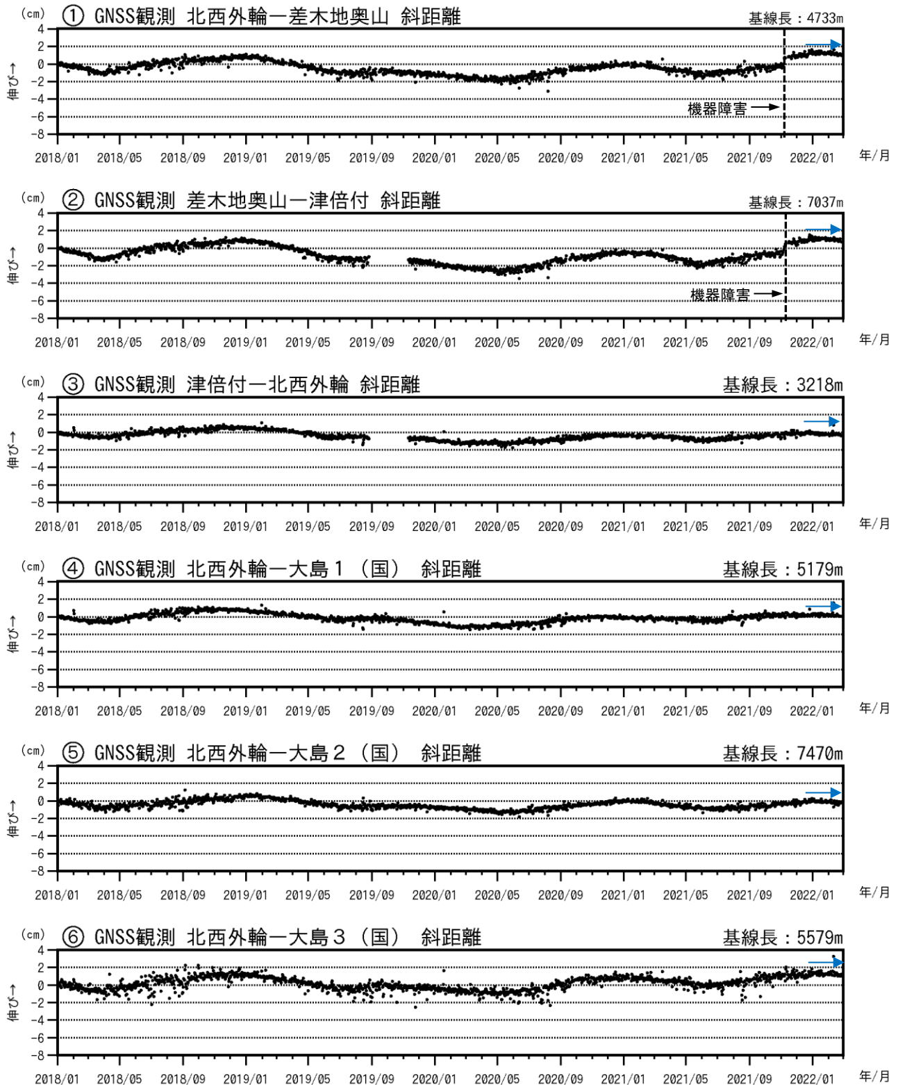
図3-2 伊豆大島 GNSS連続観測による基線長変化(2018年1月～2022年2月28日)
