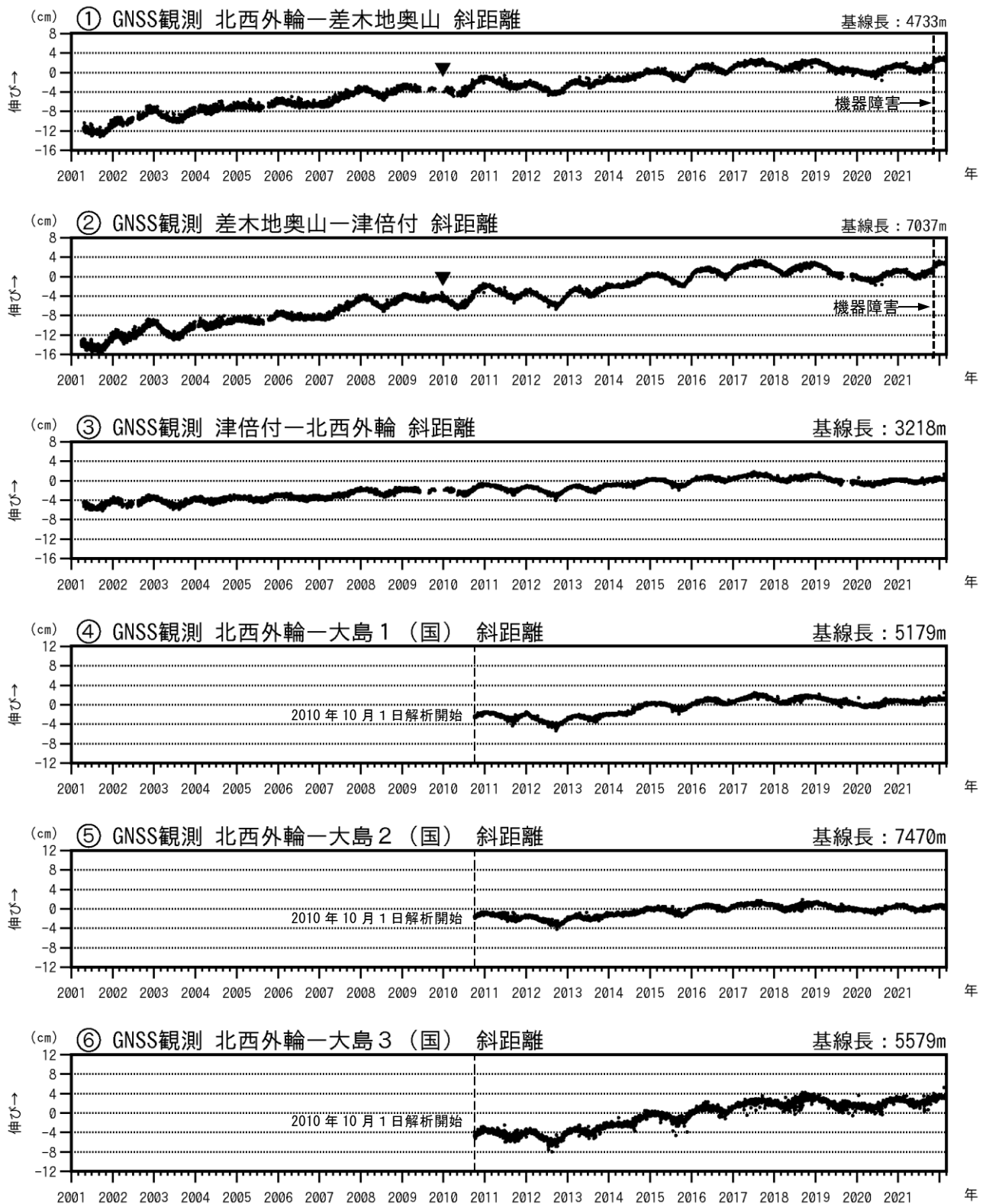
図3-1 伊豆大島 GNSS 連続観測による基線長変化(2001年1月～2022年2月28日)
