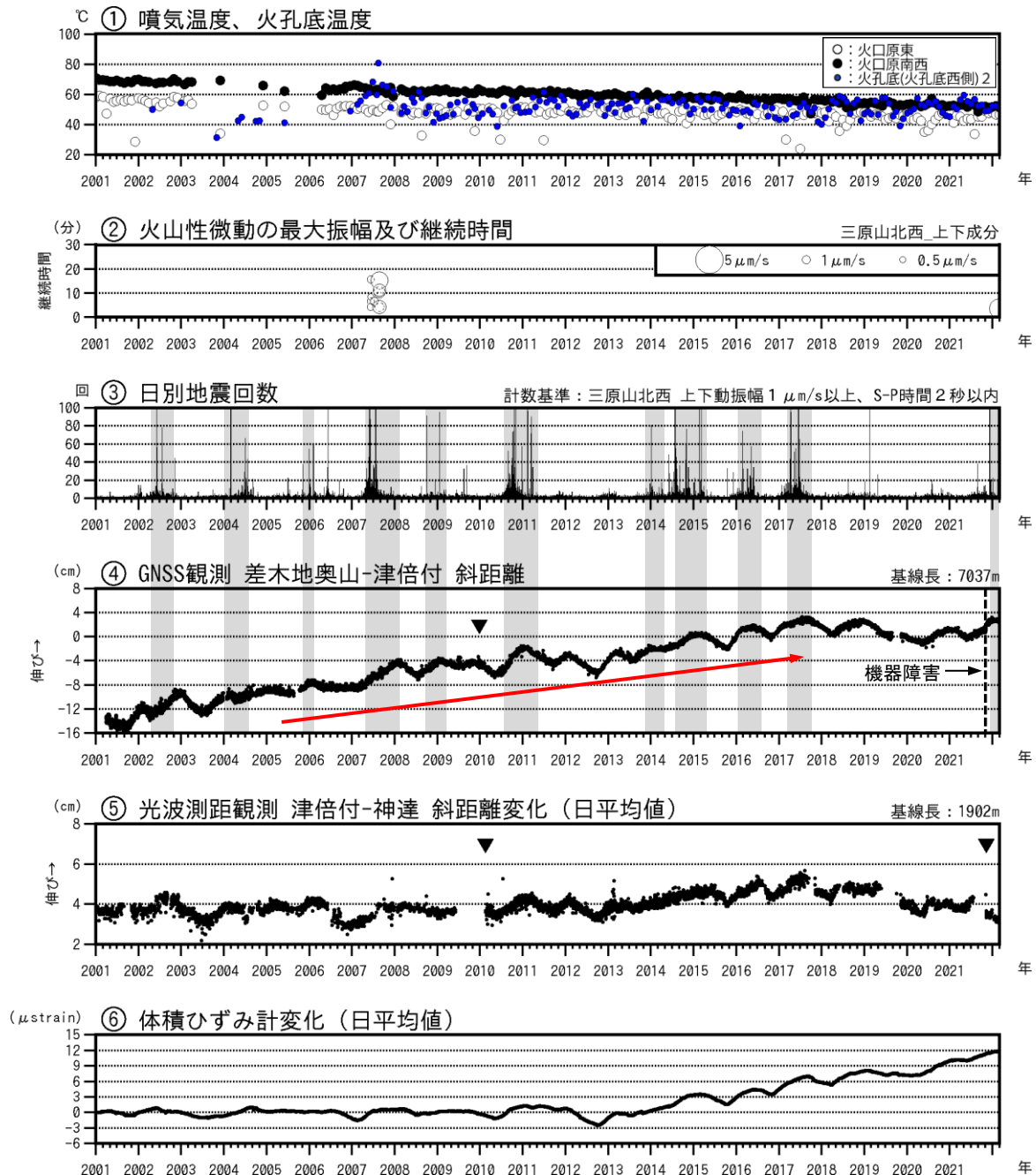
図2 伊豆大島 最近の火山活動経過図（2001年1月～2022年2月28日）
