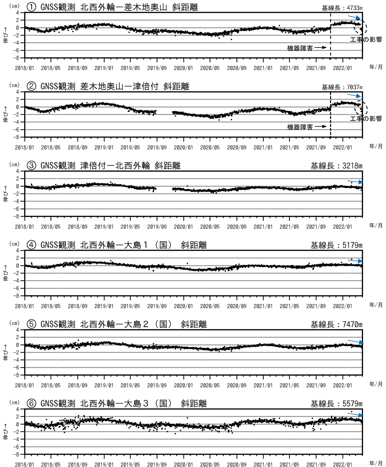
図3-2 伊豆大島 GNSS連続観測による基線長変化(2018年1月～2022年3月31日)
