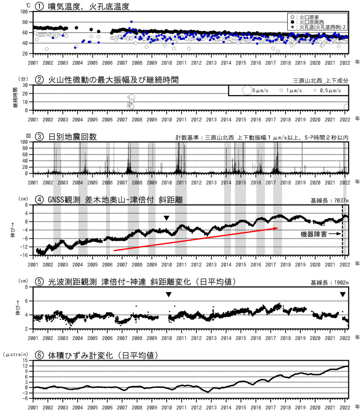
図2 伊豆大島 最近の火山活動経過図（2001年1月～2022年3月31日）
