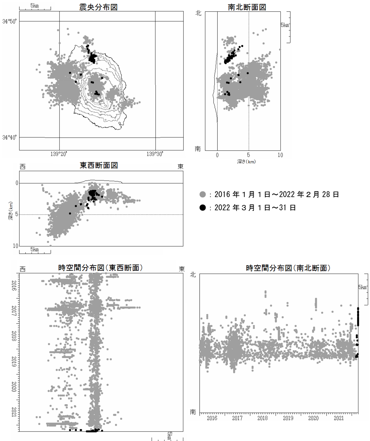
図4 伊豆大島 震源分布図（2016 年 1 月 1 日～2022 年 3 月 31 日）
