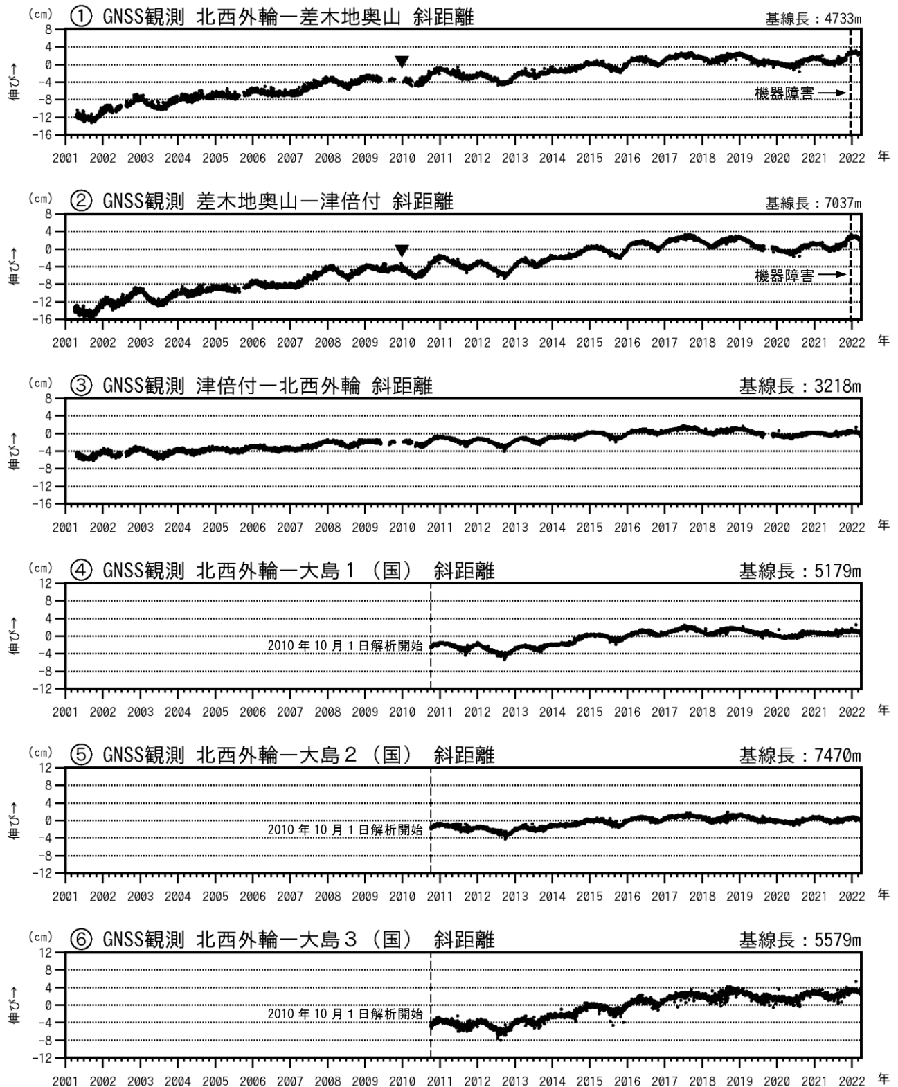
図3-1 伊豆大島 GNSS 連続観測による基線長変化(2001年1月～2022年3月31日)
