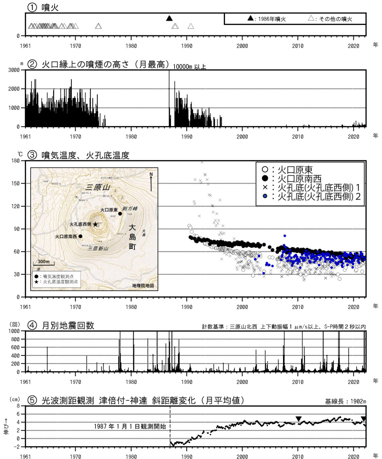
図1 伊豆大島 長期間の火山活動経過図（1961年1月～2022年3月31日）
